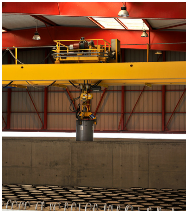
Stockage de colis de déchets dans un ouvrage du Centre de stockage de l'Aube (CSA)
