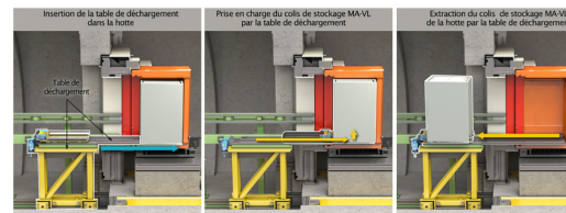
Double porte étanche entre la hotte de transfert et l'alvéole de stockage
