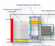
Portique mobile pour constituer une pile de deux colis
