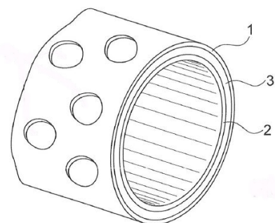
Schéma de principe de la technologie avec le chemisage externe perforé (1), le chemisage interne (2) et le matériau de remplissage entre les deux structure (3).
