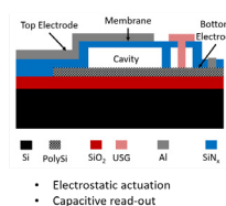
Présentation du dispositif de détection par ultrason
