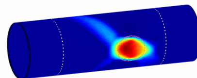
Simulation de la propagation d'ondes guidées dans un cylindre en acier
