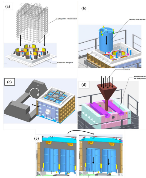
Étapes de fabrication d'un conteneur de stockage de déchets radioactifs en béton moulé.
