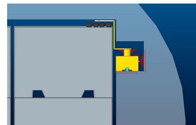
Image 3D du bras Cléopatra dans un alvéole de colis de stockage MA-VL.
