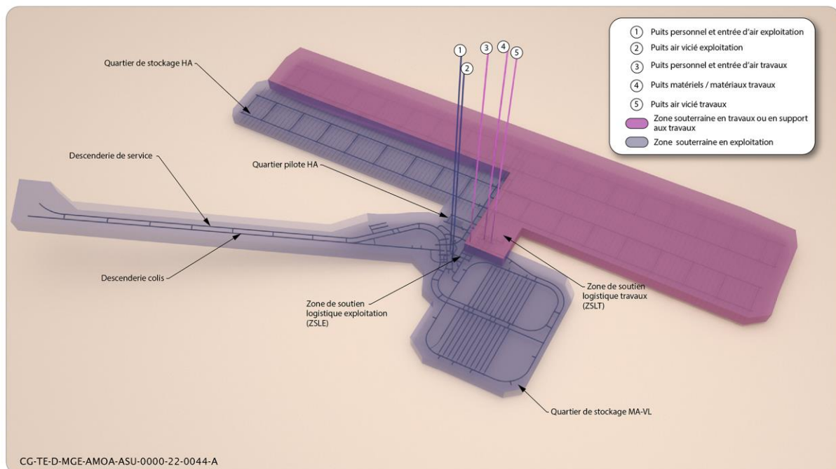
Figure 5-8 Illustration du principe de séparation de la zone souterraine exploitée pour le stockage (en gris) et de la zone souterraine en travaux ou en support aux travaux (en magenta)
