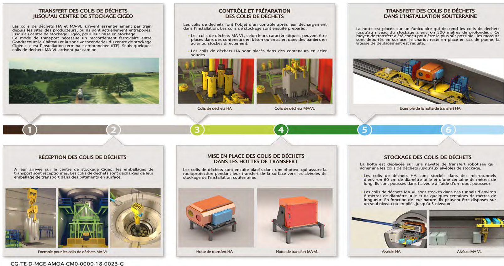
Figure 2-11 Grands principes de cheminement des colis de déchets HA et MA-VL jusqu'à leur emplacement de stockage
