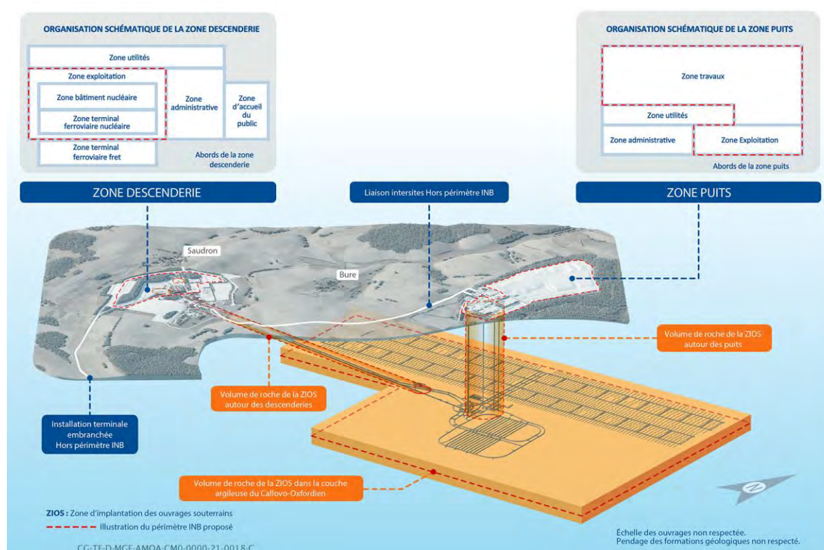
Figure 2-6 Représentation schématique de l'INB
