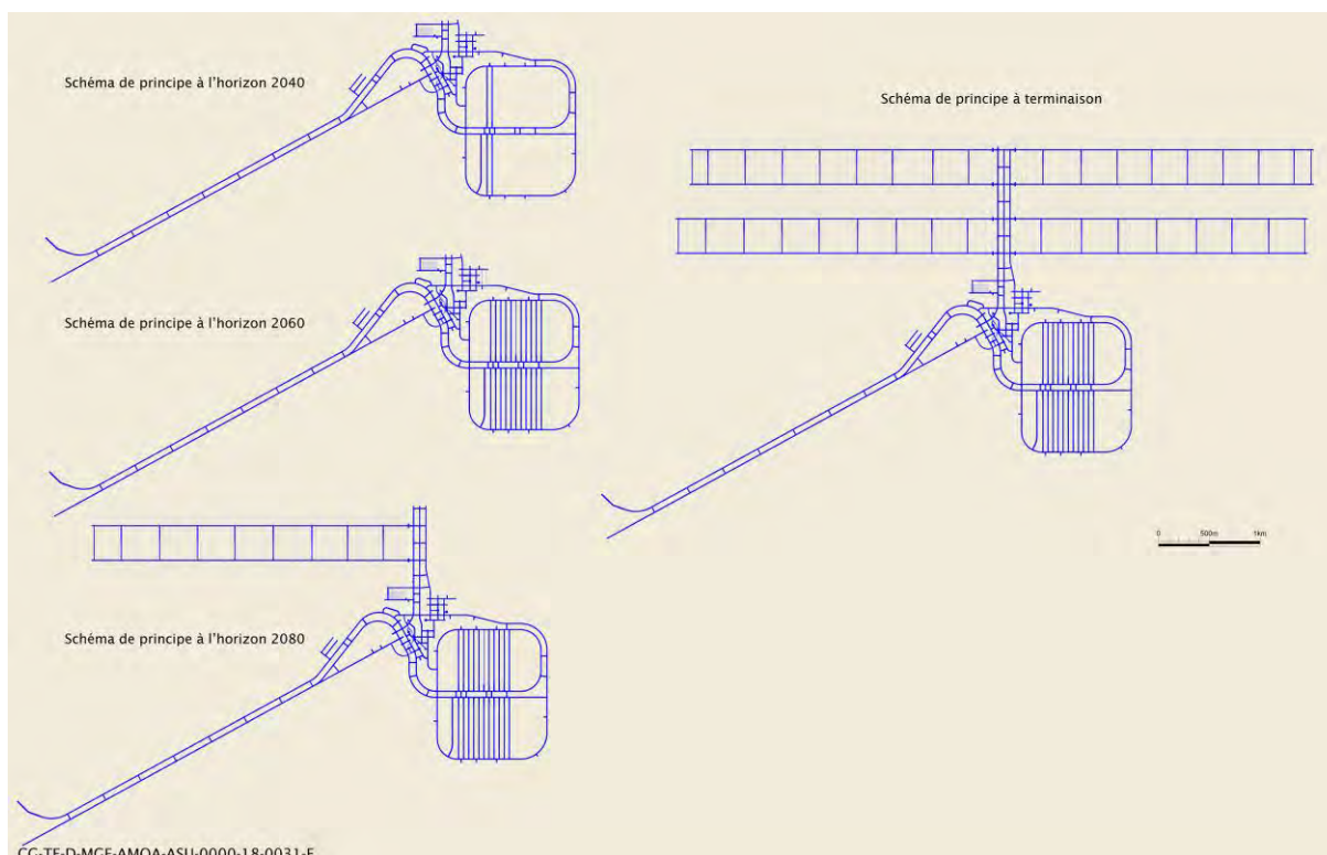
Figure 2-14 Schéma illustratif du développement progressif des ouvrages souterrains de l'INB Cigéo
