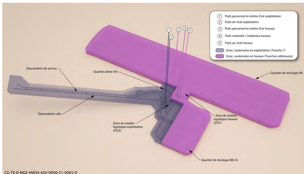
Figure 2-10 Illustration de principe de séparation des zones souterraines en exploitation et en travaux et liaisons surface-fond associées (dimensions et proportions non représentatives)
