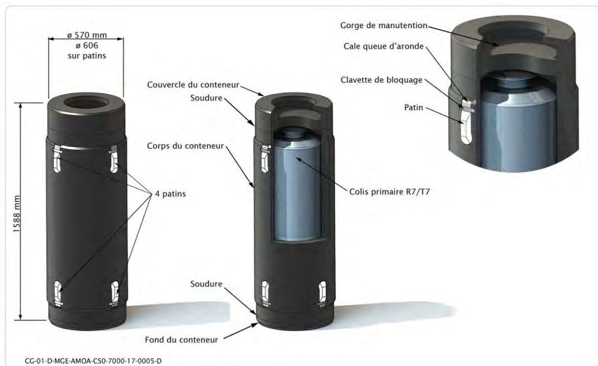
Figure 3-4 Illustration d'un colis de stockage de déchets vitrifiés HA avec son conteneur de stockage
