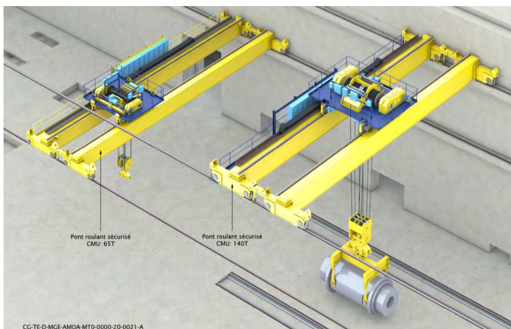
Figure 5-11 Illustration des ponts roulants sécurisés
