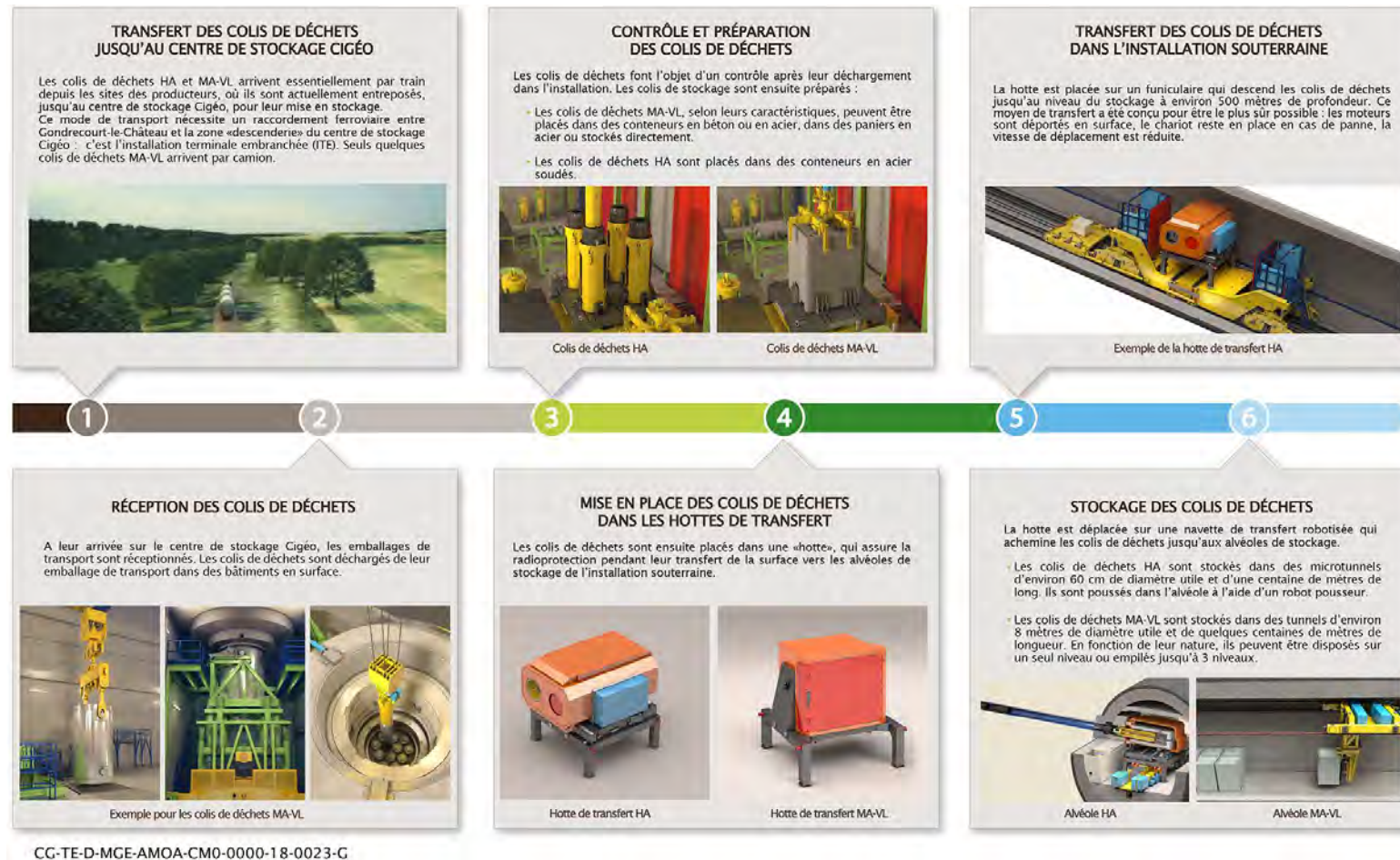
Figure 7-10 Cheminement des colis de déchets de leur arrivée à Cigéo jusqu'à leur emplacement de stockage
