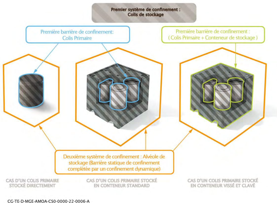
Figure 5-7 Illustration des systèmes de confinement des colis de déchets MA-VL stockés en alvéoles de stockage en fonction du mode de stockage retenu
