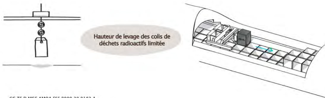
Figure 7-21 Illustration de la manutention des colis de stockage MA-VL à faible hauteur
