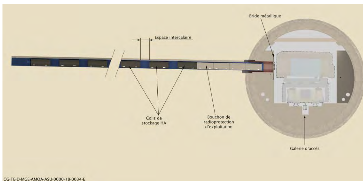
Figure 2-12 Coupe longitudinale schématique d'un alvéole HA
