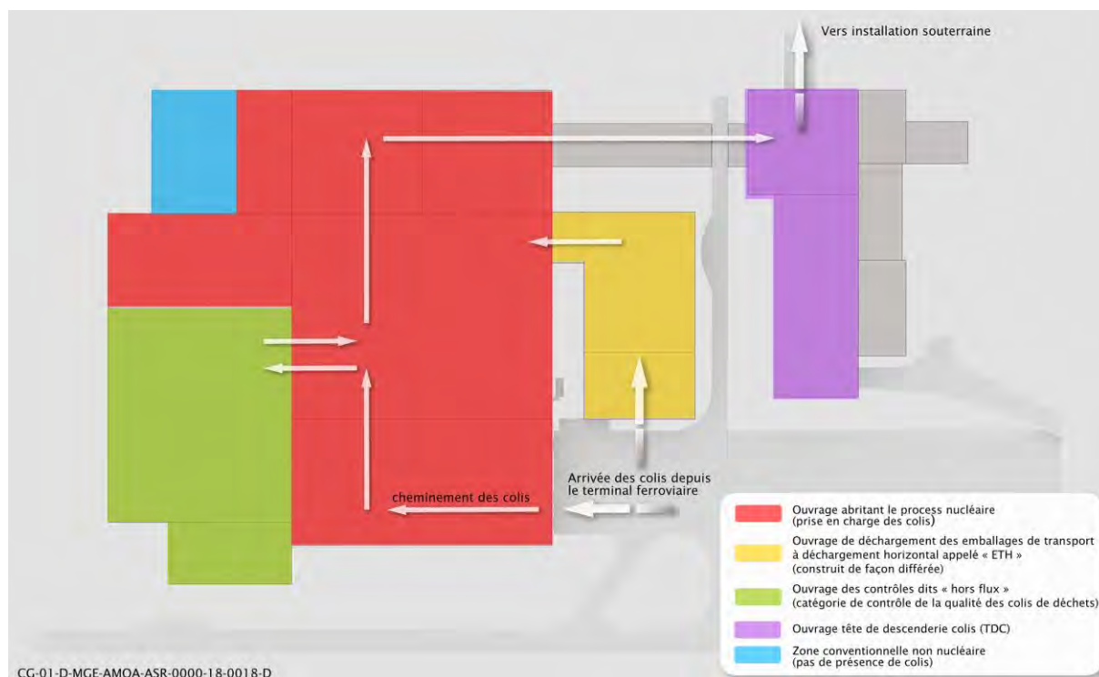
Figure 2-8 Illustration du principe d'organisation du Bâtiment EP1 et de la tête de descente
