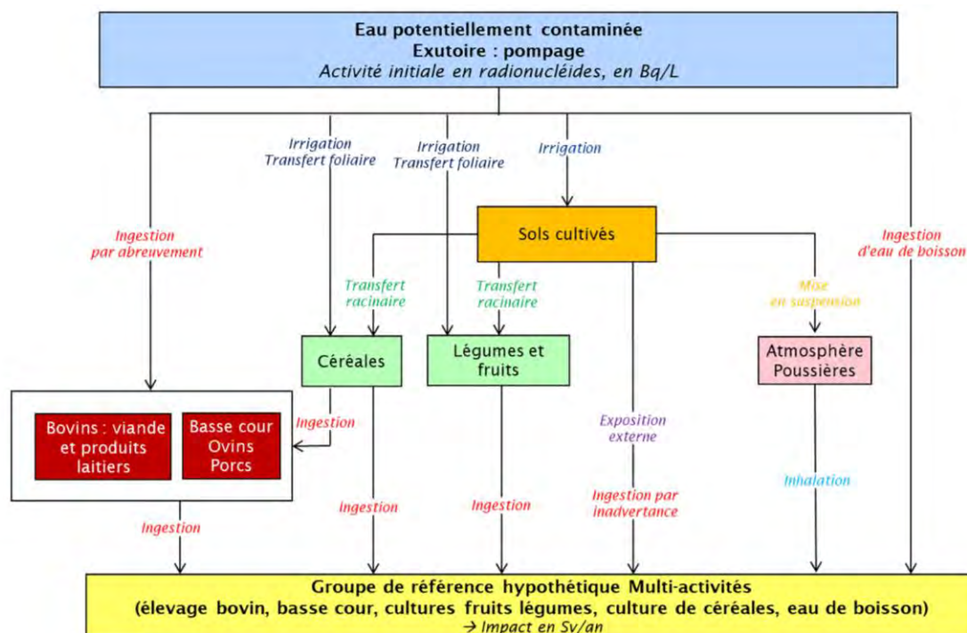
Figure 4-6 Schéma illustratif des voies de contamination d'un individu utilisant de l'eau potentiellement contaminée par des radionucléides extraite par pompage à un exutoire
