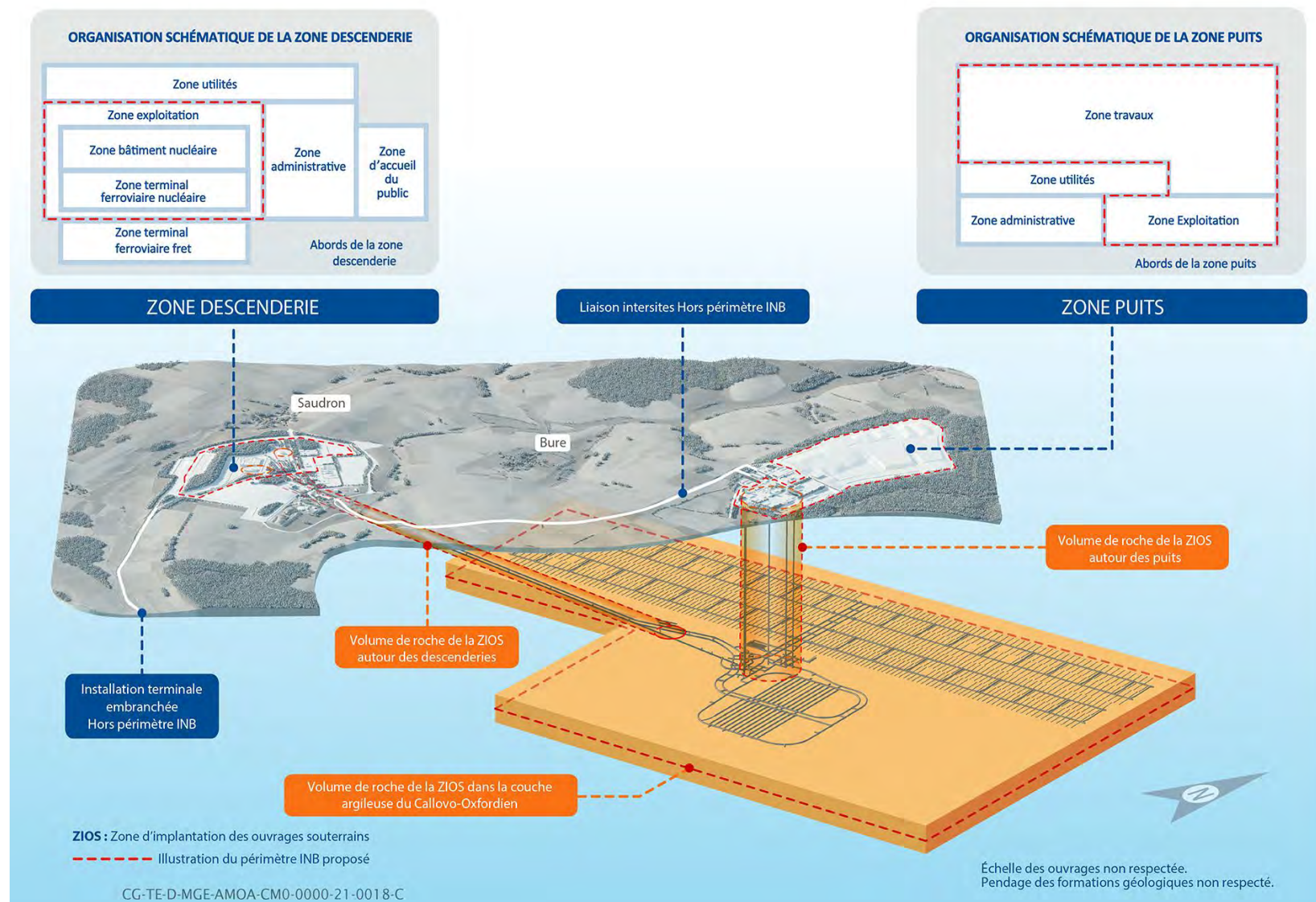
Figure 7-9 Représentation schématique du périmètre INB de Cigéo
