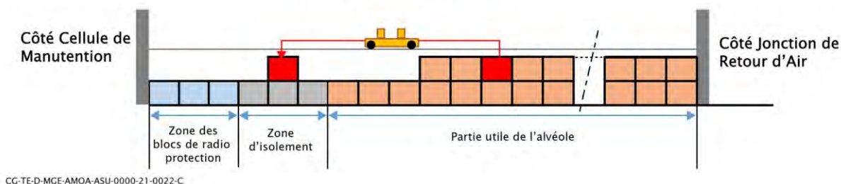
Figure 6-3 Schéma de principe de l'alvéole de stockage renforcée pour le stockage de colis de déchets bitumés en l'état
