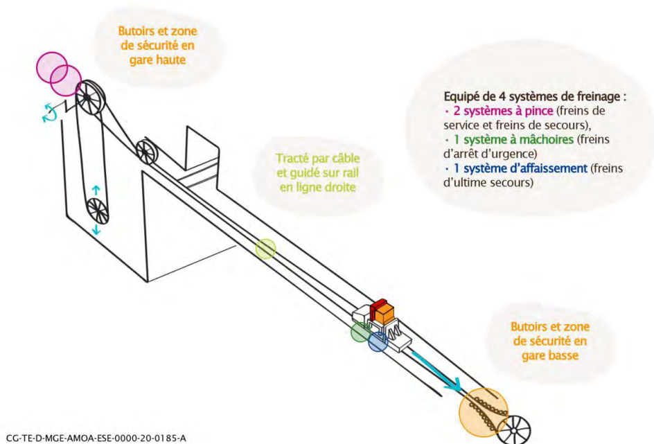
Figure 7-20 Illustration des dispositifs de sécurité du transfert incliné par funiculaire en descenterie
