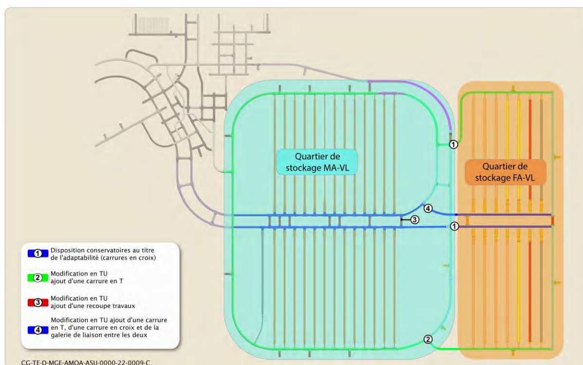
Figure 6-5 Illustration des ouvrages d'un éventuel quartier de stockage FA-VL (hypothèse à terminaison)
