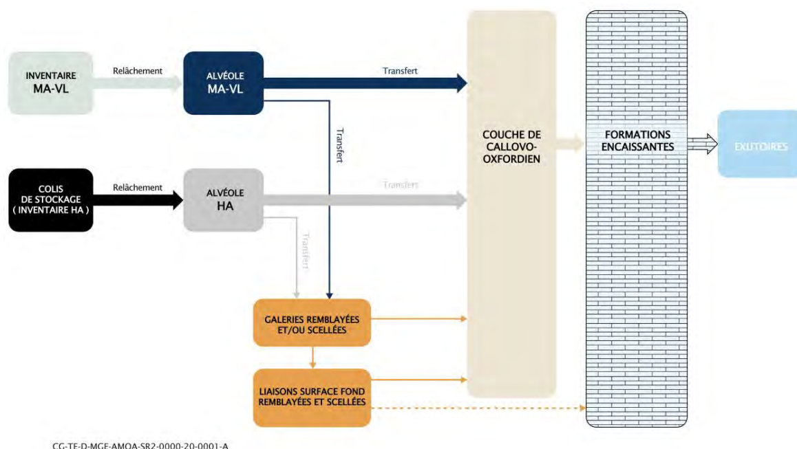
Figure 7-15 Schéma illustratif des composants et des voies de transfert pour le scénario d'évolution normale
