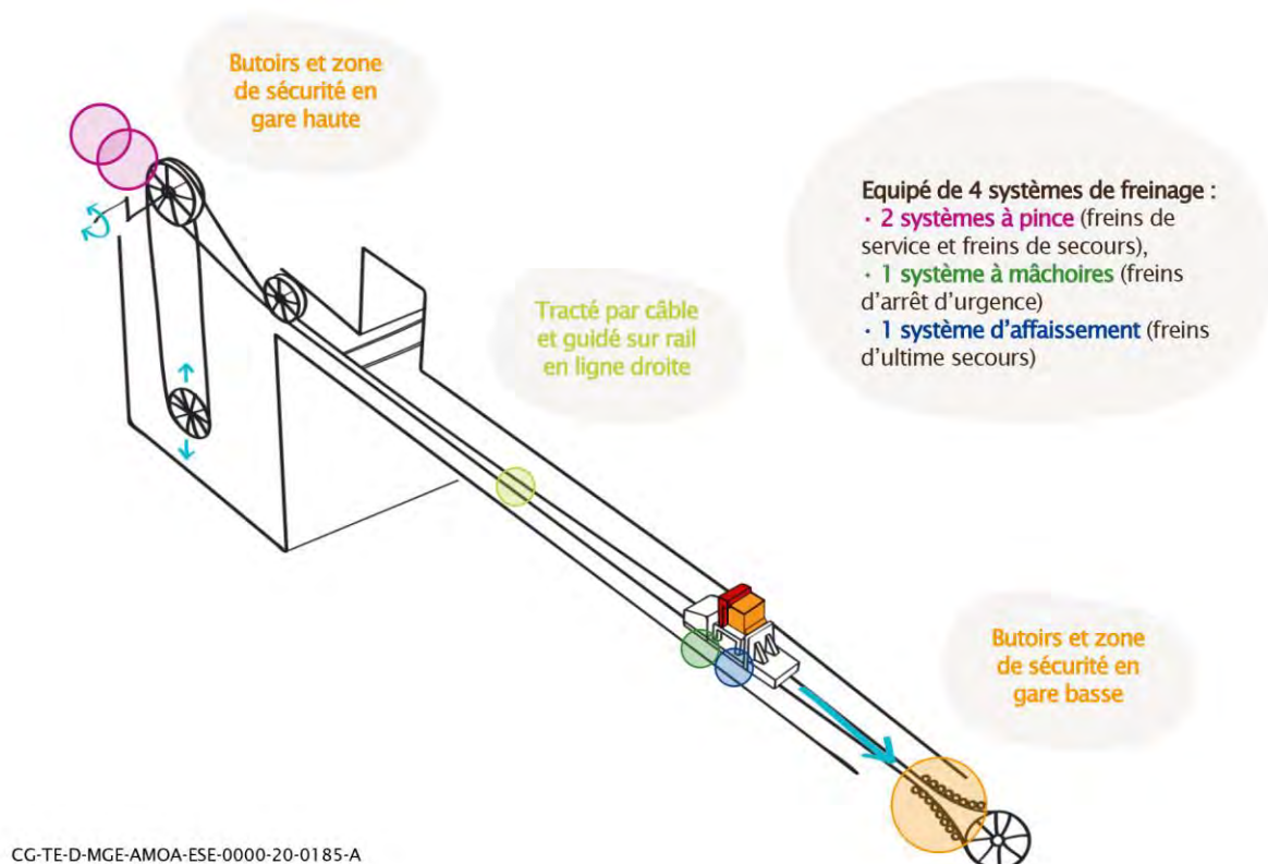
Figure 5-14 Illustration des dispositifs de sécurité du transfert incliné par funiculaire
