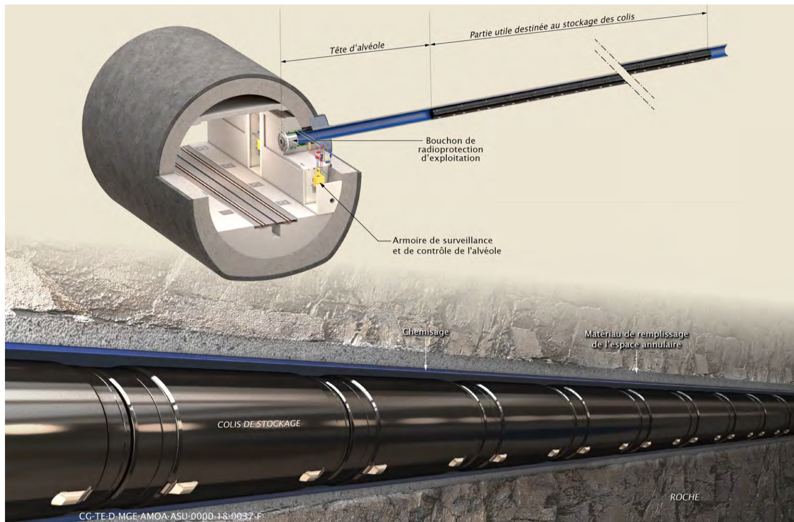
Figure 5-10 Illustration d'un alvéole HA en exploitation
