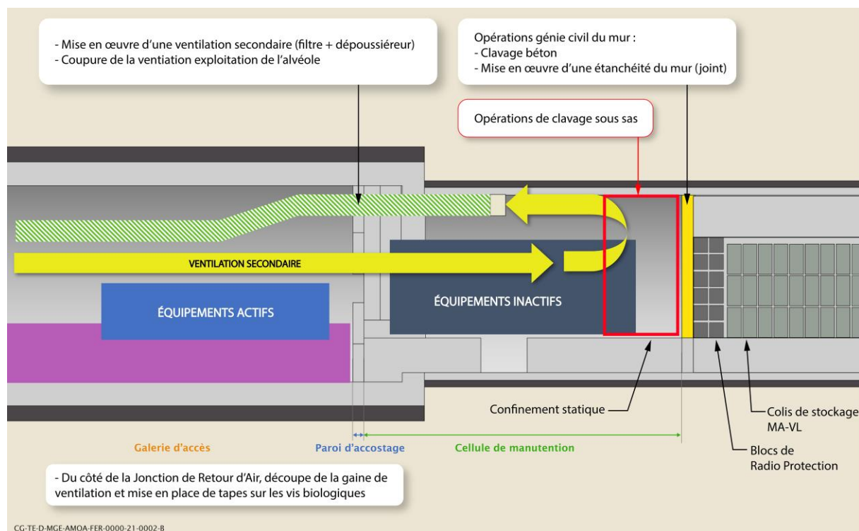
Figure 4-5 Mise en place d'une ventilation secondaire, arrêt de la ventilation exploitation de l'alvéole et mise en œuvre de l'obturation de l'alvéole
