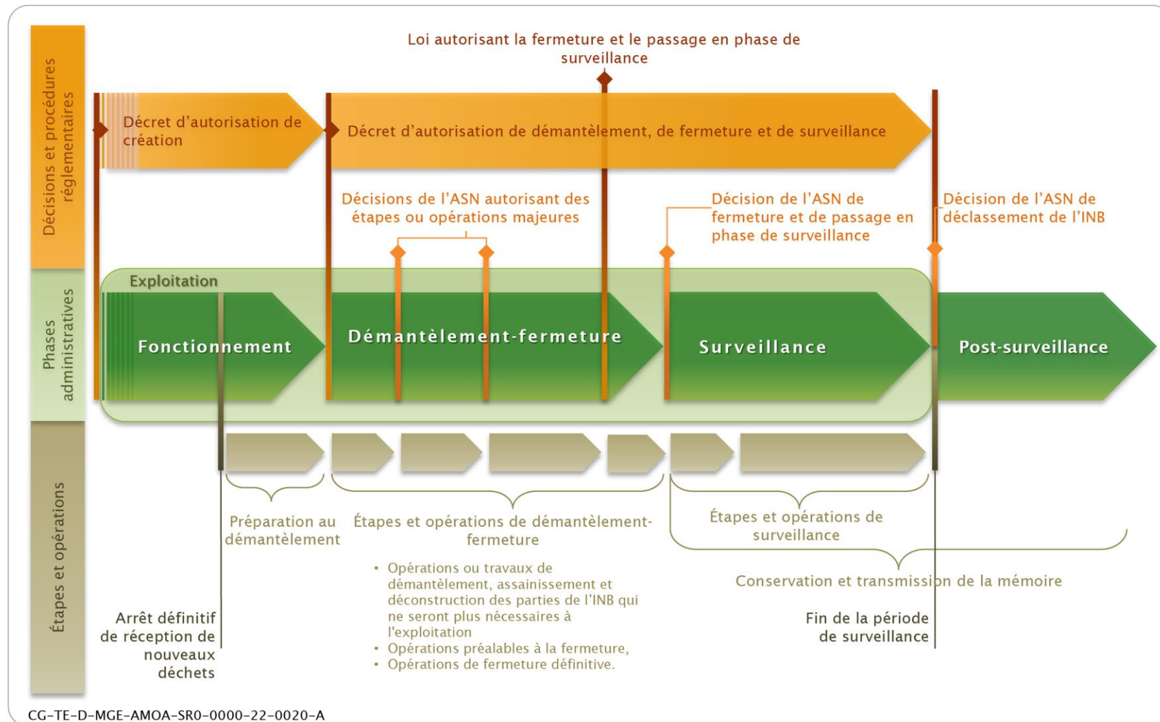
Figure 2-1 Illustration des procédures, des étapes et des opérations de démantèlement, de fermeture et de passage en surveillance de l'INB Cigéo
