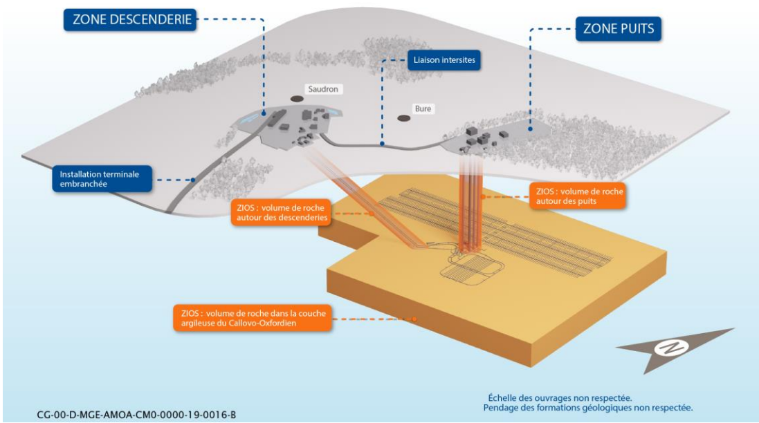
Figure 1-1 Schéma d'organisation de principe du centre de stockage Cigéo
