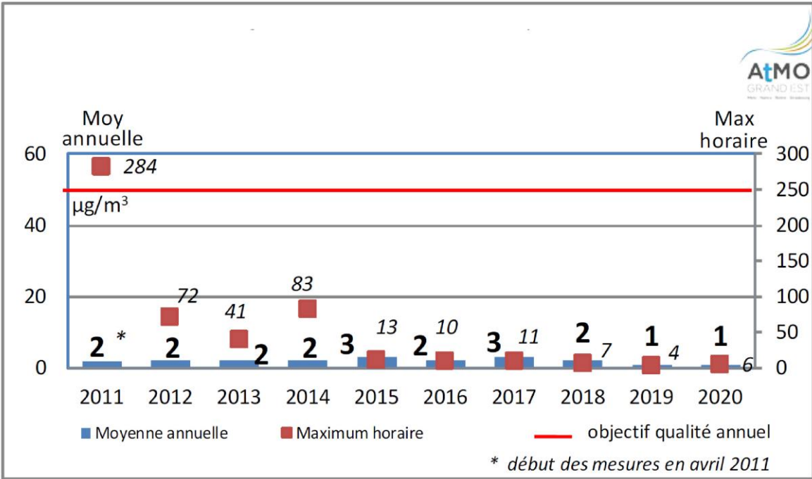
Figure 2-24 Évolution des teneurs moyennes annuelles en SO 2 et des maximas horaires à Houdelaincourt (2011-2020)
