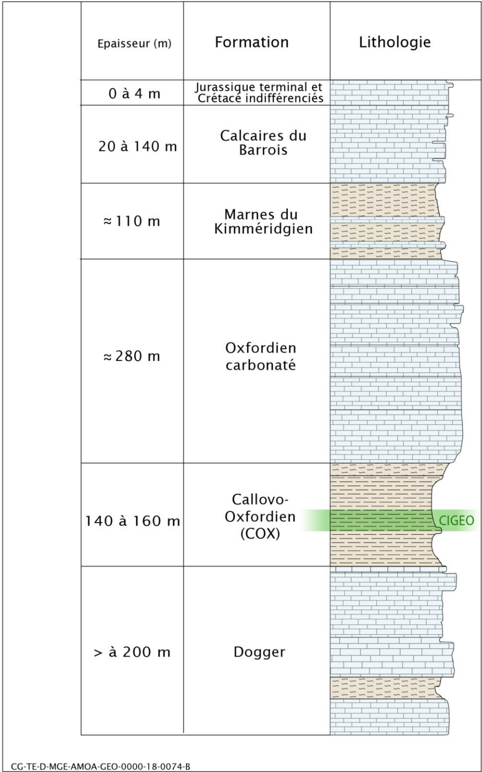
Figure 4-9 Succession schématique des formations géologiques de l'aire d'étude éloignée
