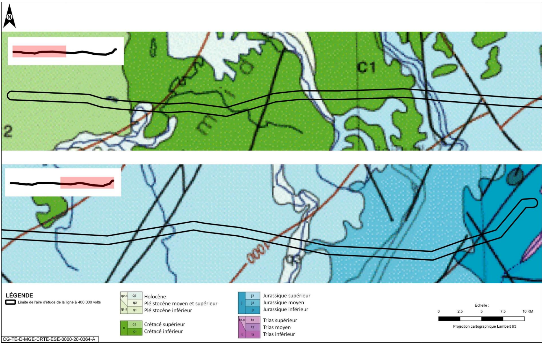
Figure 4-8 Carte géologique simplifiée le long de la ligne électrique 400 kV
