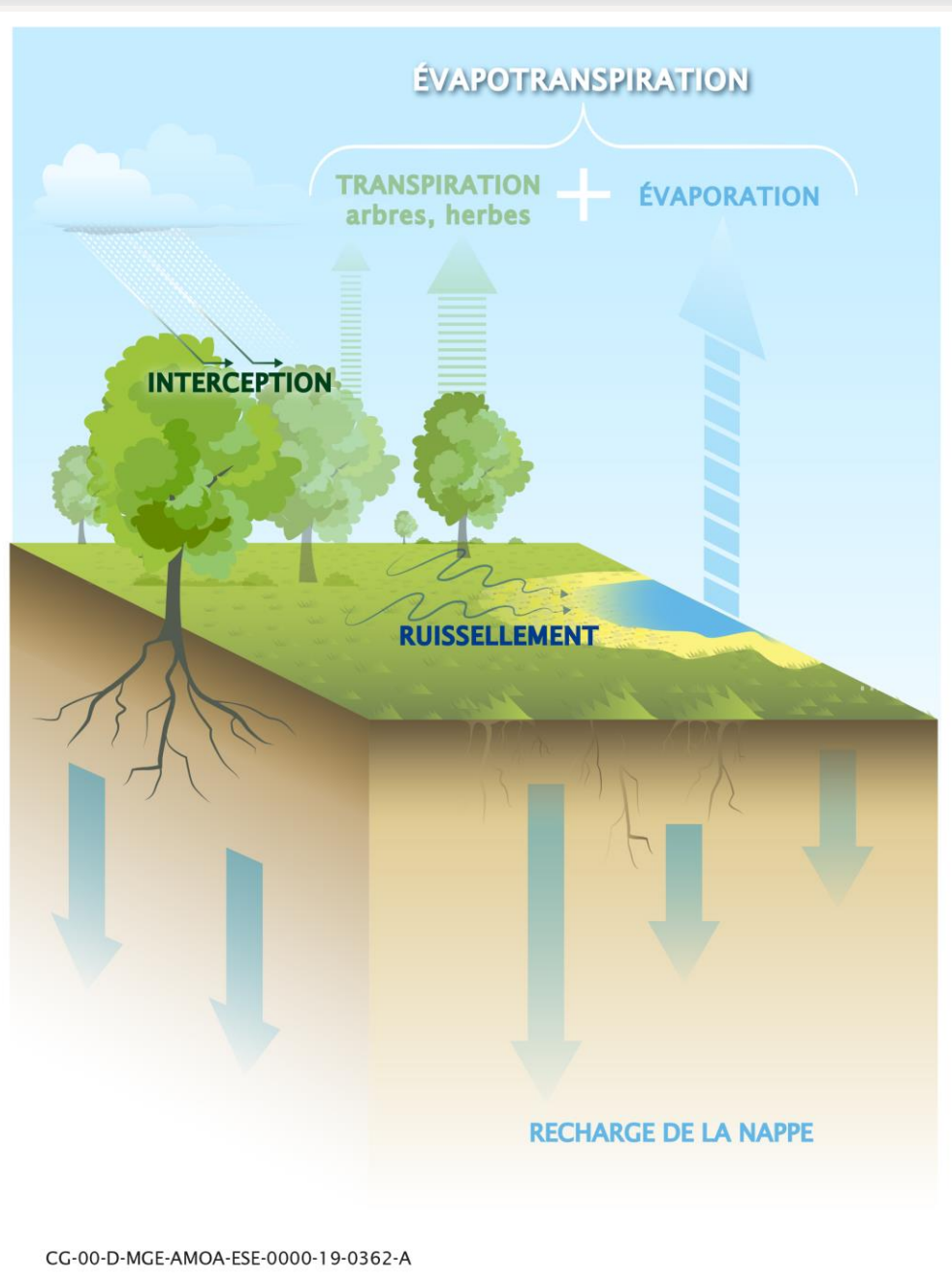
Figure 2-13 Schématisation de l'évapotranspiration
