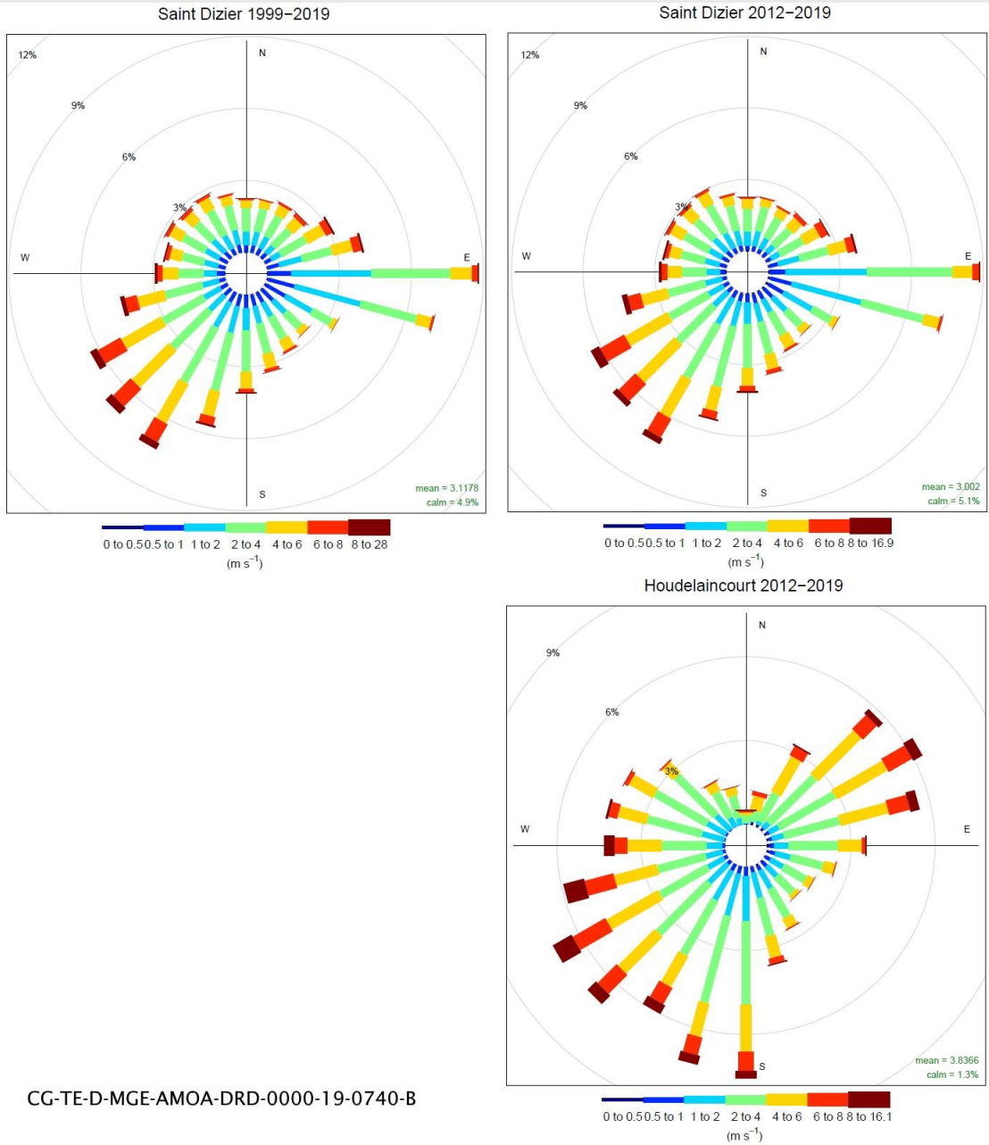
Figure 2-8 Rose des vents de Saint-Dizier, période 1999-2019 (haut à gauche), période 2012-2019 (haut à droite), et de Houdelaincourt période 2012-2019 (bas)
