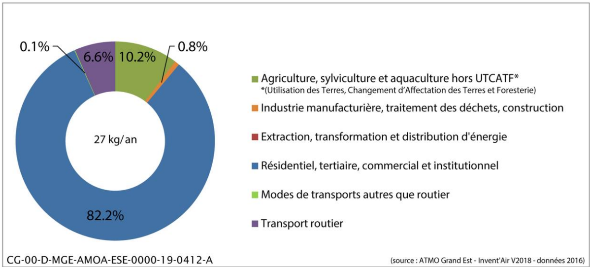
Figure 2-34 Émissions des HAP par secteur d'activité en 2017
