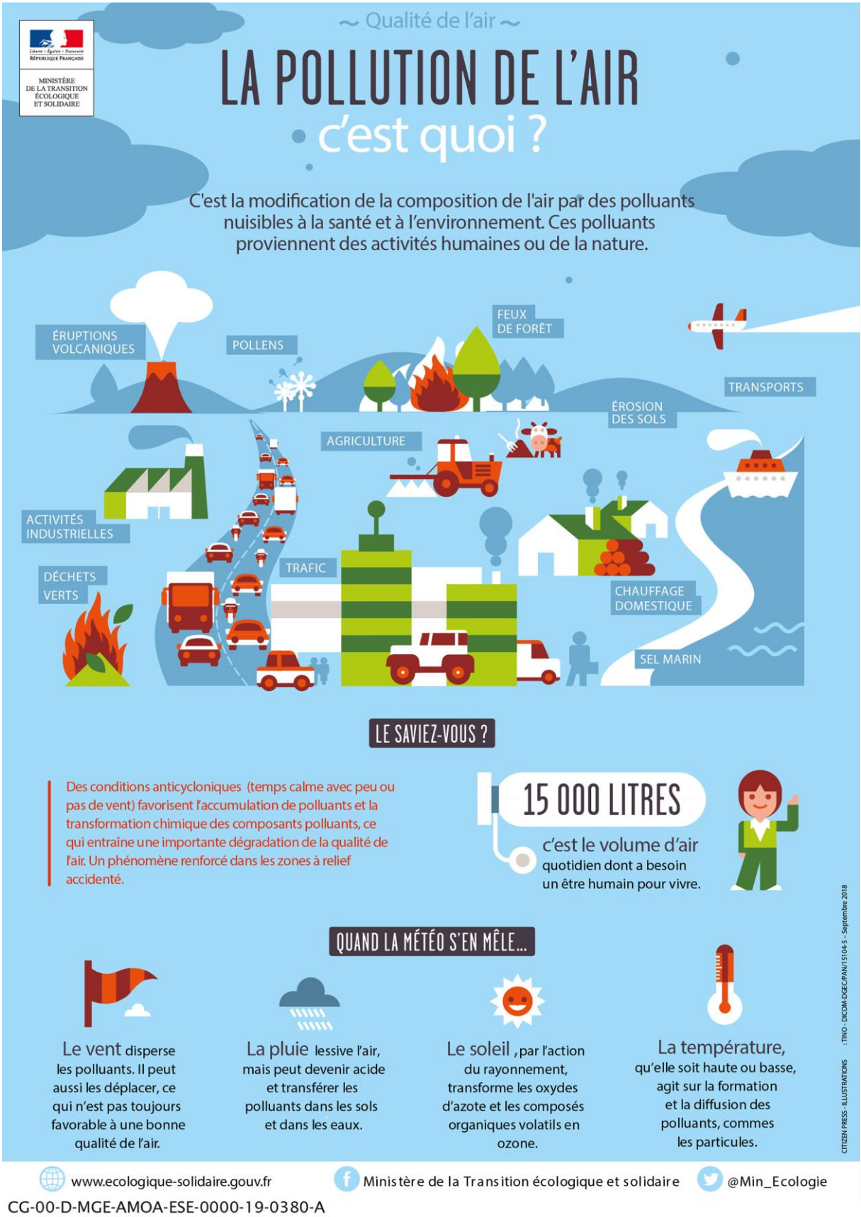
Figure 2-19 Qu'est-ce que la pollution de l'air ?
