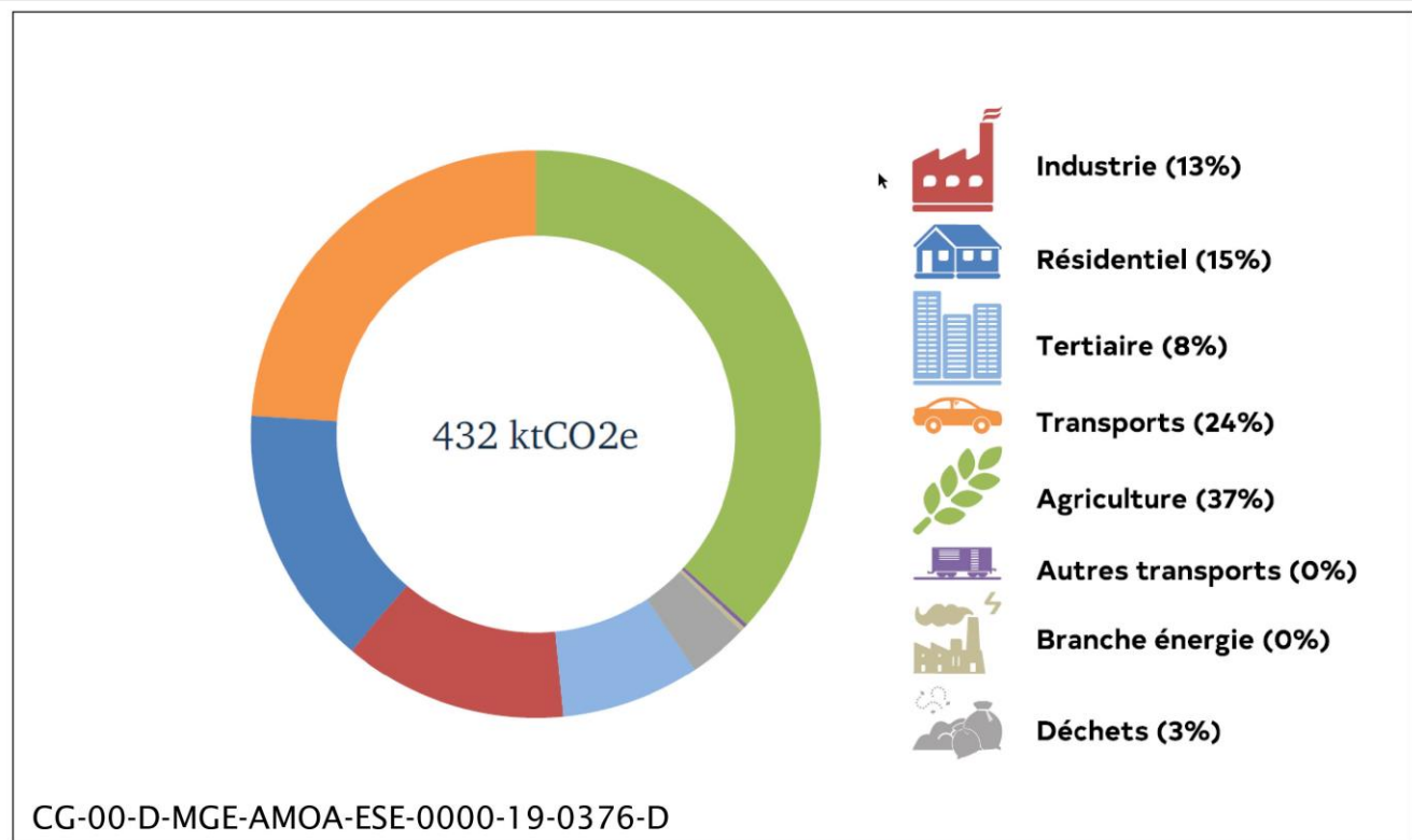
Figure 2-17 Émissions directes et indirectes de gaz à effet de serre du Pays Barrois en 2020 (tCO 2 e)
