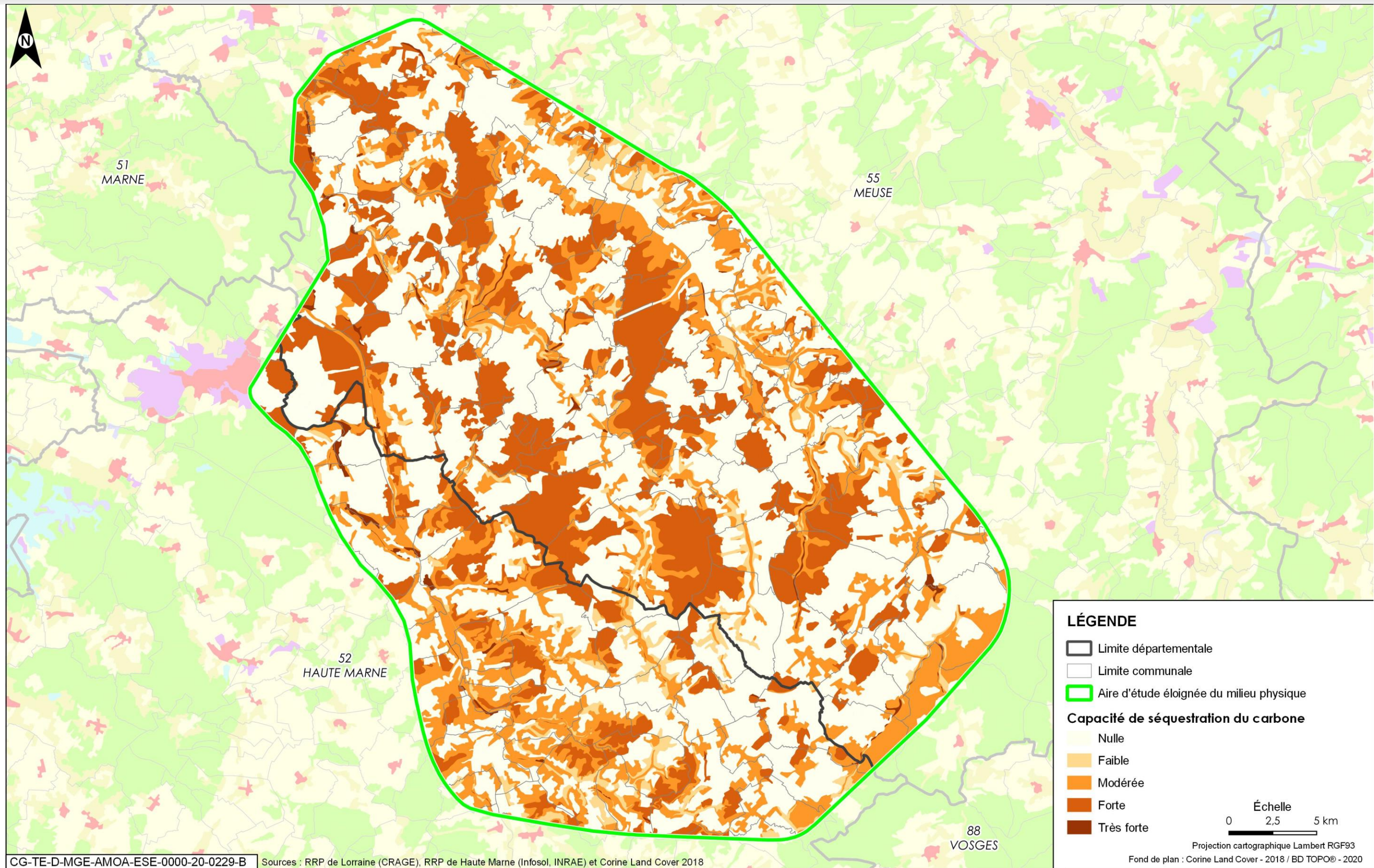
Figure 2-18 Carte de la capacité de séquestration carbone dans l'aire d'étude éloignée du milieu physique
