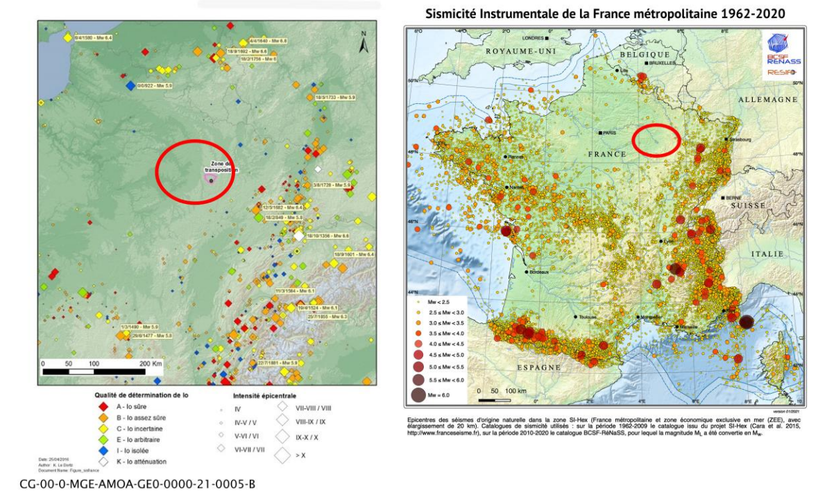
Figure 4-17 Sismicité historique (base SisFrance à gauche) et instrumentale (base SiHex – Cara et al., 2015 à droite) (80, 81)) et localisation de la région de Meuse/Haute-Marne
