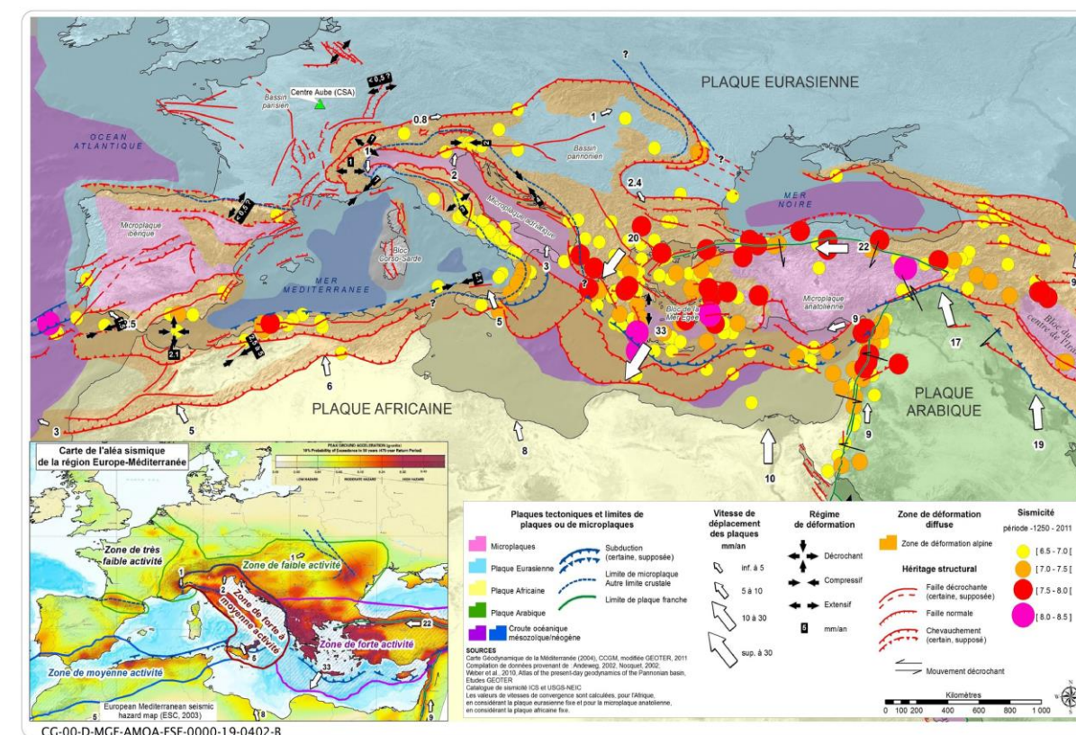
Figure 4-3 Contexte géodynamique de la plateforme ouest-européenne (et de la France) au droit de la collision Europe/Afrique
