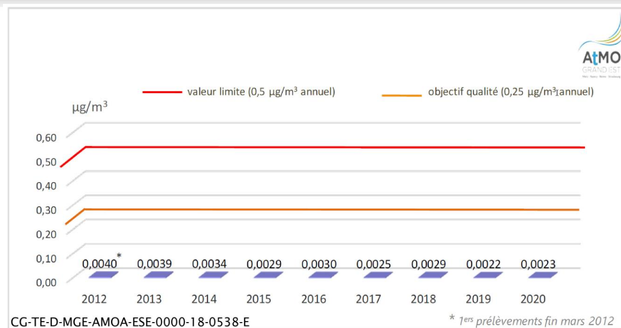
Figure 2-41 Évolution des concentrations en plomb dans les PM10 à Houdelaincourt (2012-2020)
