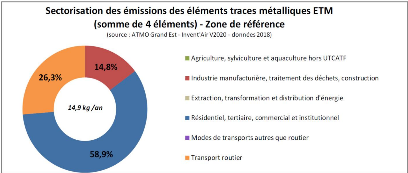
Figure 2-36 Sectorisation des émissions des éléments traces métalliques en 2019
