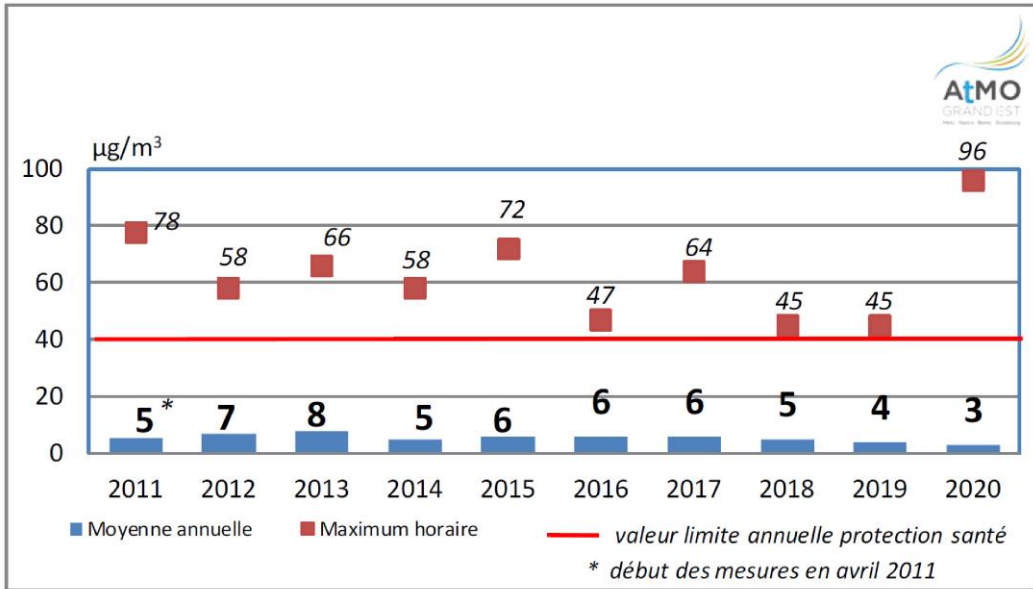
Figure 2-22 Évolution des teneurs annuelles en NO 2 et des maxima horaires à Houdelaincourt (2011-2020)
