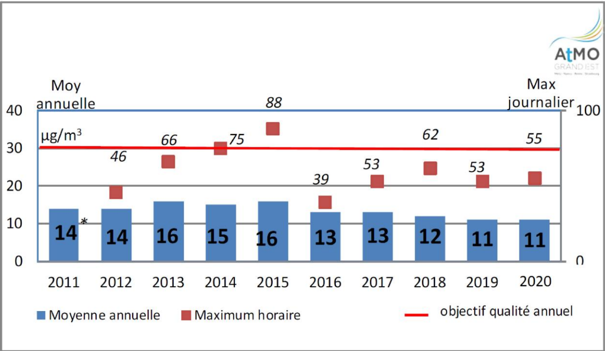
Figure 2-29 Évolution des concentrations annuelles et des maxima journaliers en PM 10 à Houdelaincourt (2011-2020)
