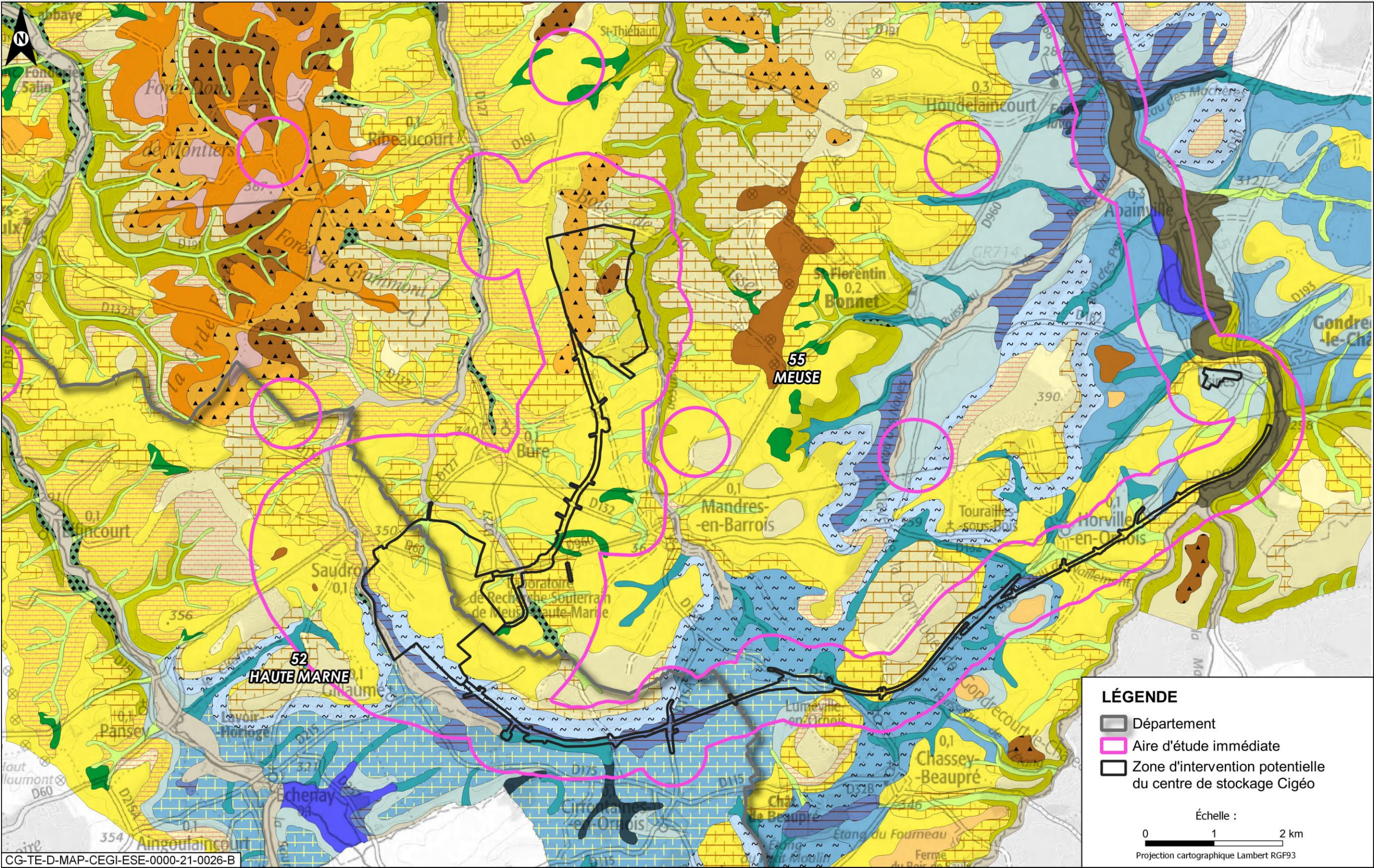
Figure 3-11 Carte pédologique au 1/50 000 au niveau de la zone d'intervention potentielle du centre de stockage Cigéo
