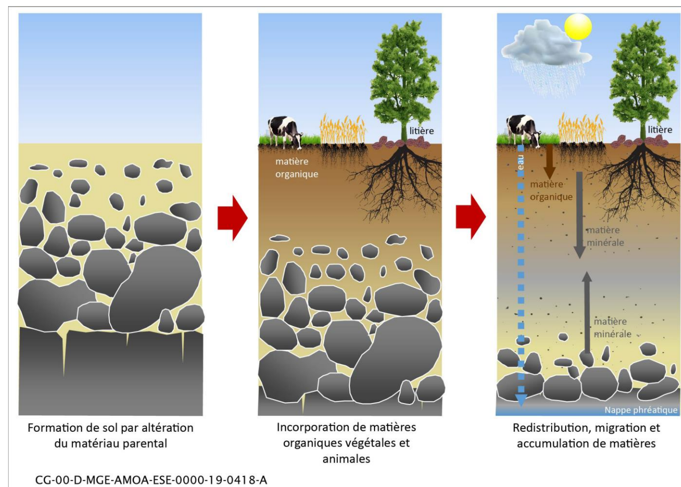
Figure 3-9 Schématisation des étapes de la formation d'un sol
