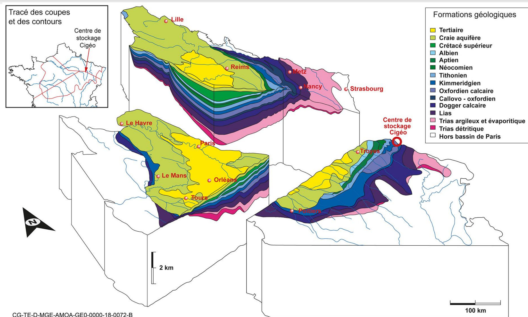
Figure 4-7 Bloc diagramme géologique du Bassin parisien
