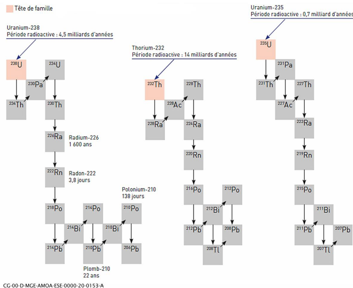
Figure 3-13 Chaînes de désintégration de l'Uranium-238, du Thiorium-232 et de l'Uranium-235
