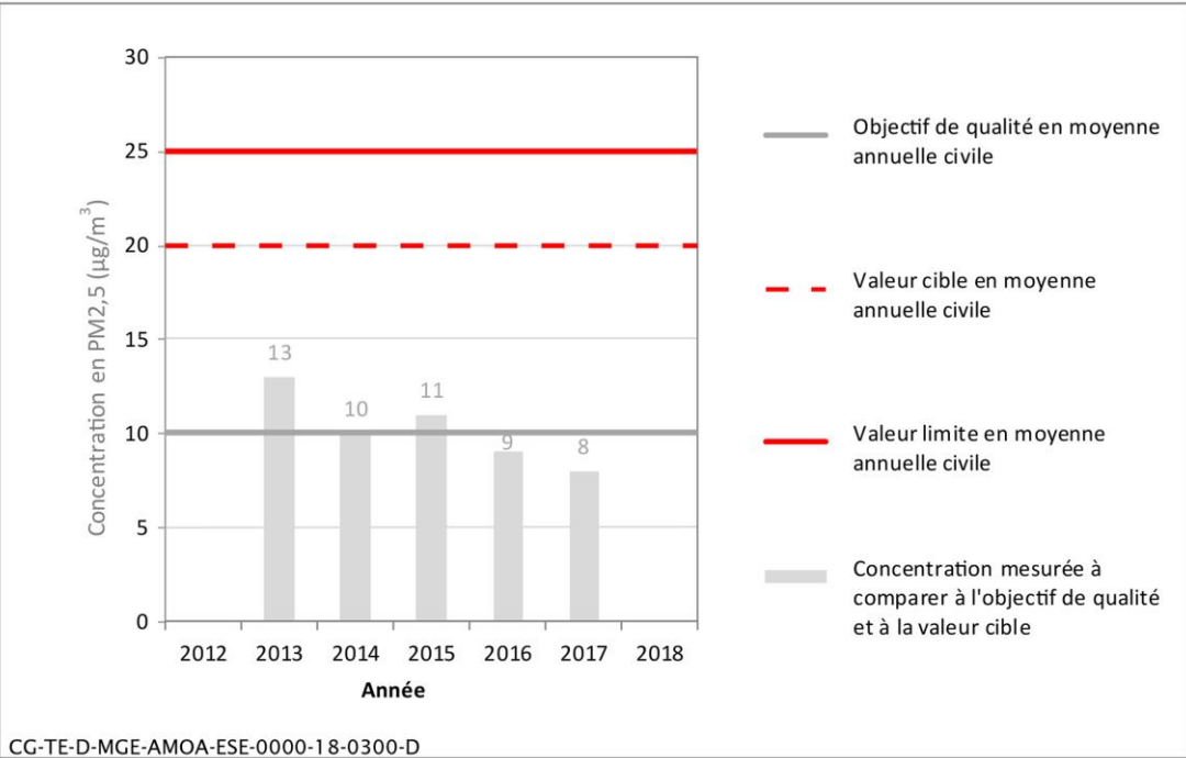
Figure 2-31 Évolution des concentrations en PM 2,5 sur Houdelaincourt (2012-2018)
