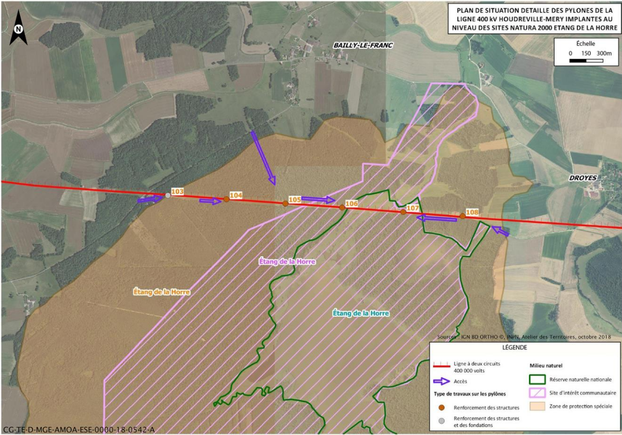
Figure 6-2 Localisation des pylônes de la ligne 400 kV dans le secteur de l'Étang de la Horre
