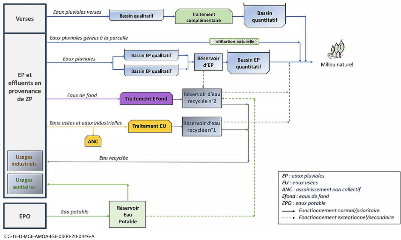
Figure 5-57 Schéma illustratif de principe de la gestion des eaux au droit de la zone puits en fin d'aménagements préalables et en phase de construction initiale
