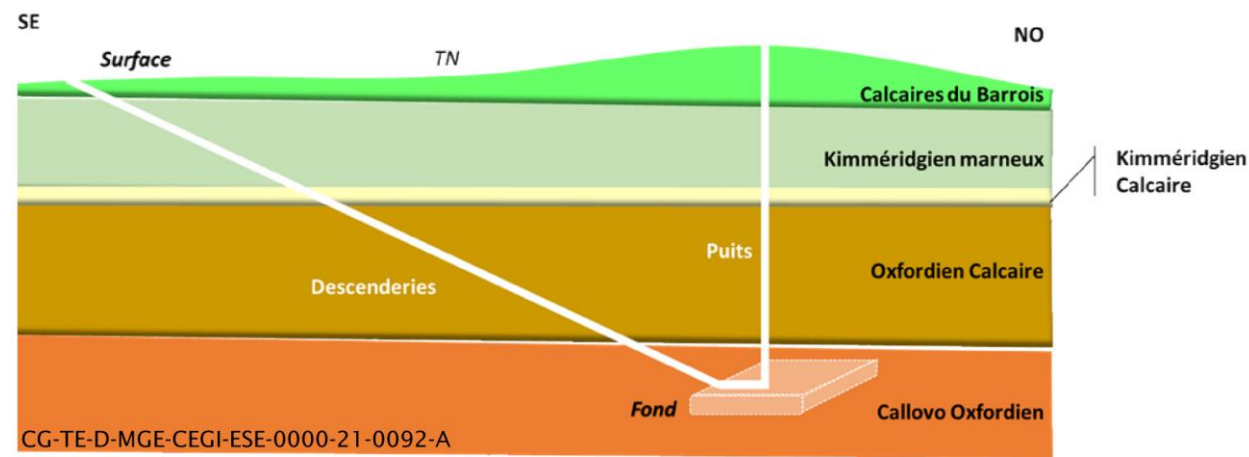
Figure 5-6 Coupe schématique des grandes formations géologiques traversées
