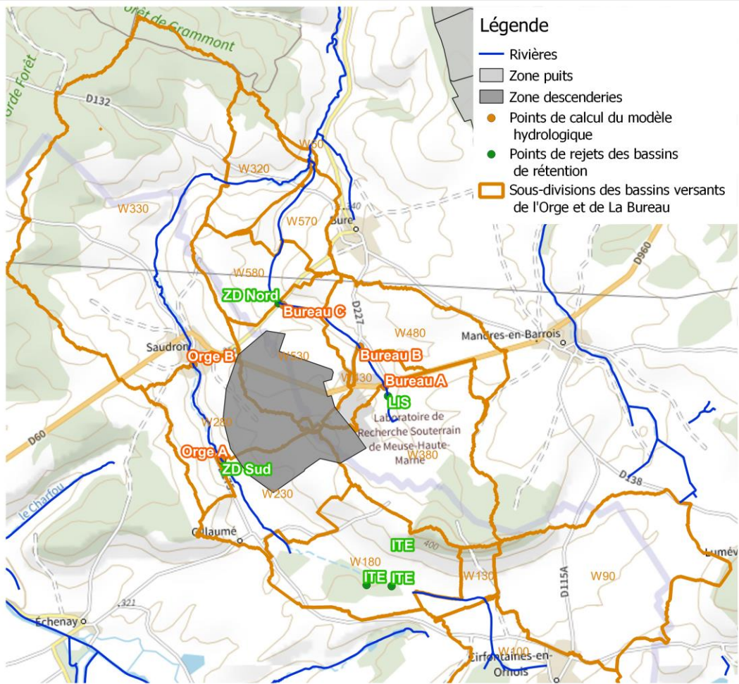
Figure 5-42 Localisation des bassins et points de calcul de la simulation hydrologique pour l'Orge et la Bureau
