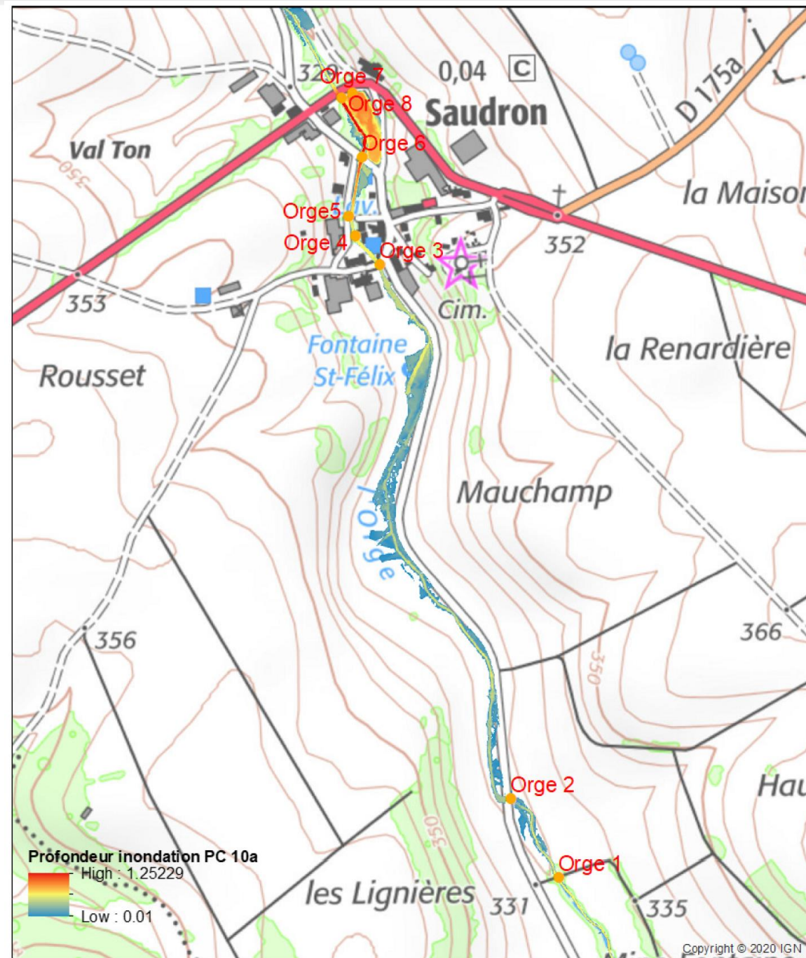
Figure 5-45 L'Orge : étendue et profondeur d'inondation (m), phase de construction initiale avec une période de retour de 10 ans
