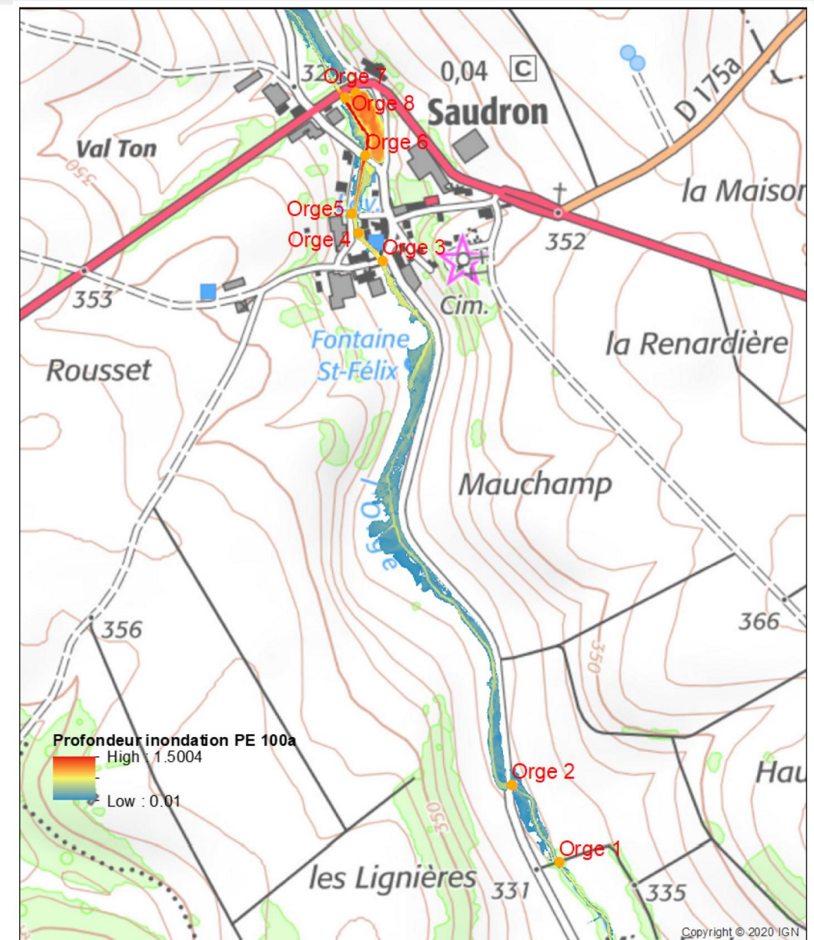
Figure 5-46 L'Orge : étendue et profondeur d'inondation (m), phase de fonctionnement avec une période de retour de 100 ans
