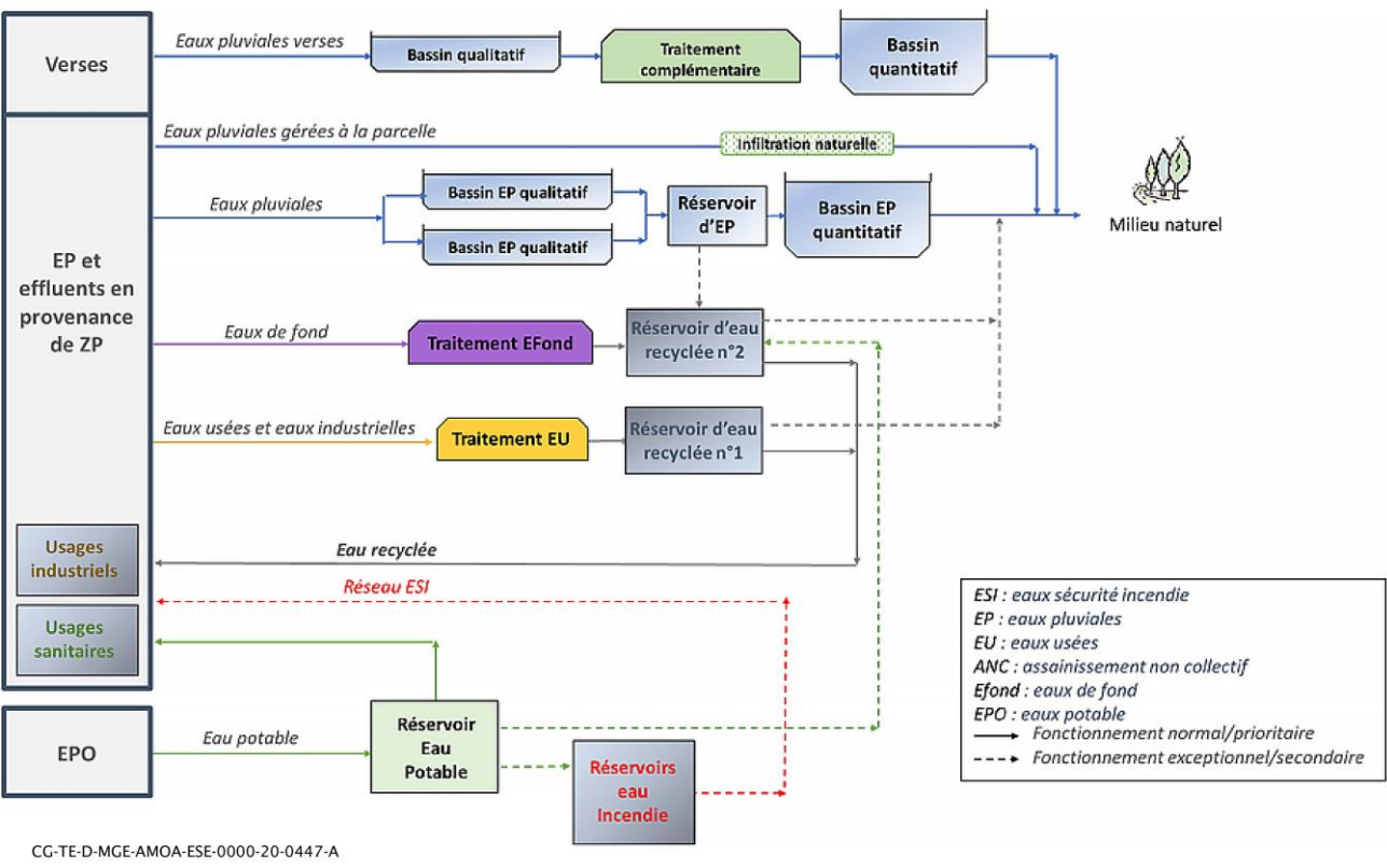
Figure 5-58 Schéma illustratif de principe de la gestion des eaux au droit de la zone puits en phase de fonctionnement
