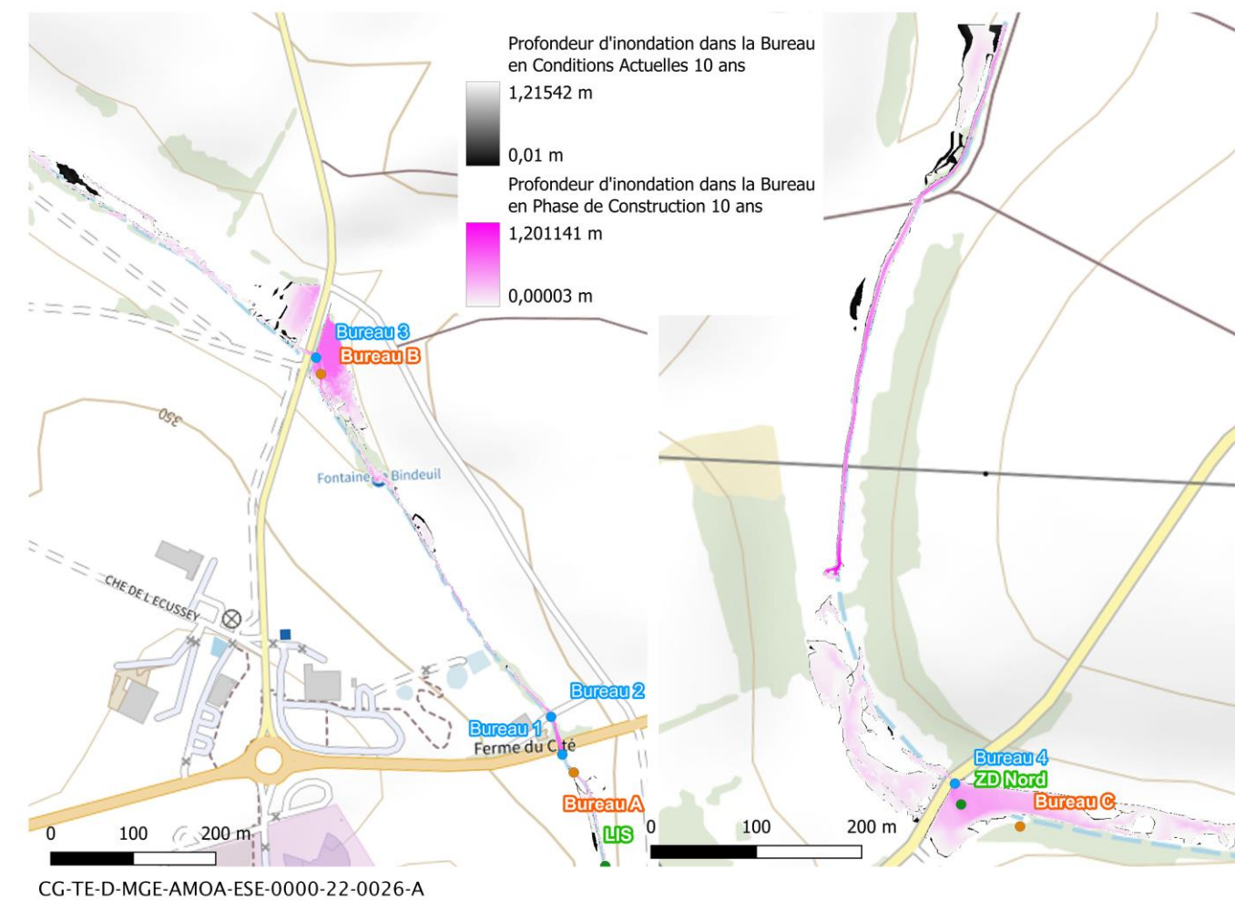
Figure 5-47 Profondeurs d'inondation dans la Bureau en conditions actuelles et en phase de construction initiale pour une période de retour 10 ans
