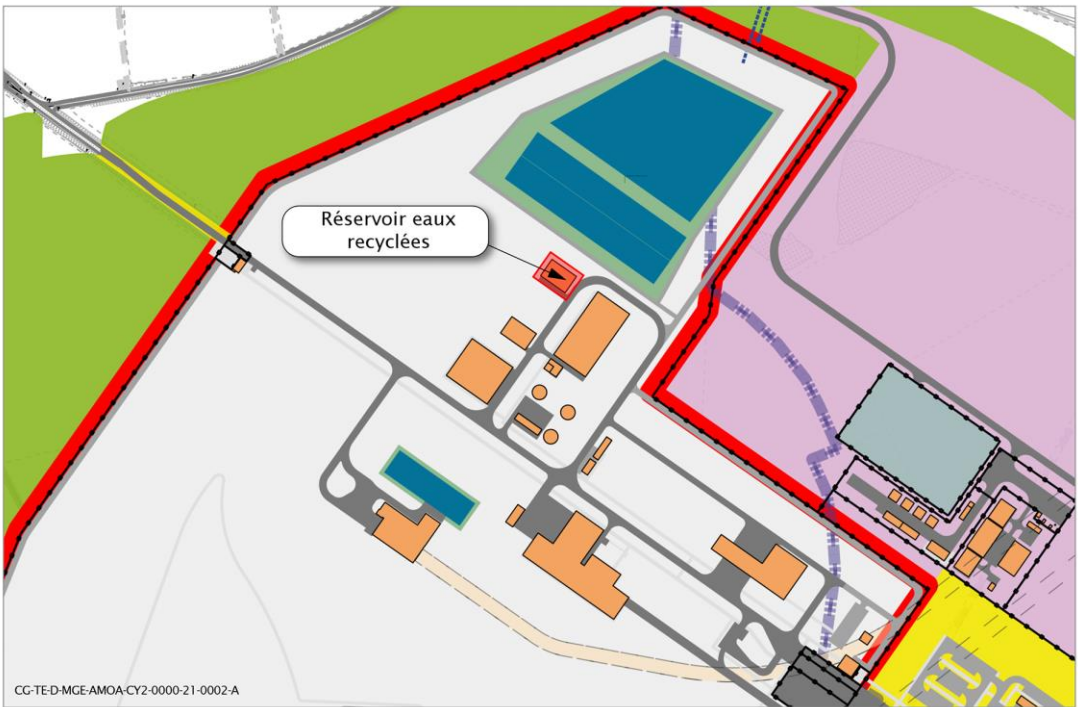
Figure 5-35 Localisation des réservoirs de distribution des eaux recyclées en zone descendrie
