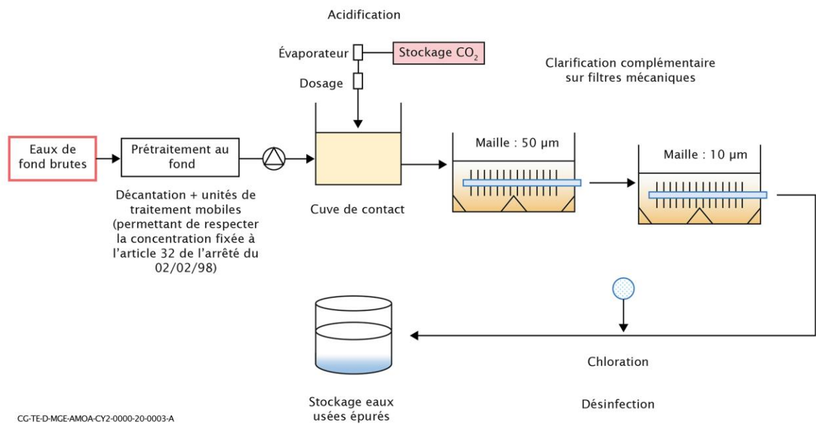
Figure 5-38 Schéma illustratif d'ensemble du dispositif de traitement des eaux de fond
