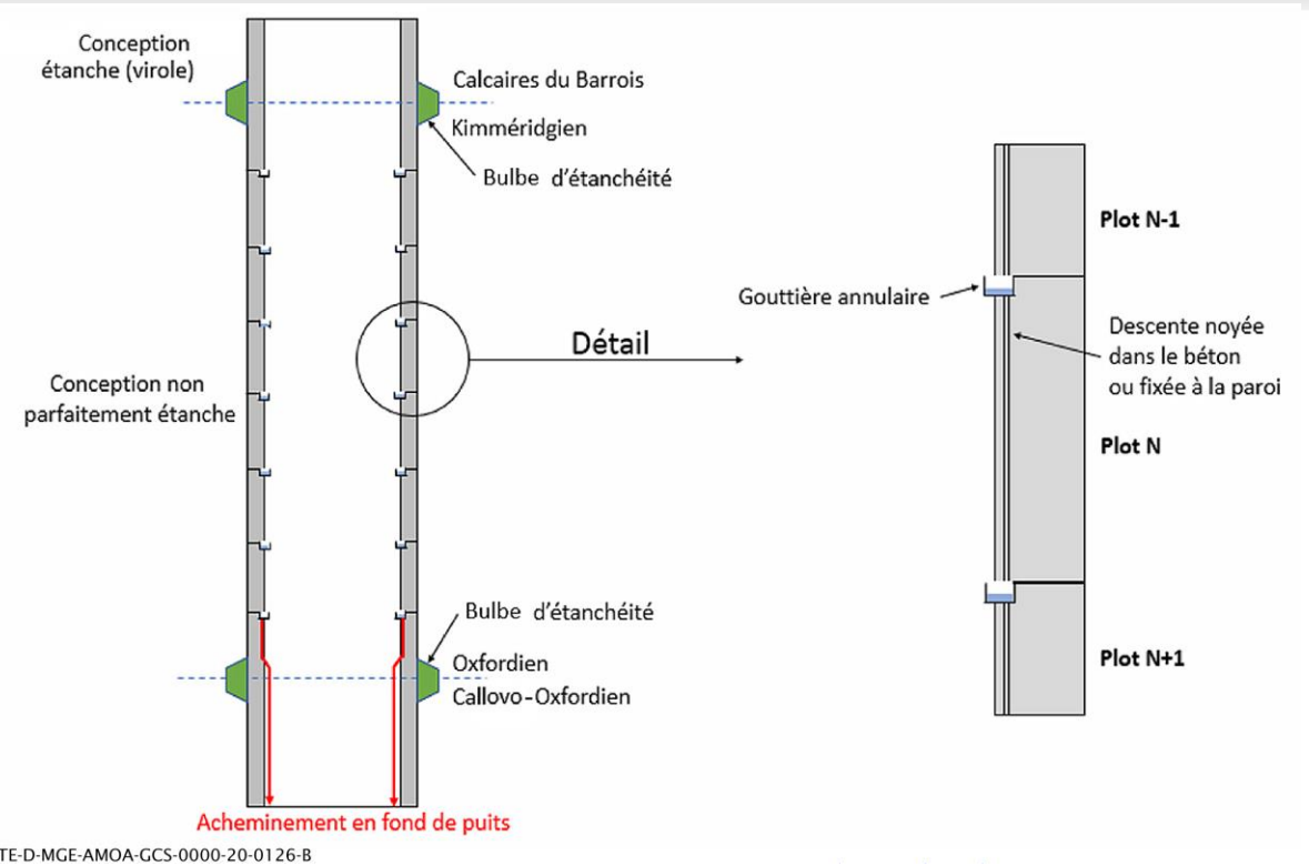
Figure 5-10 Schéma de principe de la collecte des eaux d'infiltration pour les puits semi-étanches)
