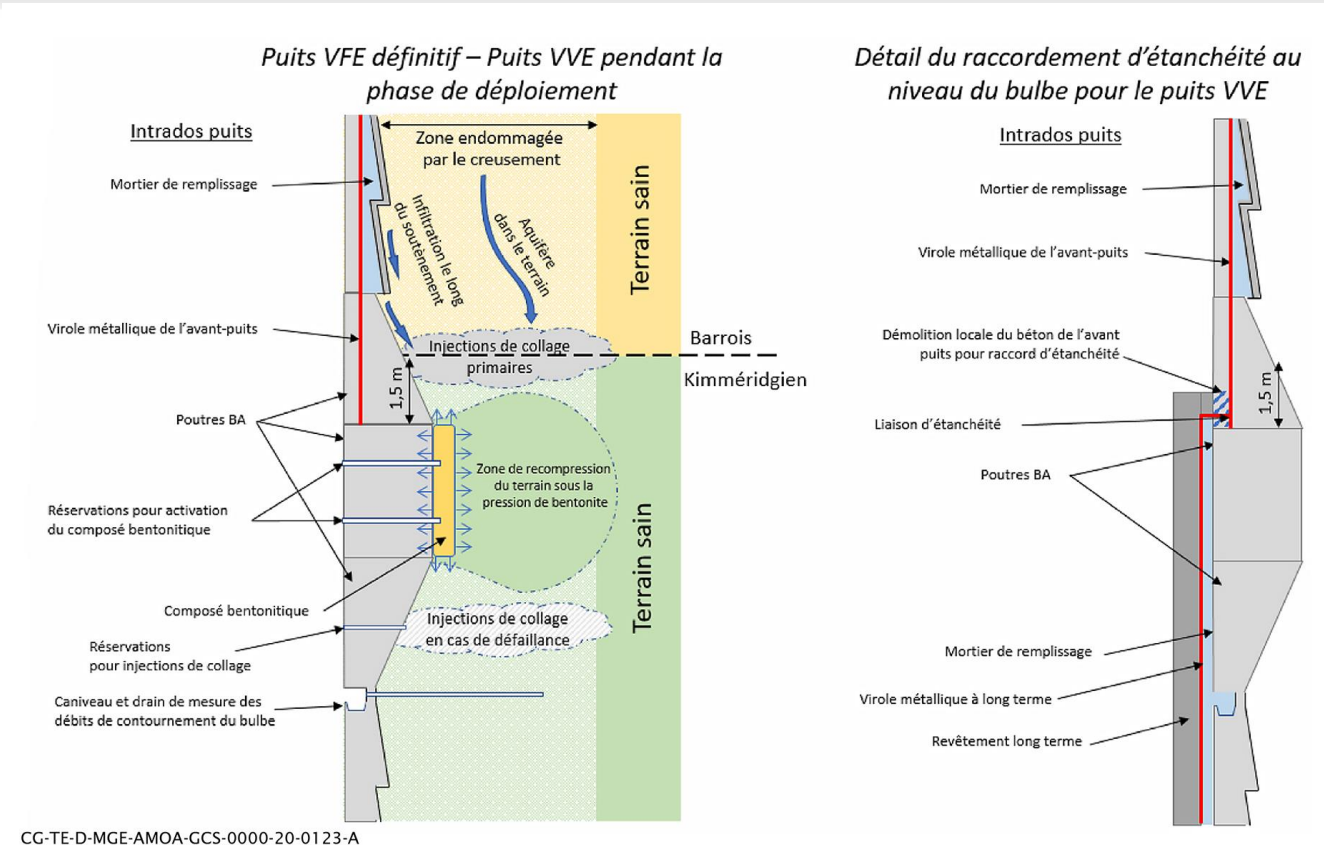
Figure 5-12 Vue en coupe d'un bulbe d'étanchéité
