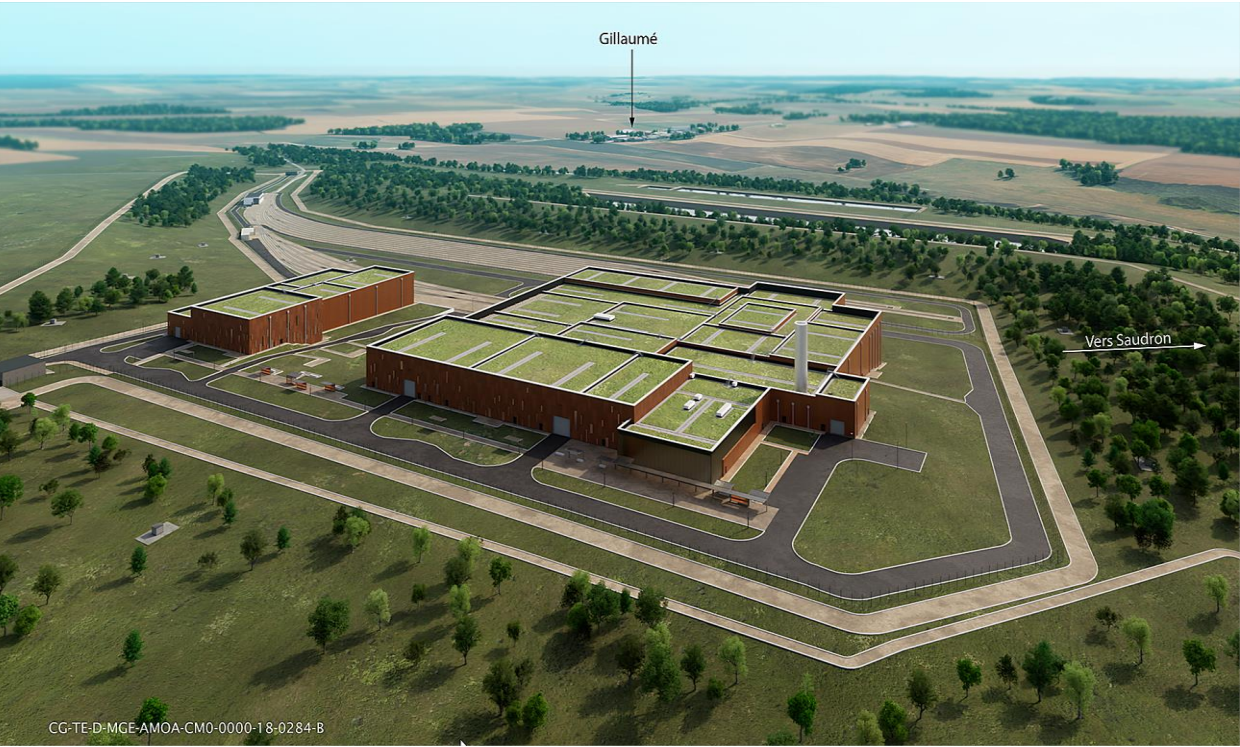
Figure 5-13 Exemple de configuration possible du bâtiment EP1 et de la tête de descendrière
