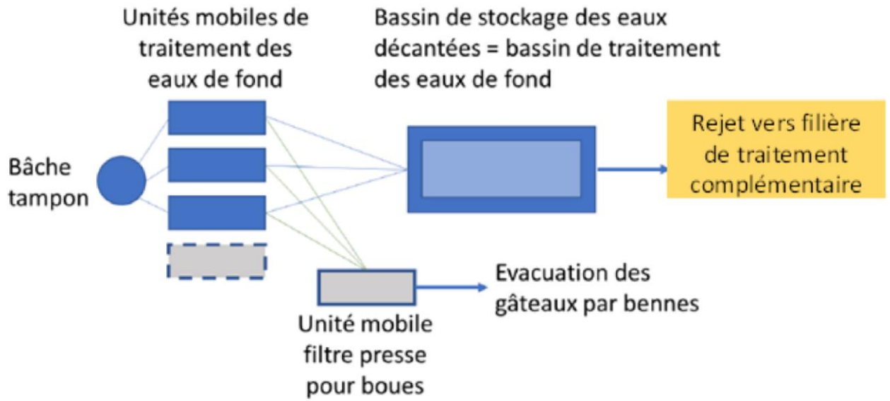
Figure 5-37 Filière de traitement des eaux de fond prévue en premier traitement
