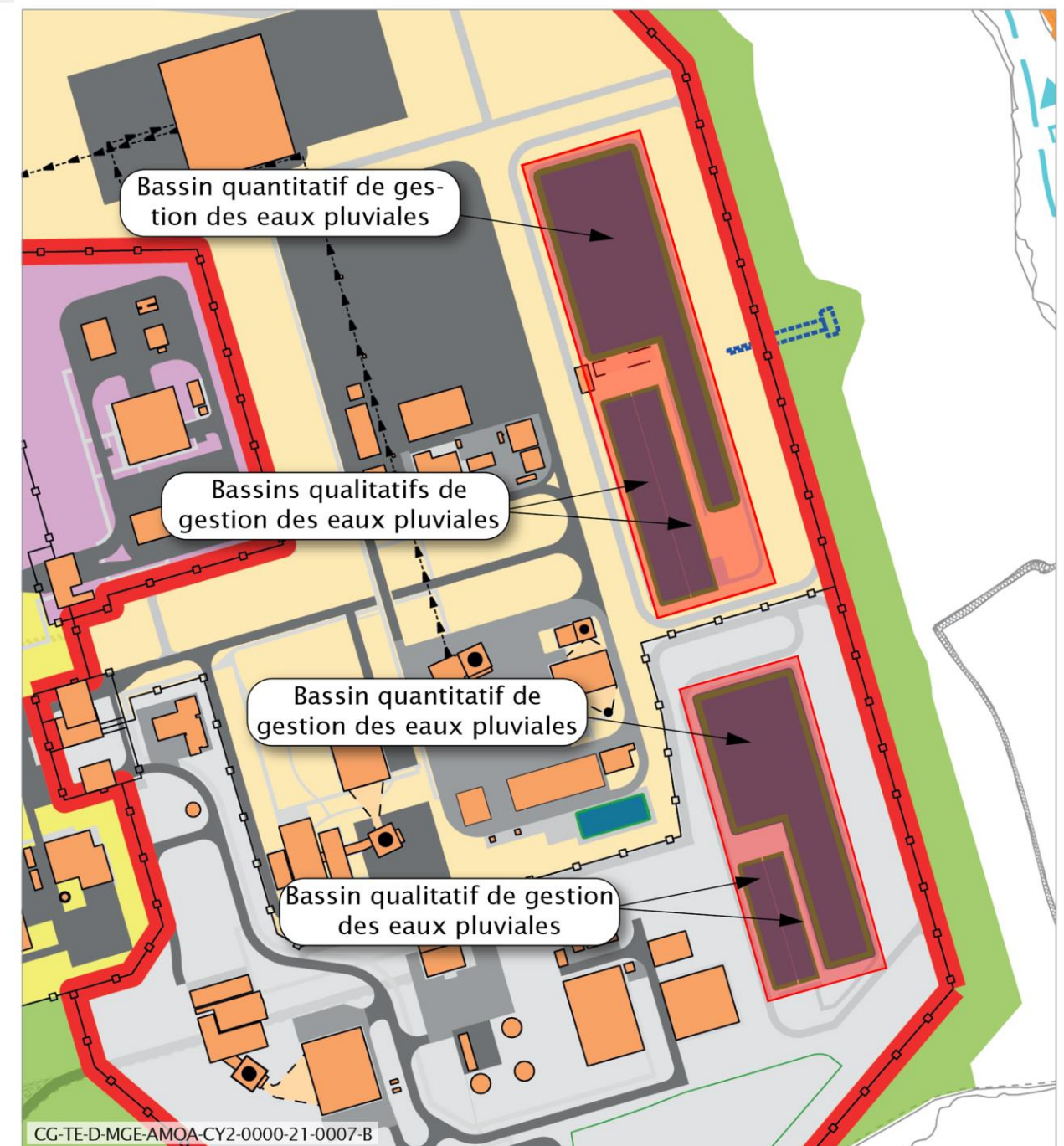
Figure 5-21 Localisation des ouvrages liés à la gestion des eaux pluviales en zone puits
