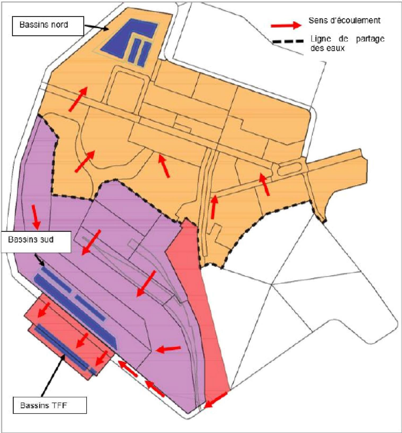
Figure 5-14 Schéma d'écoulement des eaux en zone descendrière
