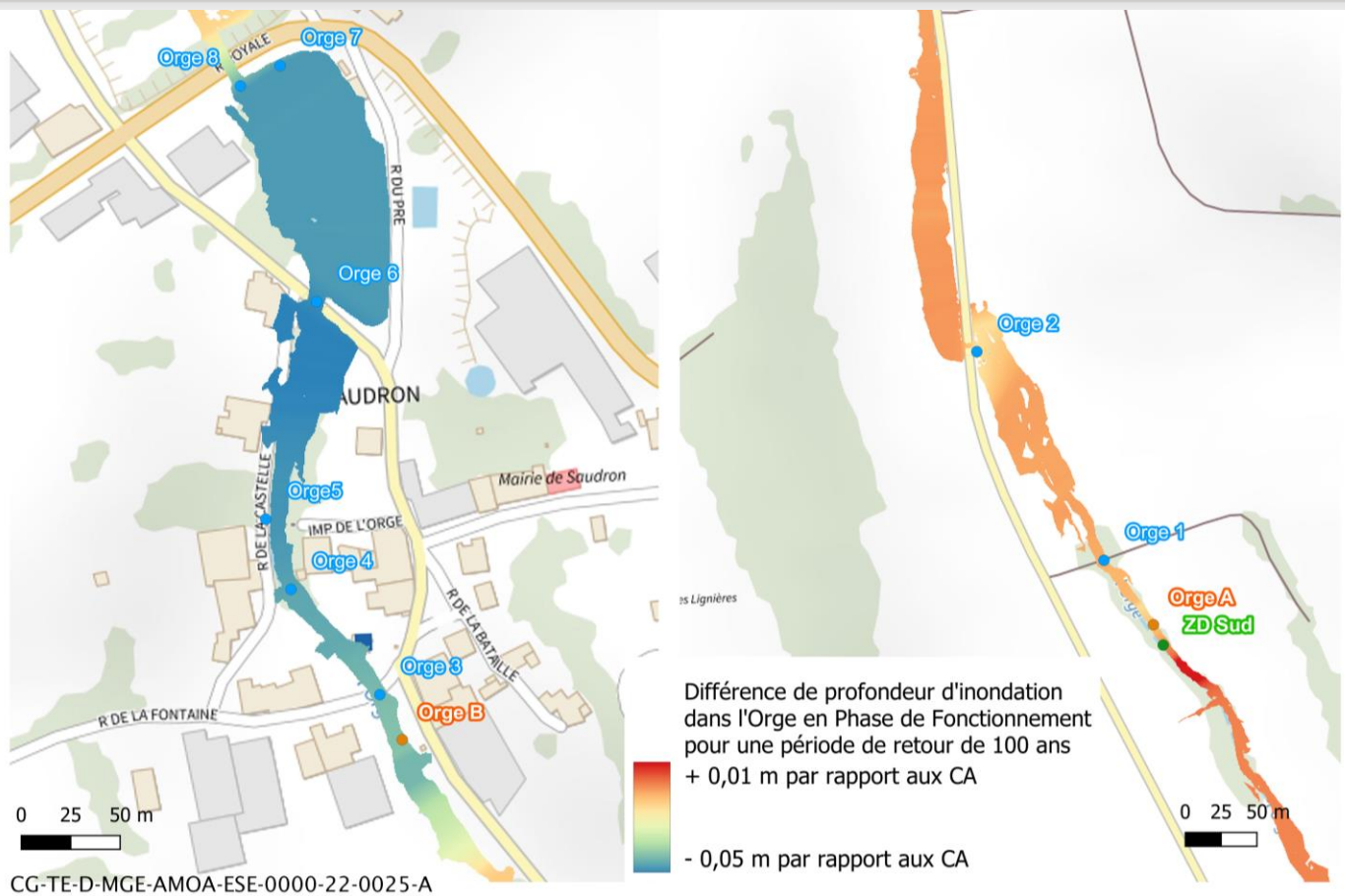
Figure 5-44 Différence de profondeur d'inondation dans l'Orge en phase de fonctionnement par rapport aux conditions actuelles (CA) pour une période de retour 100 ans
