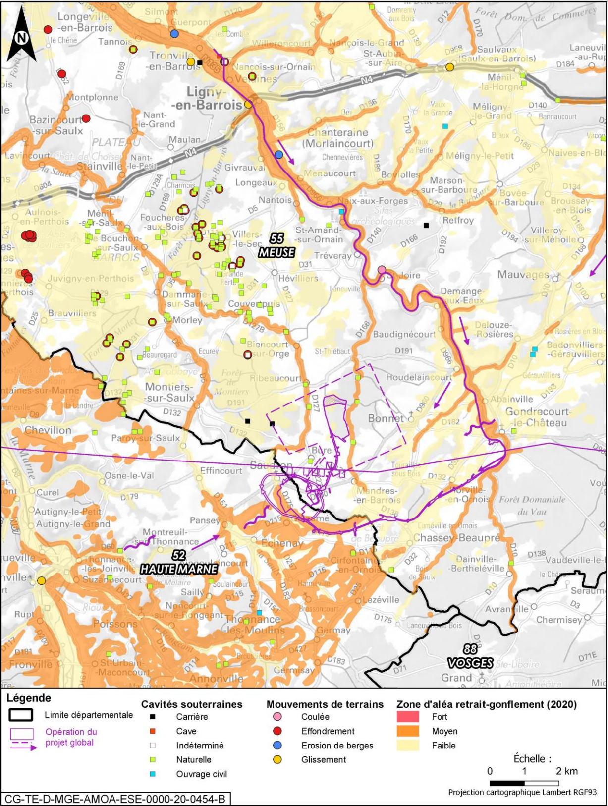
Figure 4-7 Risque de mouvements de terrain
