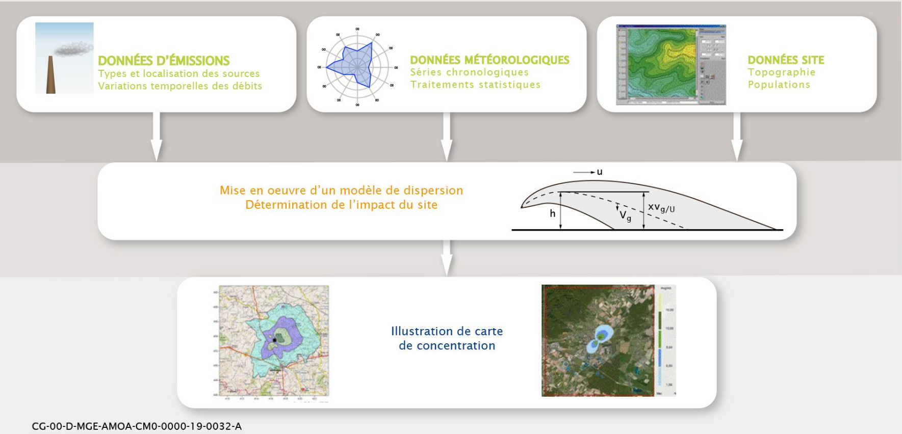
Figure 2-18 Illustration des modélisations de la dispersion atmosphérique des gaz et aérosols
