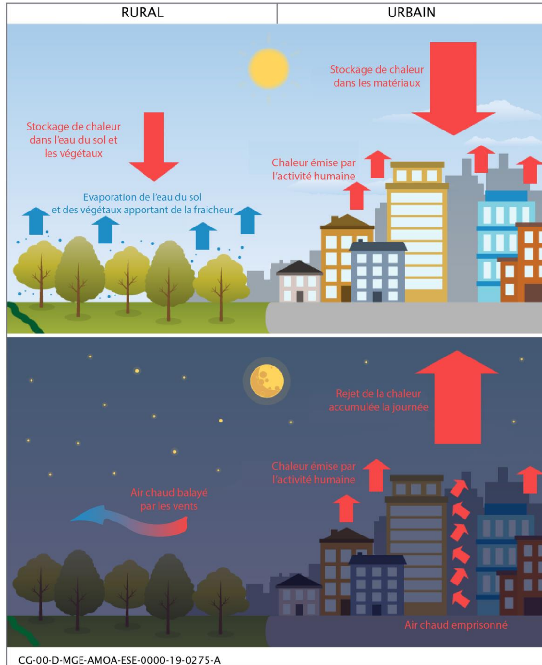
Figure 2-2 Représentation schématique du phénomène d'îlot de chaleur
