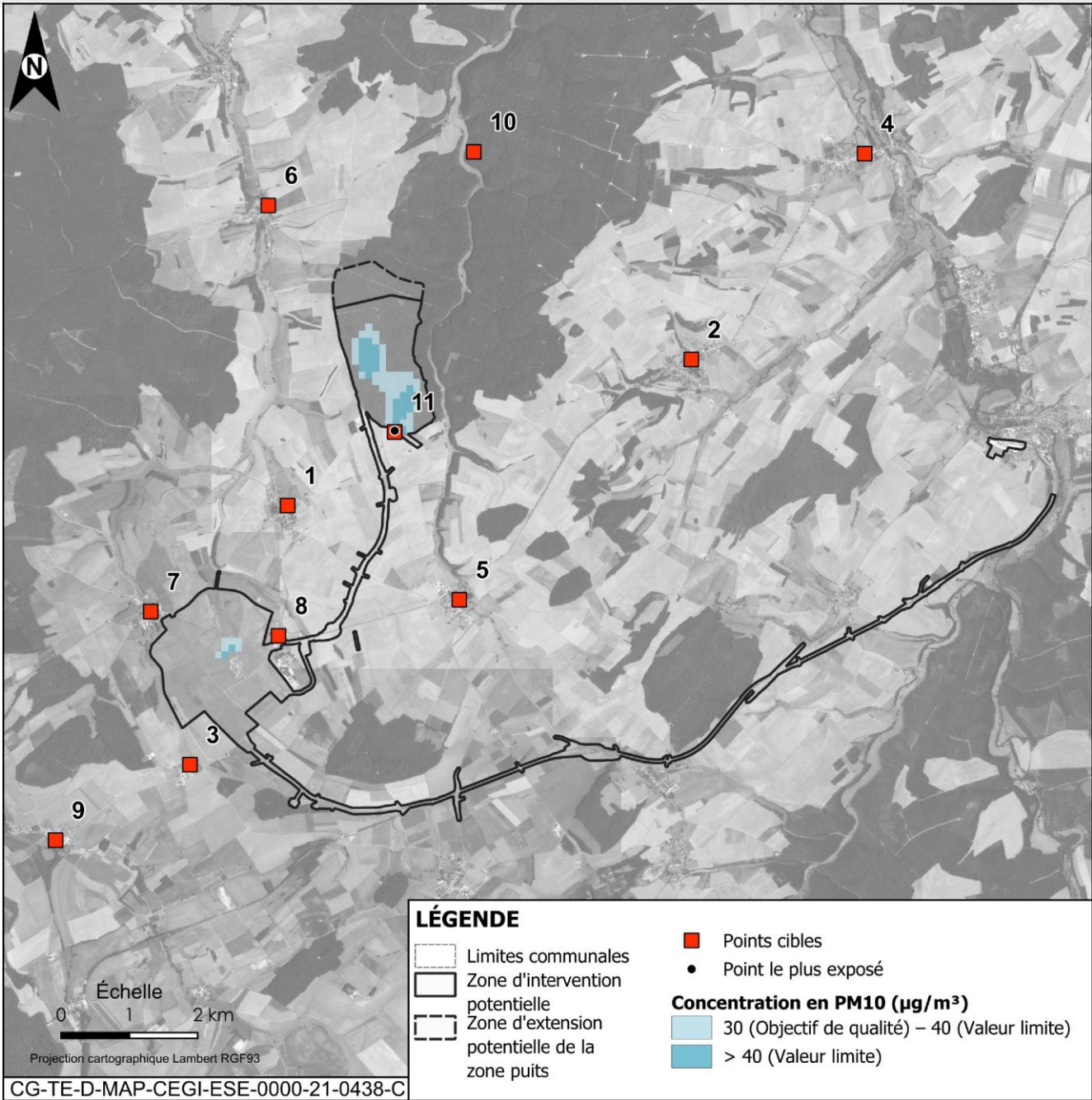
Figure 2-10 Concentration en PM 10 (µg/m 3 ) en phase de construction initiale
