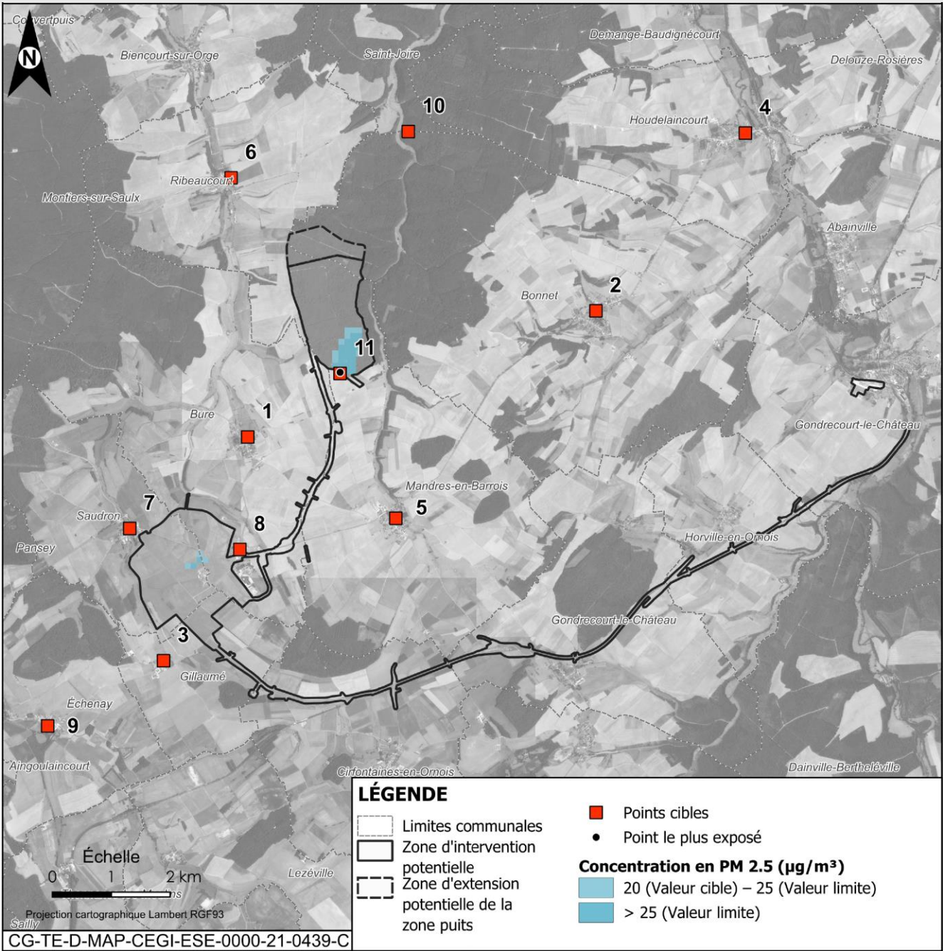
Figure 2-11 Concentration en PM2,5 ( \mu\text{g}/\text{m}^3 ) en phase de construction initiale
