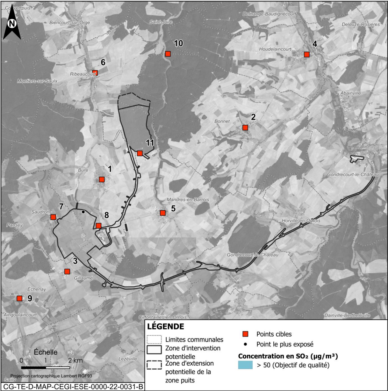
Figure 2-9 Concentration en SO 2 (µg/m 3 ) en phase de construction initiale
