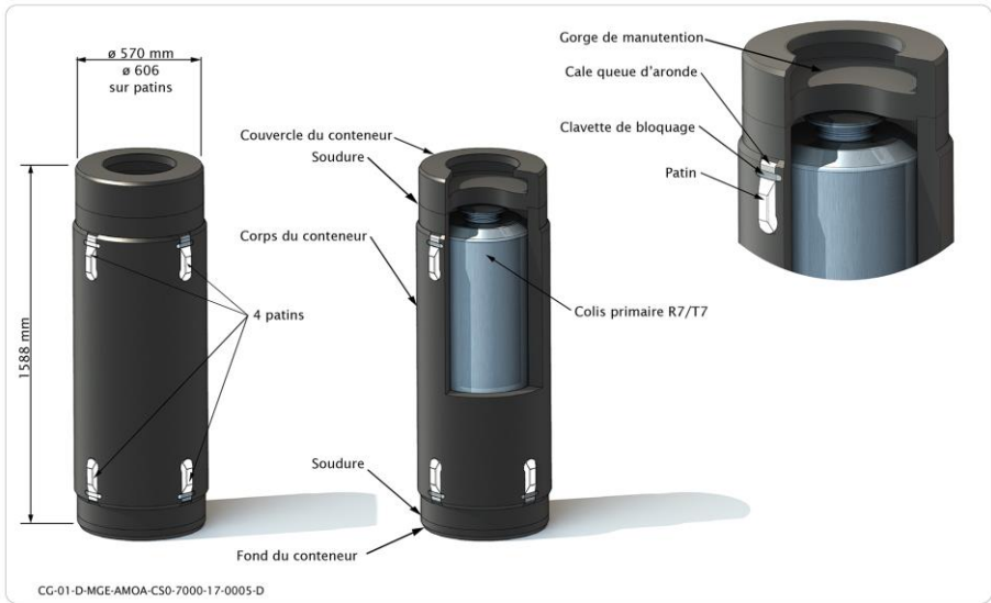
Figure 4-2 Illustration d'un colis de stockage des déchets vitrifiés avec son conteneur de stockage
