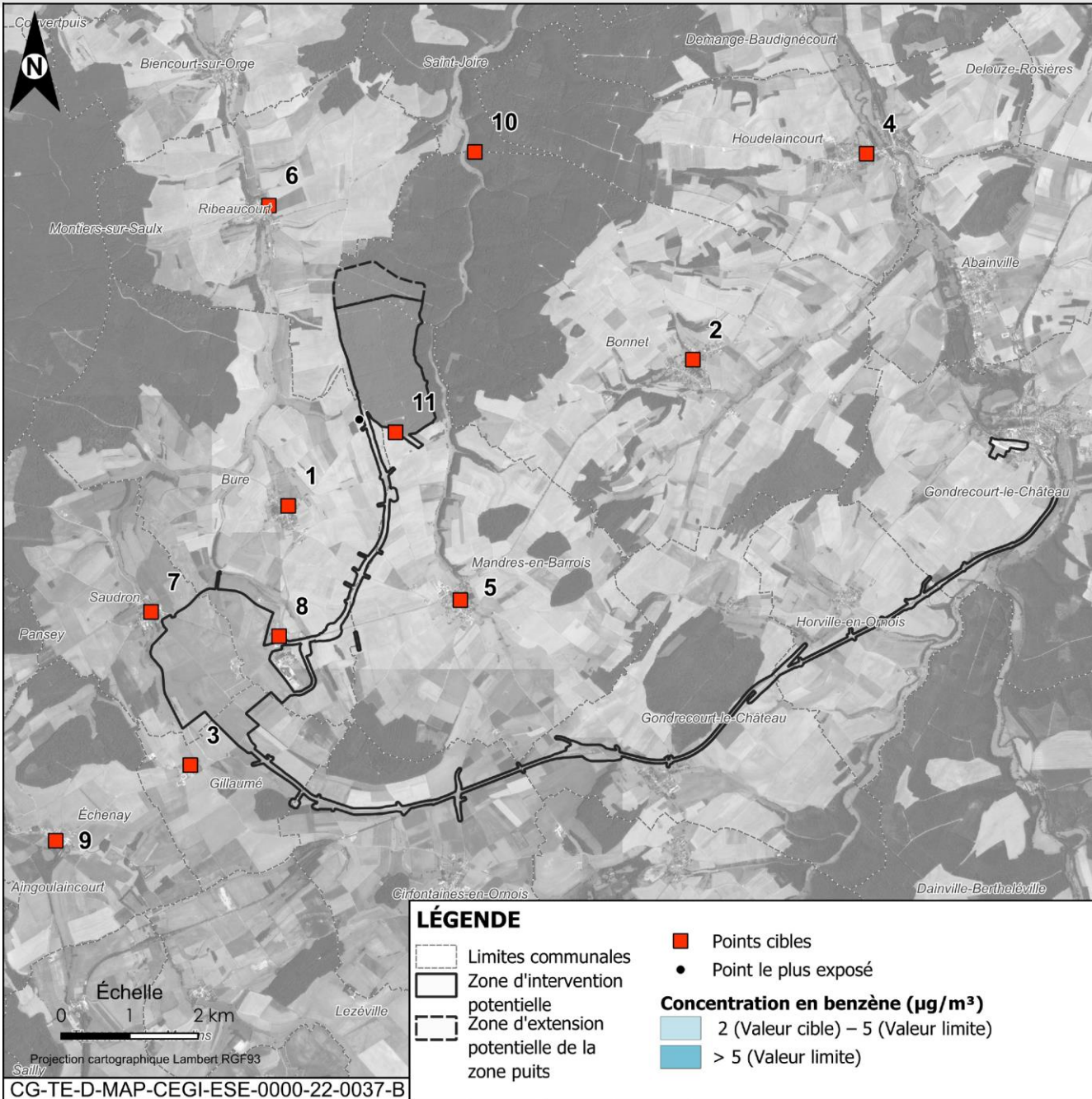
Figure 2-17 Concentration en benzène ( \mu\text{g}/\text{m}^3 ) en phase de fonctionnement
