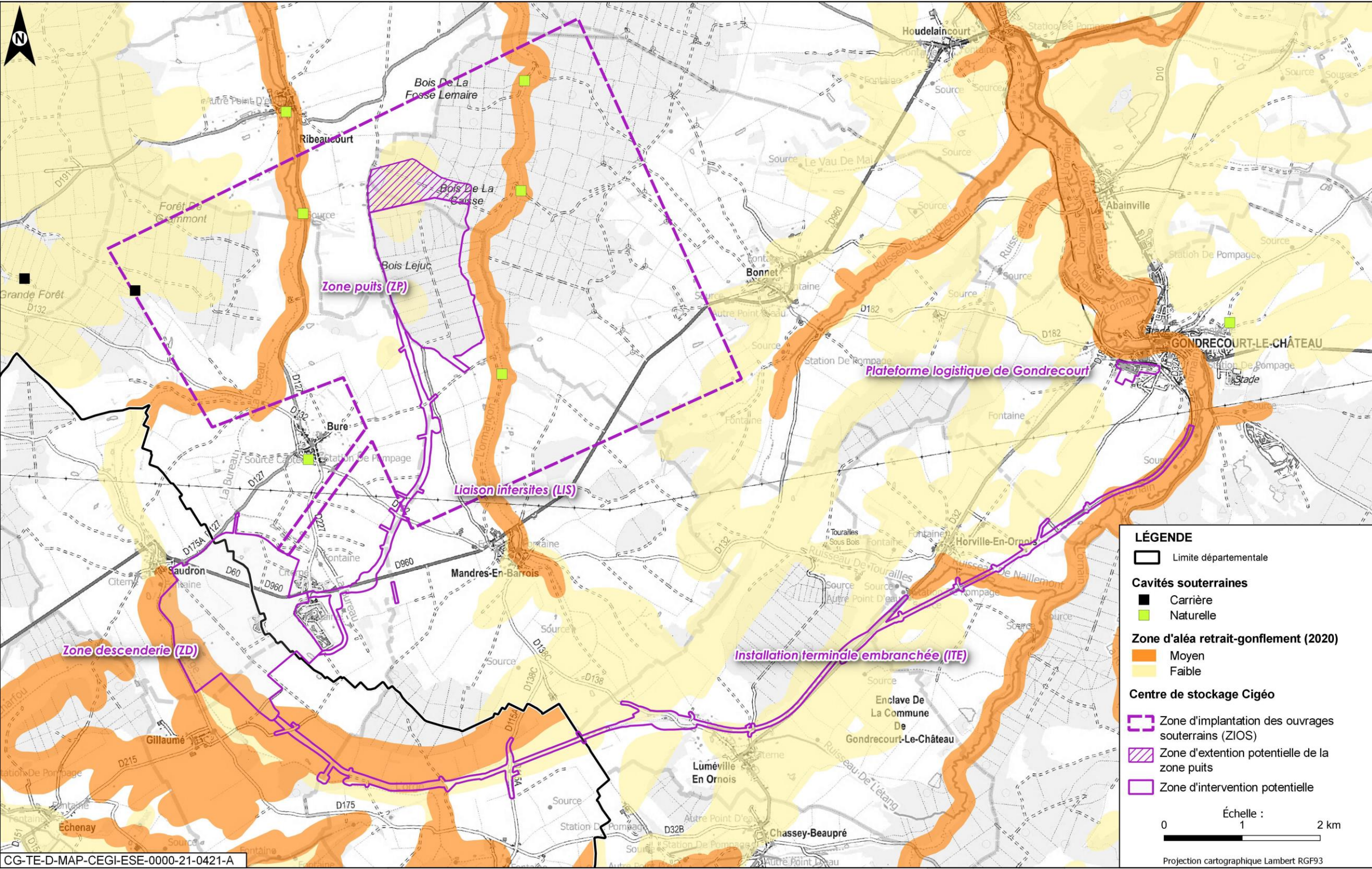
Figure 4-8 Risque de mouvements de terrain – zoom sur le centre de stockage Cigéo
