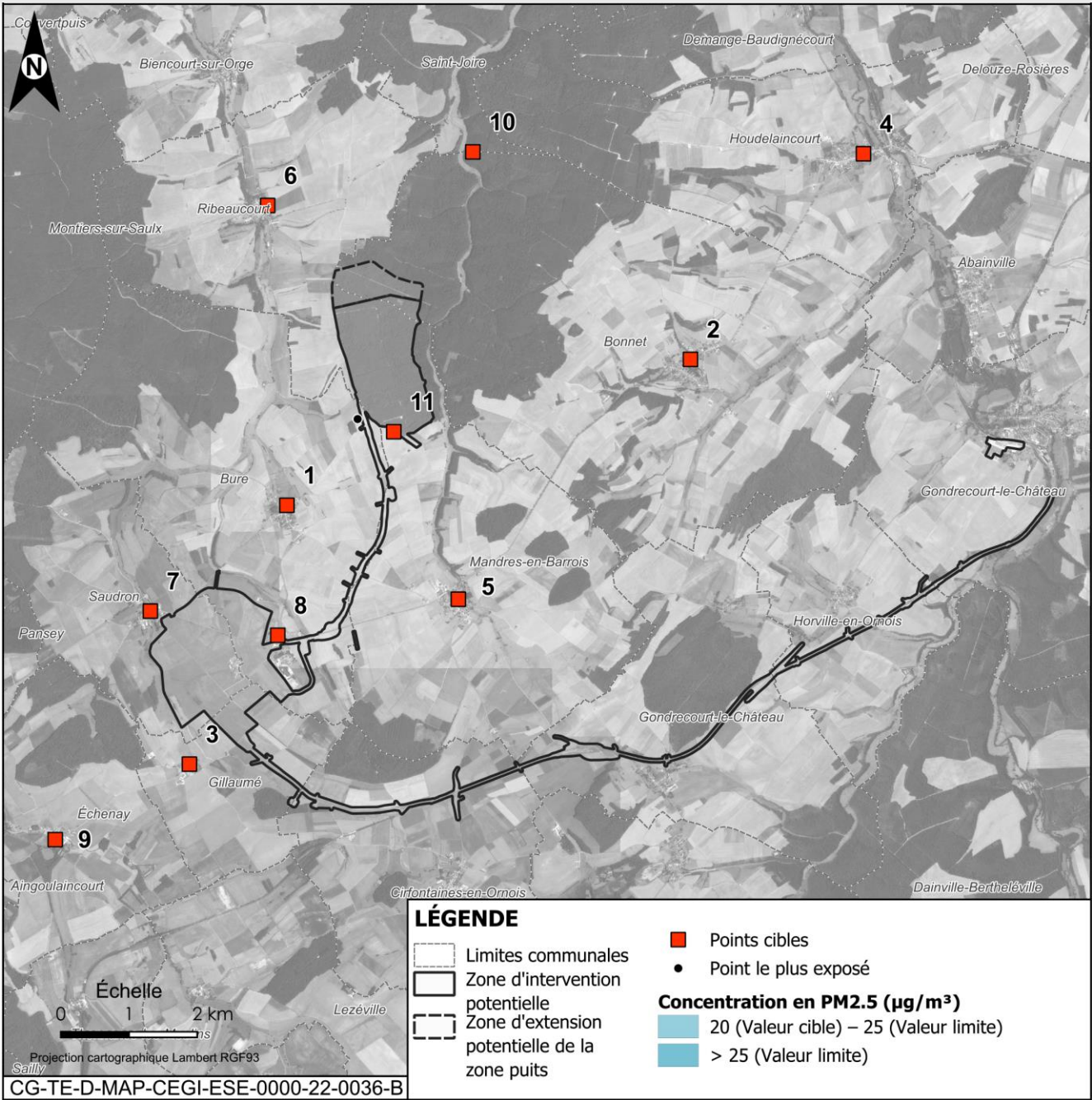
Figure 2-16 Concentration en PM2,5 ( \mu\text{g}/\text{m}^3 ) en phase de fonctionnement
