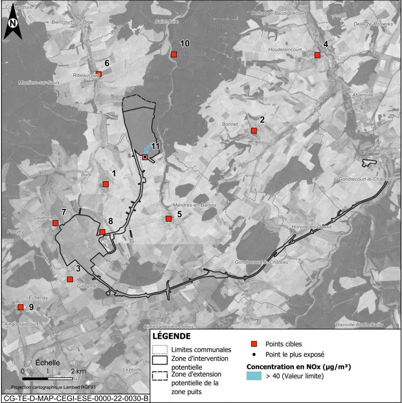
Figure 2-8 Concentration en Nox ( \mu\text{g}/\text{m}^3 ) en phase de construction initiale
