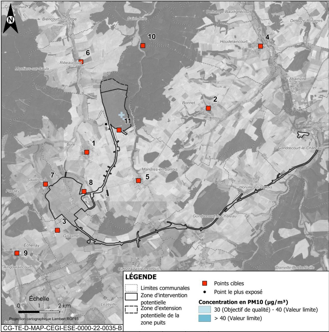
Figure 2-15 Concentration en PM10 (µg/m 3 ) en phase de fonctionnement
