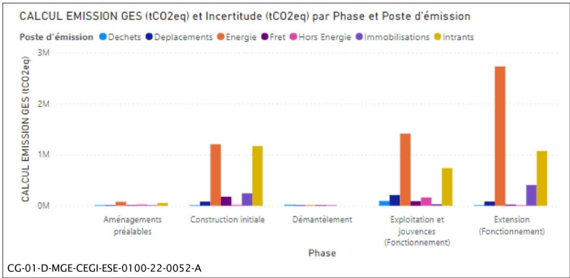
Figure 2-5 Émissions de gaz à effet de serre par phases opérationnelles et postes d’émission
