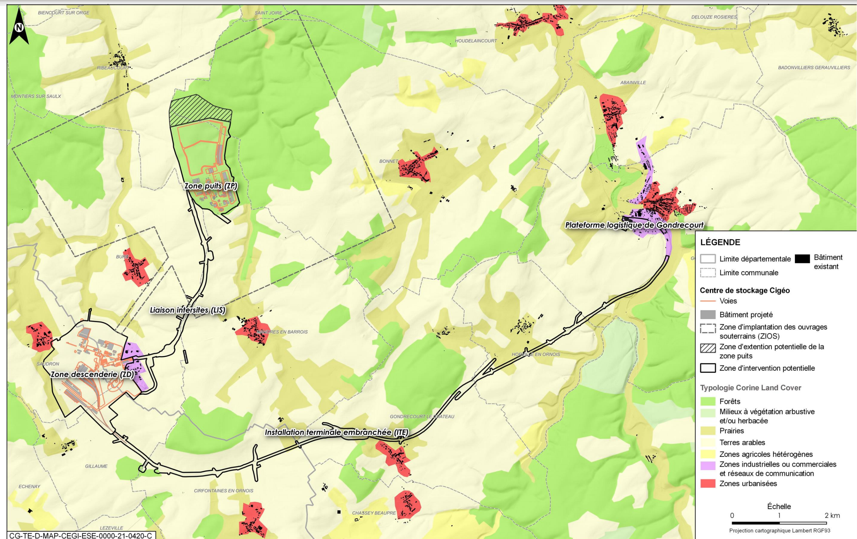
Figure 3-3 Occupation du sol au sein du projet global Cigéo - zoom sur le centre de stockage
