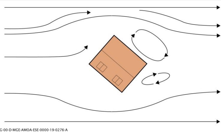
Figure 2-3 Obstacle à l'écoulement du vent, représentation du phénomène de turbulence
