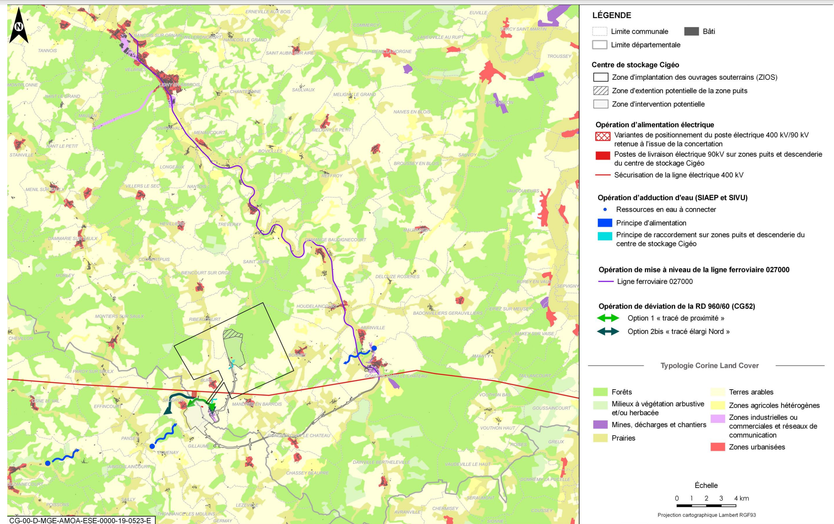
Figure 3-2 Occupation du sol au sein du projet global Cigéo
