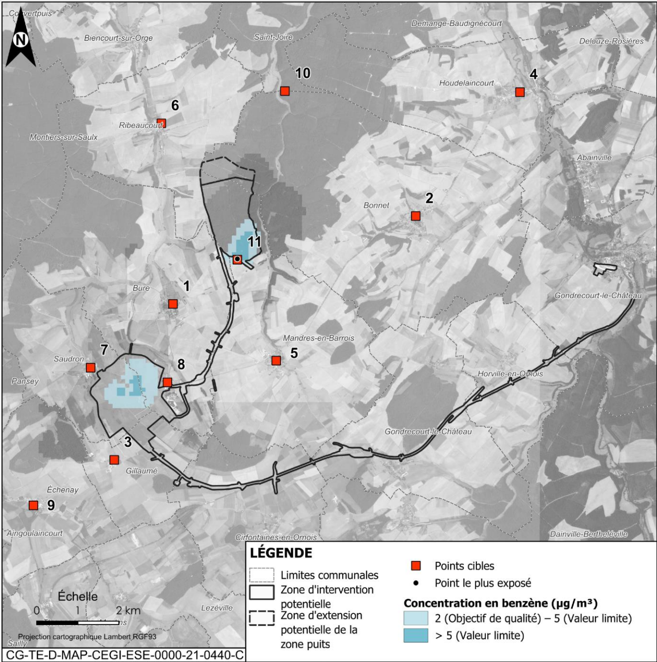
Figure 2-12 Concentration en benzène ( \mu\text{g}/\text{m}^3 ) en phase de construction initiale
