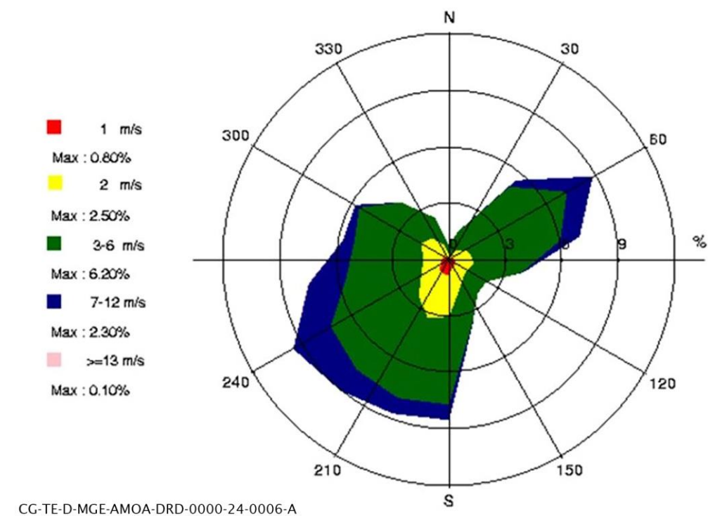
Figure 2-19 Rose des vents à la station atmosphérique d'Houdelaincourt
