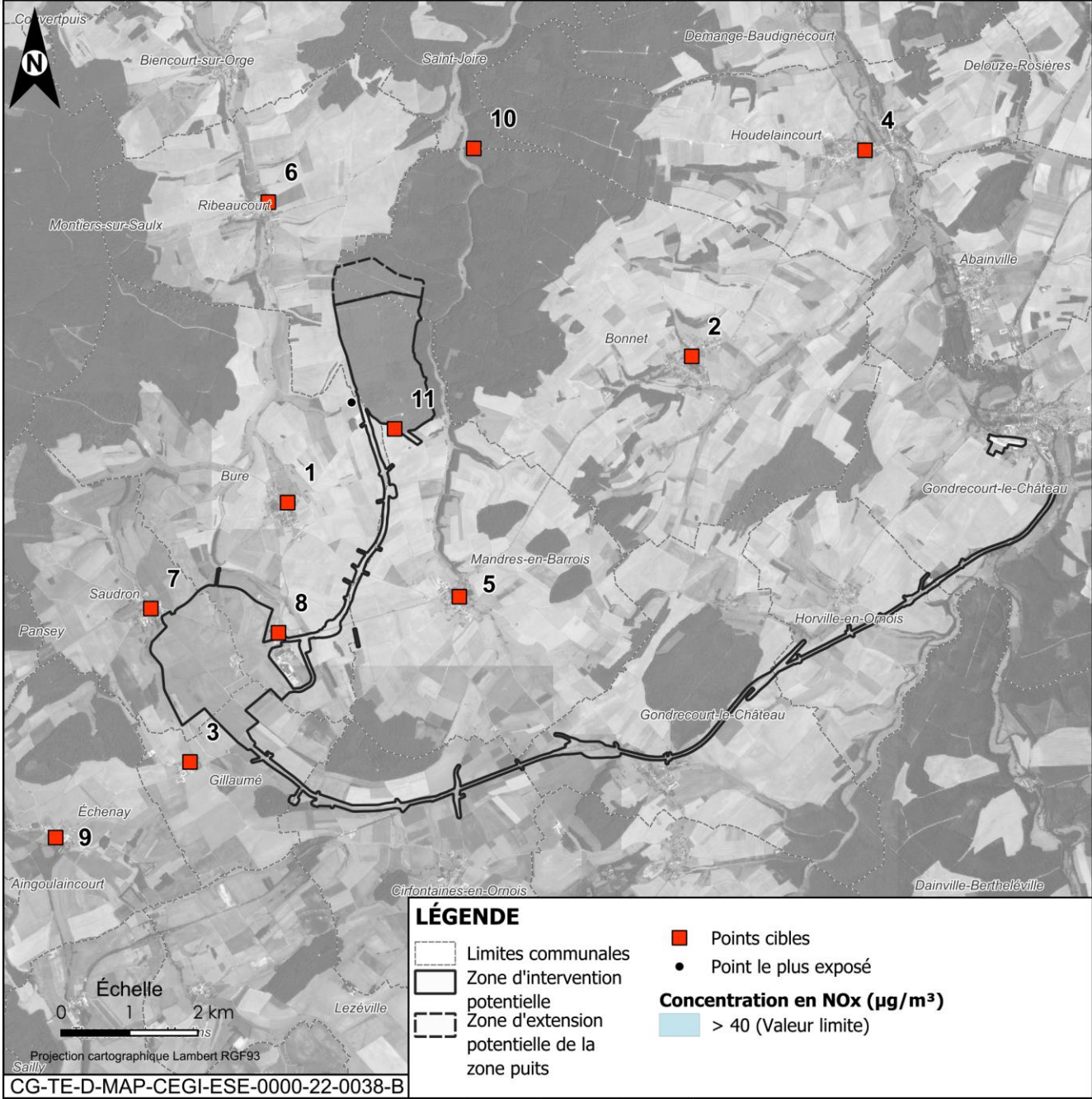
Figure 2-13 Concentration en Nox (µg/m³) en phase de fonctionnement
