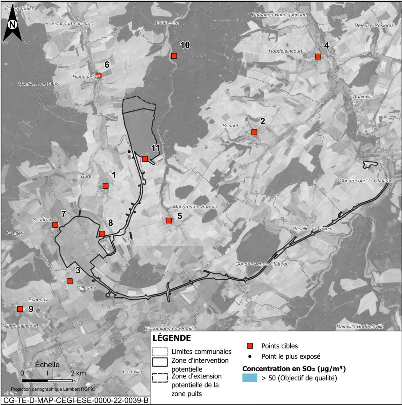
Figure 2-14 Concentration en SO 2 (µg/m 3 ) en phase de fonctionnement
