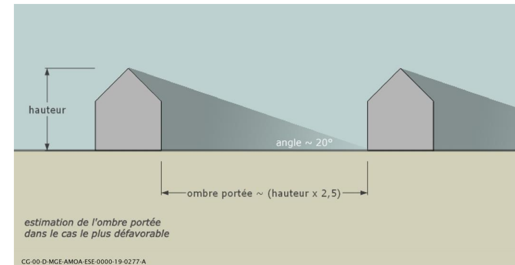
Figure 2-4 Représentation schématique du phénomène d'ombre portée
