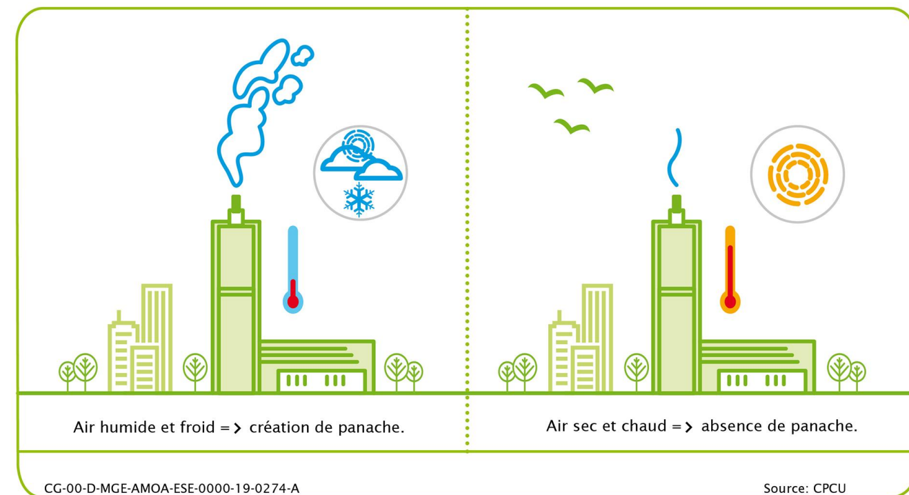
Figure 2-1 Variation du panache de fumée selon les conditions météorologiques
