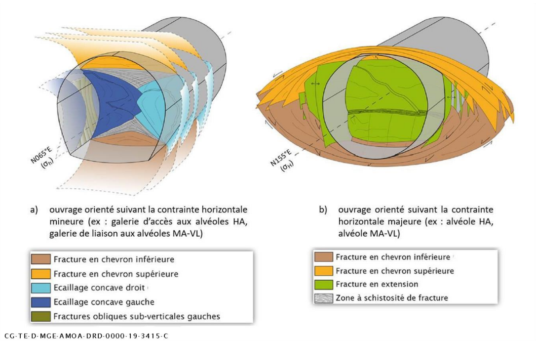
Figure 4-6 Représentation de la fracturation induite autour des ouvrages suivant leurs orientations par rapport à la contrainte horizontale mineure (gauche) et majeure (droite)
