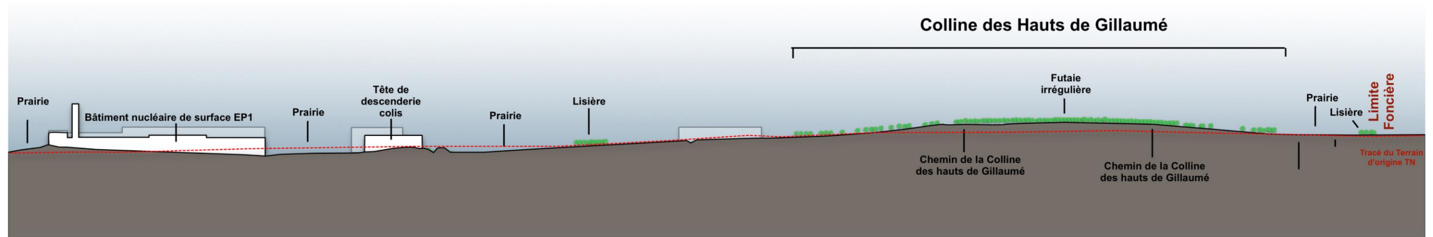
Figure 14-74 Coupe n° 3 : zone descendante dans un axe entre le bâtiment nucléaire de surface EP1 et la butte de Gillaumé à l'est.
