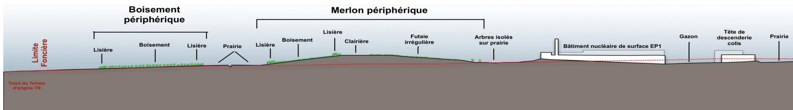
Figure 14-73 Coupe n° 2 : zone descendrière dans un axe reliant la limite foncière nord-ouest côté Saudron et le bâtiment nucléaire de surface EP1
