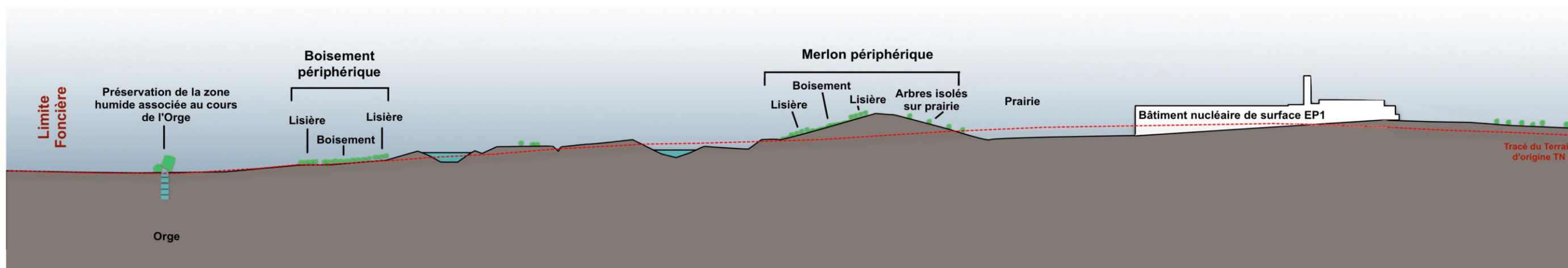
Figure 14-72 Coupe n° 1 : zone descendrière dans un axe reliant la zone humide associée aux cours de l'Orge et le bâtiment nucléaire de surface EP1
