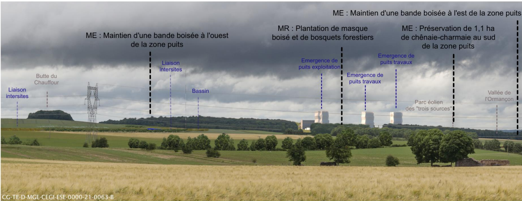
Figure 14-62 Mesures de réduction (MR) en phase de fonctionnement depuis le point de vue 19b (zoom) (mesures plantées matures)
