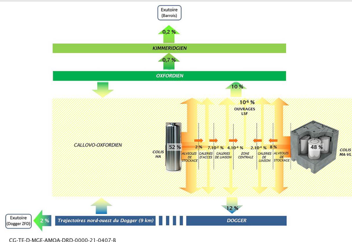
Figure 5-10 Scénario d'évolution normale – situation de référence, quartiers de stockage HA et MA-VL, iode 129 : bilan (%) de la répartition des voies de transfert dans les composants ouvragés et le milieu géologique depuis les colis jusqu'aux exutoires à million d'années par rapport à l'inventaire total initial (HA + MA-VL)
