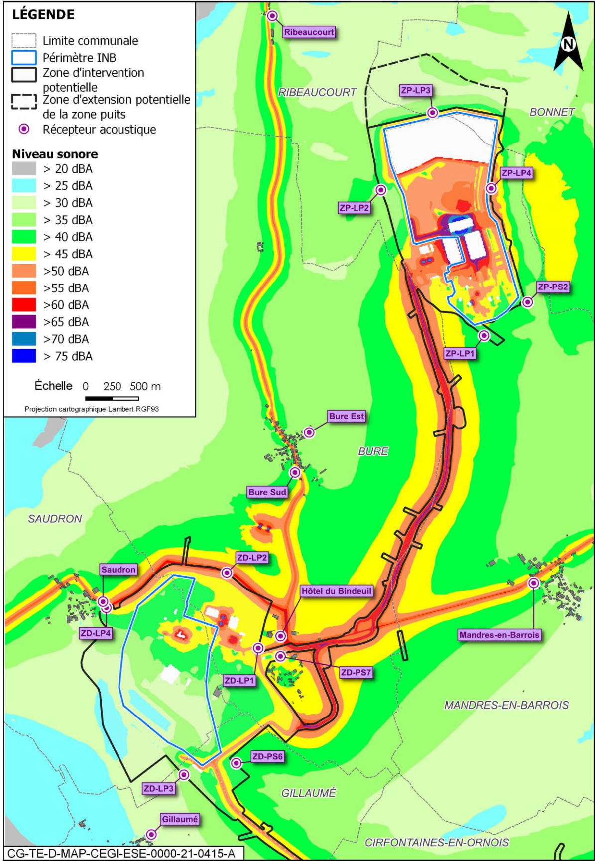
Figure 2-6 Propagation acoustique - Fonctionnement - Toutes sources du projet global Cigéo (diurne)
