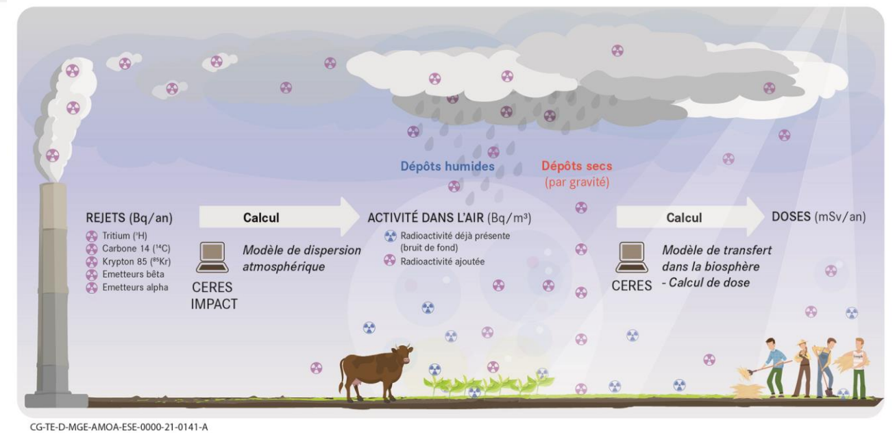
Figure 4-11 Schéma présentant les modèles et codes utilisés pour la dispersion atmosphérique et les calculs de dose
