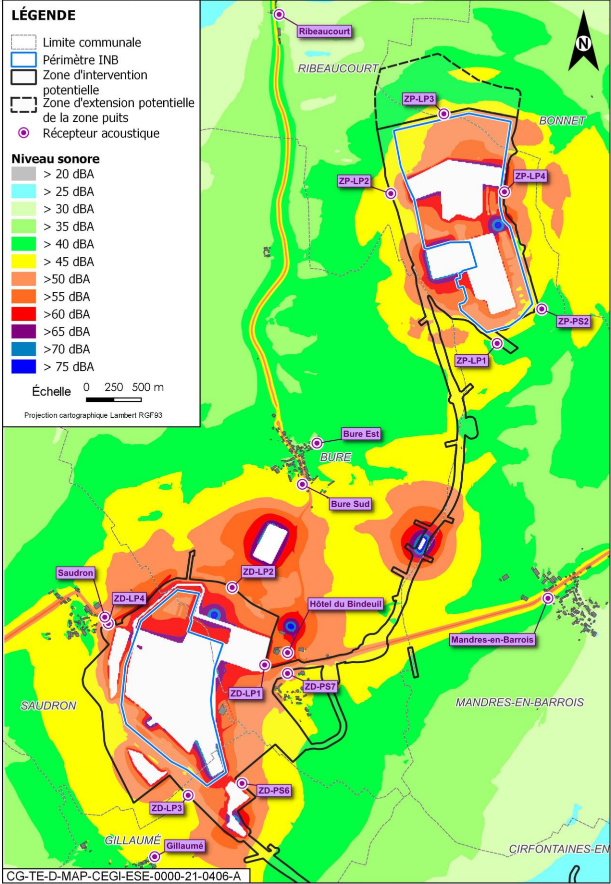
Figure 2-3 Propagation acoustique - Aménagements préalables - Toutes sources (Diurne)
