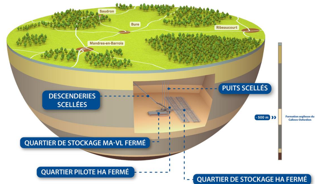
Figure 5-2 Illustration schématisée du centre de stockage après sa fermeture définitive
