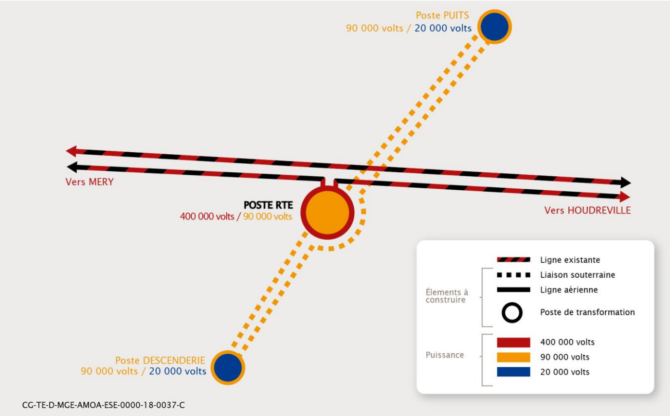
Figure 2-9 Illustration des opérations de raccordement sur la ligne électrique 400 kV 5
