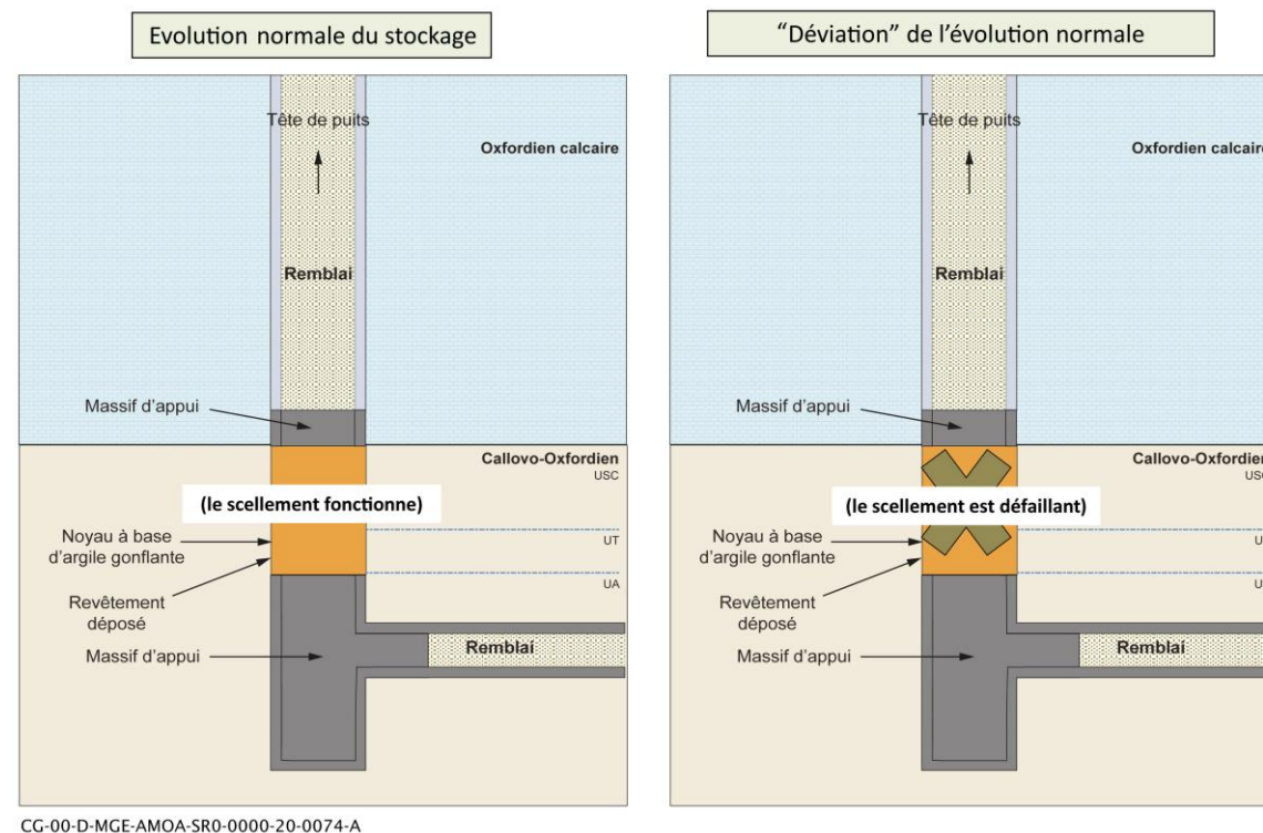
Figure 5-6 Illustration montrant la différence entre l'évolution normale et une situation possible de défaillance de scellement pouvant induire une "déviation" de l'évolution normale
