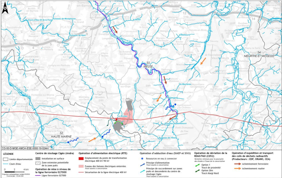
Figure 3-2 Localisation du groupe de référence situé à Bure et des ruisseaux de l'Orge, de La Bureau et de l'Ormançon
