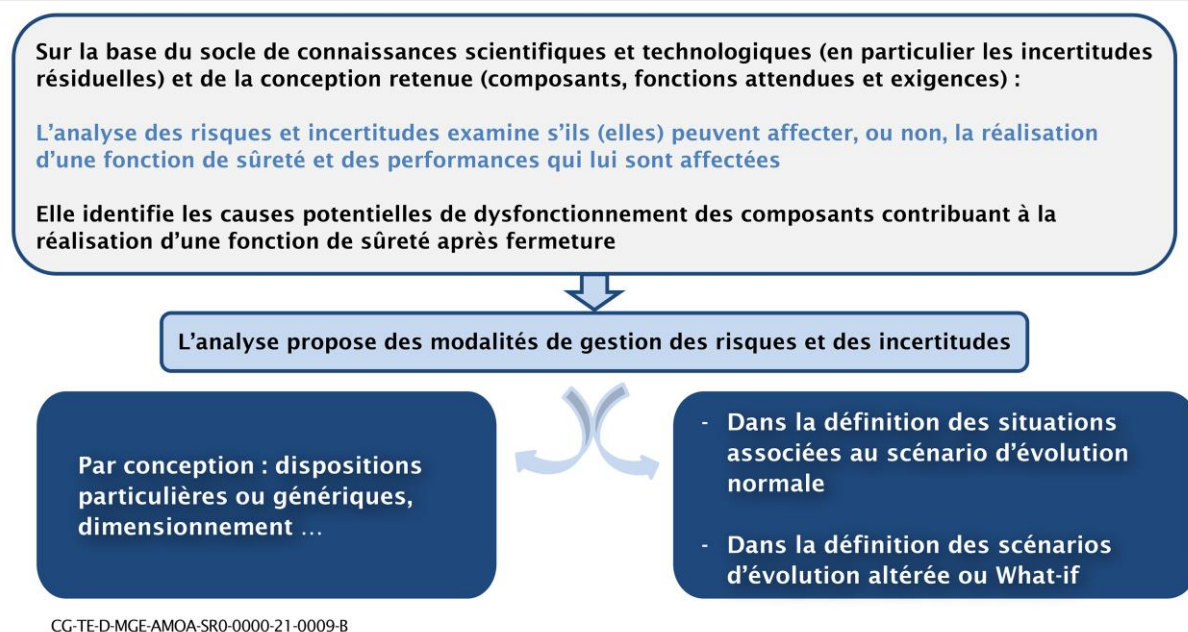
Figure 8-4 Schéma illustratif du déroulement de l'analyse des risques et incertitudes après fermeture
