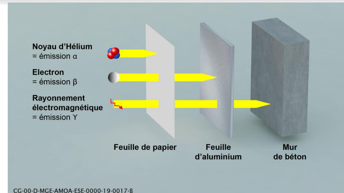
Figure 4-1 Illustration des trois types de rayonnements ionisants
