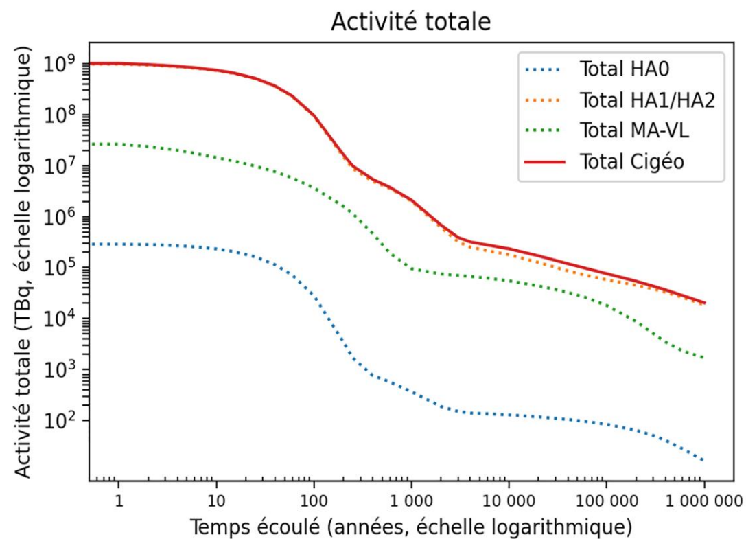
Figure 5-1 Illustration de la décroissance dans le temps de la radioactivité totale des déchets de l'inventaire de référence de l'INB Cigéo (courbe rouge) et de la radioactivité de l'inventaire total des colis de déchets HA0, HA1/HA2 et MA-VL (courbes pointillées)
