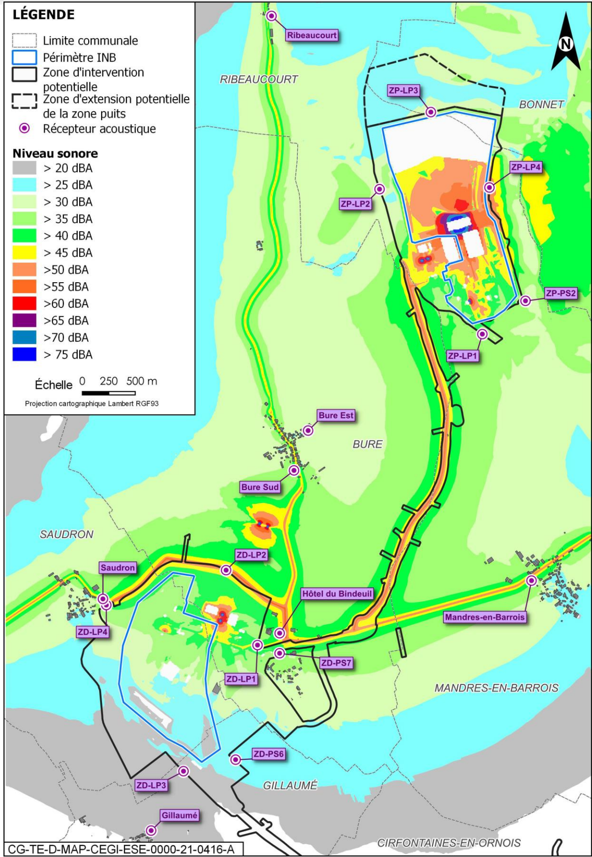
Figure 2-7 Propagation acoustique - Fonctionnement - Toutes sources du projet global Cigéo (nocturne)
