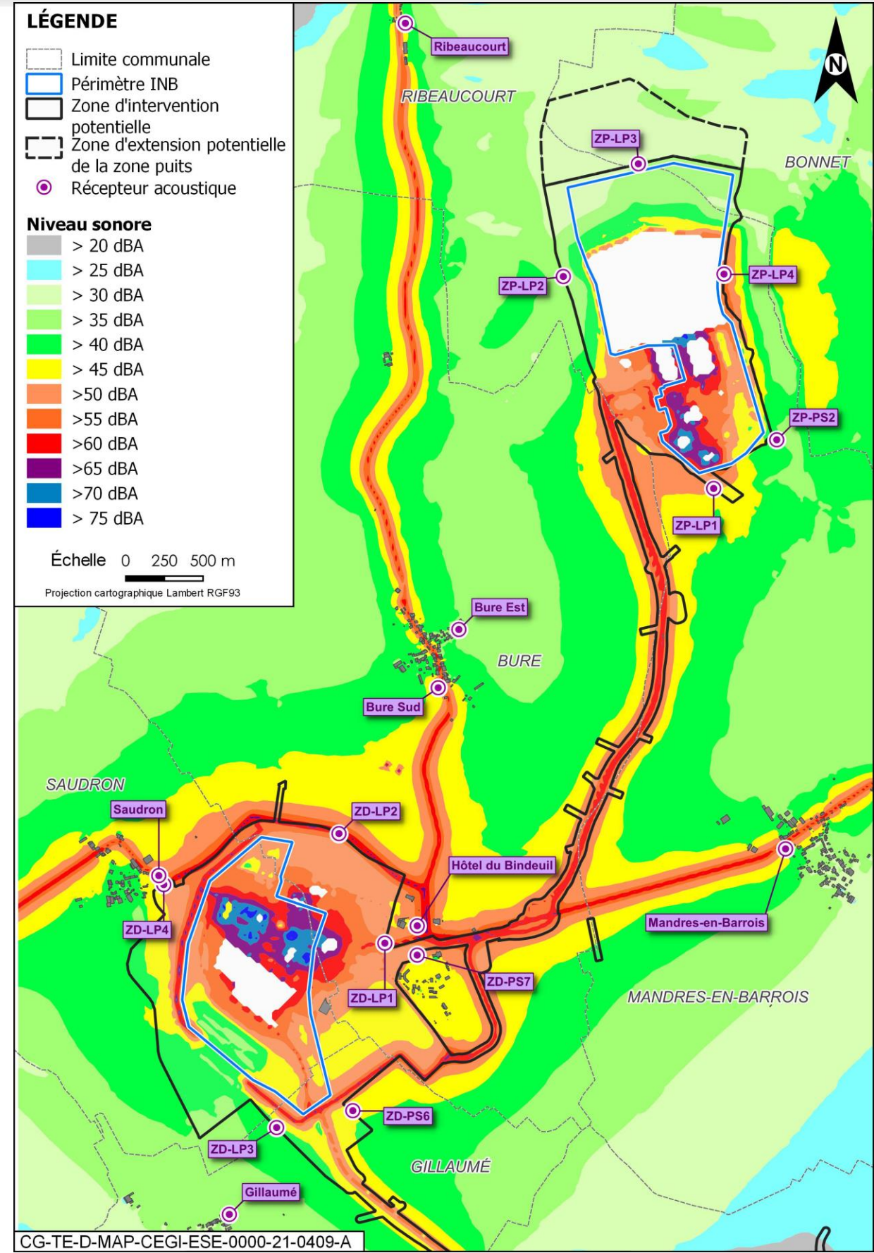
Figure 2-4 Propagation acoustique - Construction initiale - Toutes sources (diurne)
