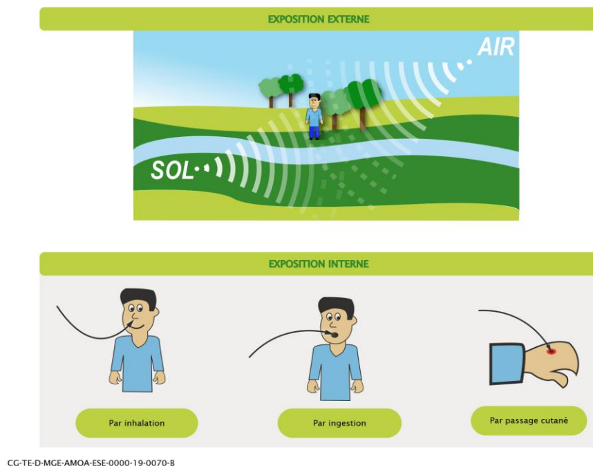
Figure 4-3 Illustration des types d'exposition à la radioactivité
