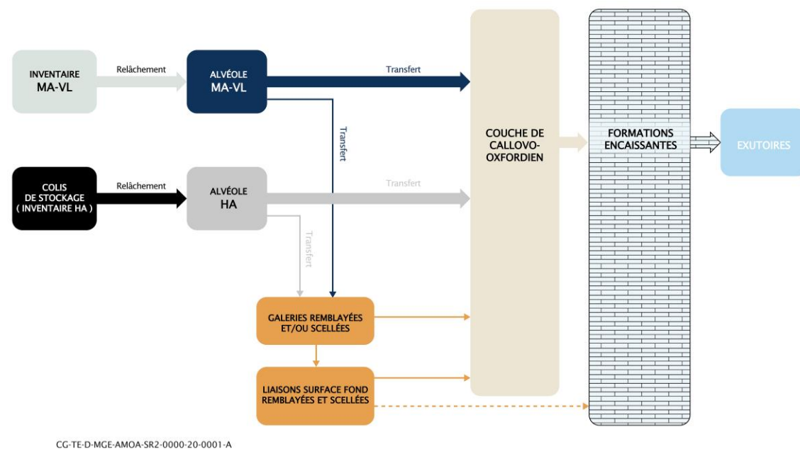
Figure 5-5 Schéma illustratif des composants et des voies de transfert potentielles pris en compte pour du scénario d'évolution normale
