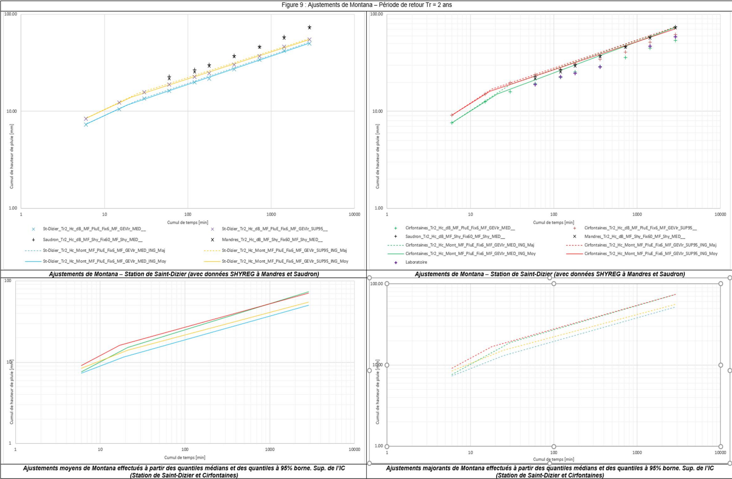
Figure Annexe 3-1 Ajustements de Montana – Période de retour Tr = 2 ans
