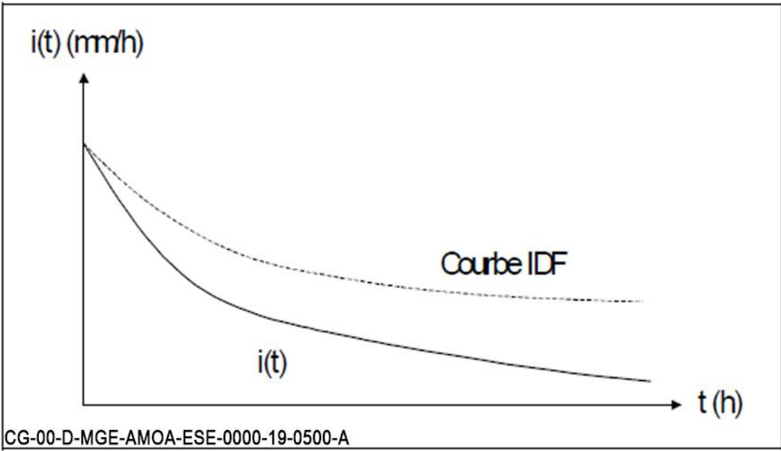
Figure Annexe 4-1 Hyétogramme instantanée « Keifer » obtenu à partir de la courbe Intensité-Durée-Fréquence associée
