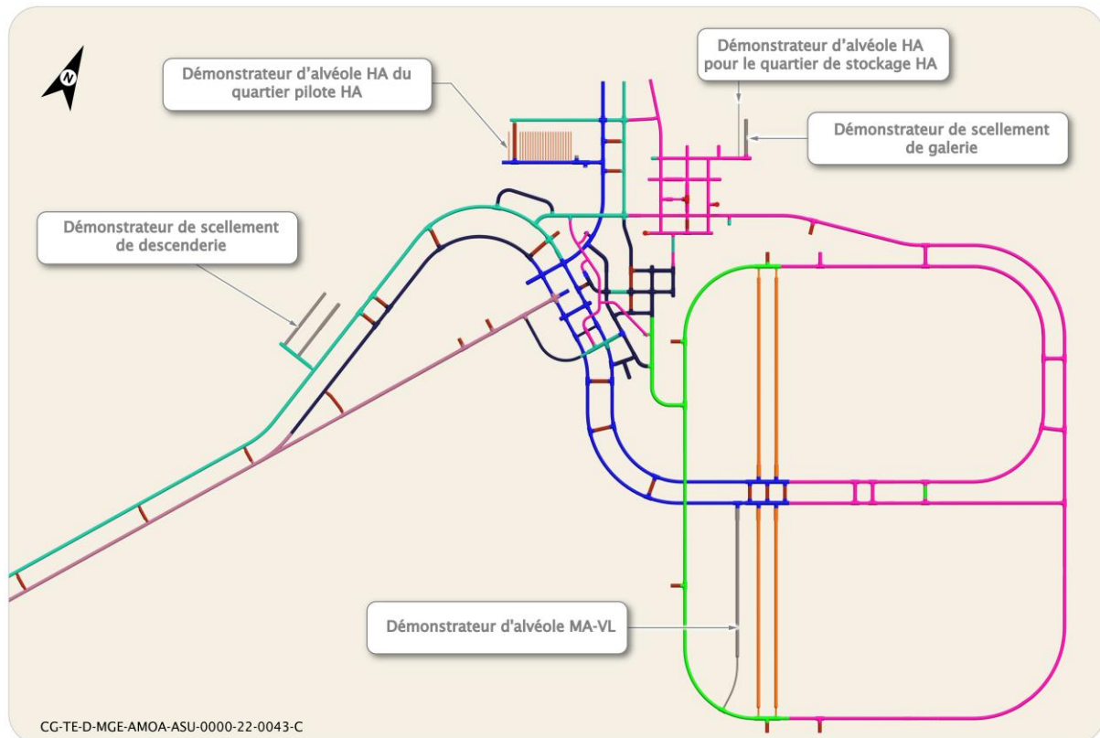
Figure 1-5 Illustration des démonstrateurs mis en place pendant la construction initiale (en tranche 1)
