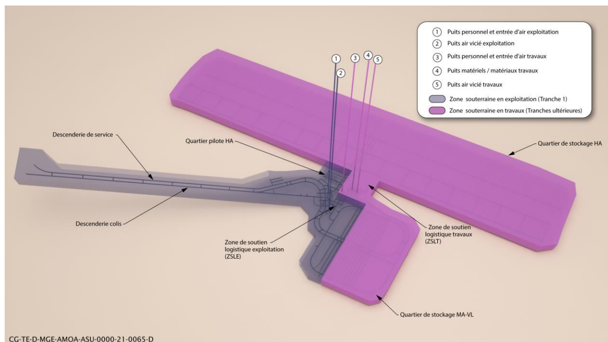
Figure 2-2 Illustration de principe de séparation des zones souterraines en exploitation et en travaux et les liaisons surface-fond associées (dimensions et proportions non représentatives)
