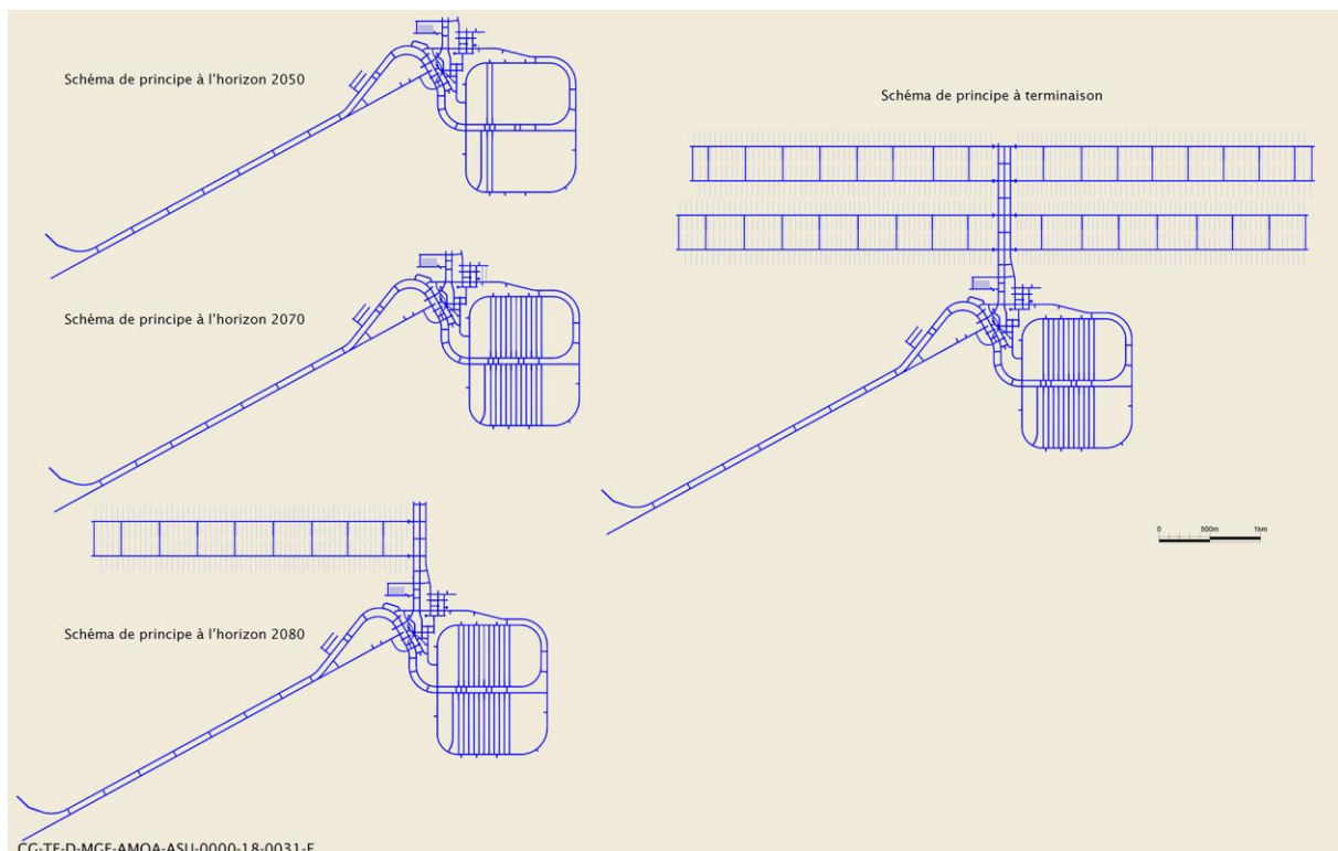
Figure 1-6 Principe de déploiement de l'installation souterraine
