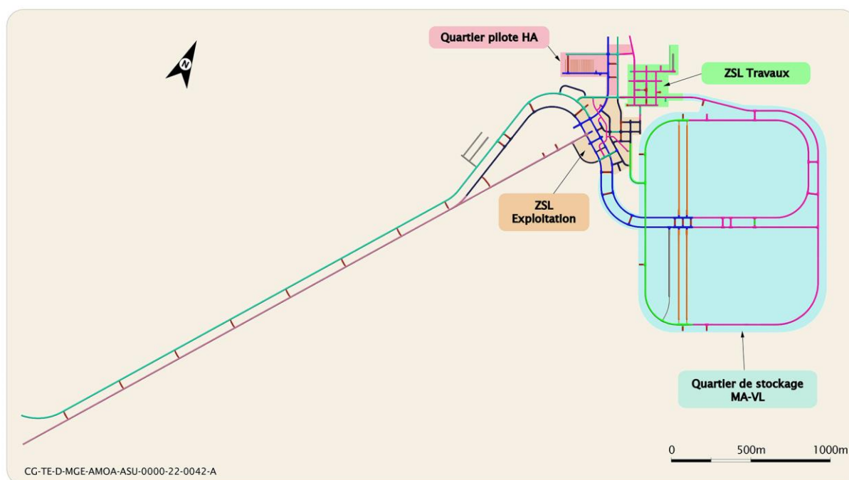
Figure 1-3 Illustration des ouvrages souterrains construits lors de la phase de construction initiale (en tranche 1)
