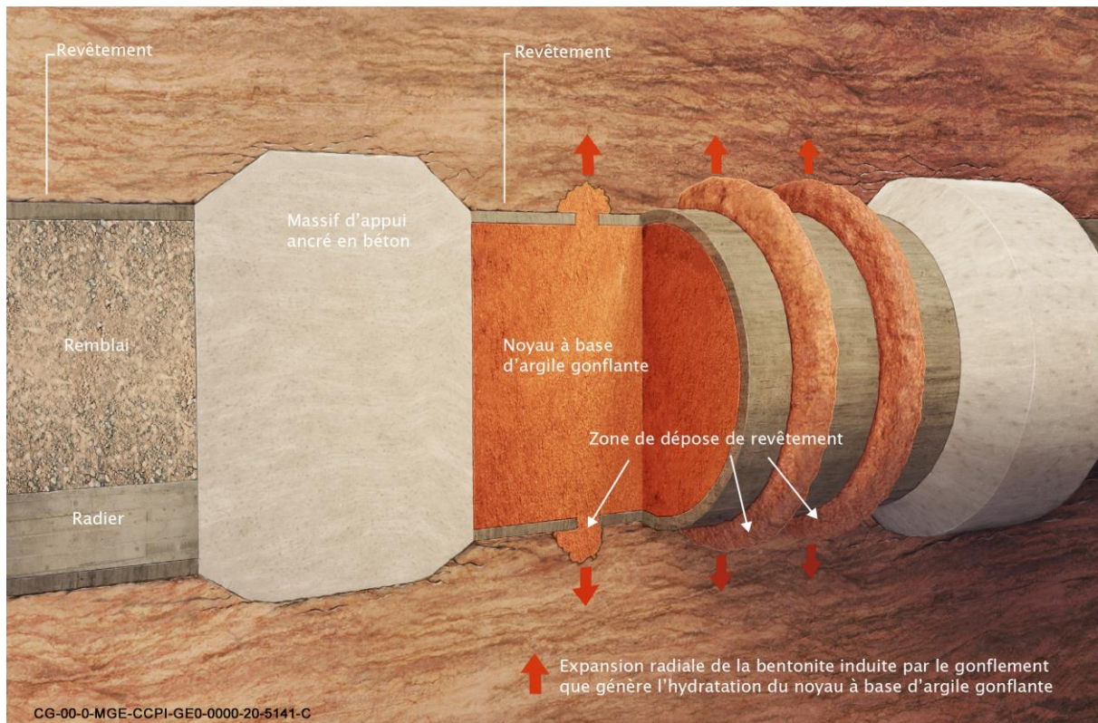
Figure 3-2 Schéma de principe illustratif d'un scellement de galerie (solution technique de référence avec massifs d'appui en béton ancrés dans la roche)
