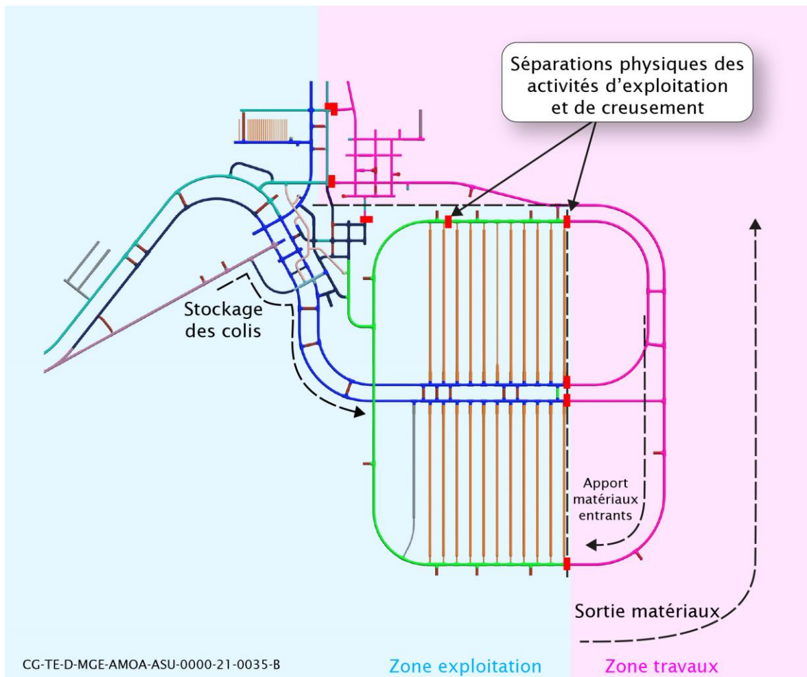
Figure 2-3 Illustration des interfaces entre les zones en exploitation et en travaux - Quartier de stockage MA-VL
