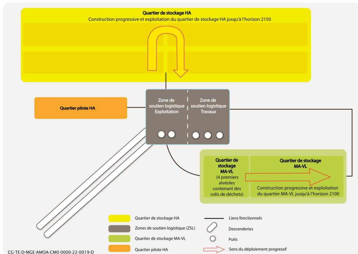
Figure 1-2 Schéma simplifié du déploiement prévisionnel de l'installation souterraine
