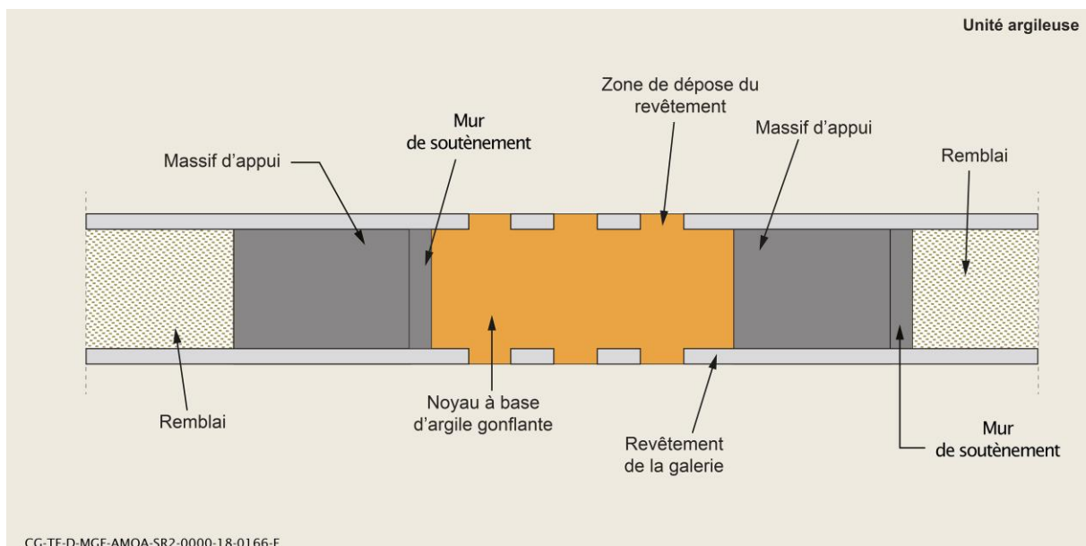
Figure 3-3 Schéma de principe d'un scellement horizontal avec confinement du noyau par frottement des massifs d'appui en béton non ancrés dans la roche et du remblai, retenu en piste d'optimisation
