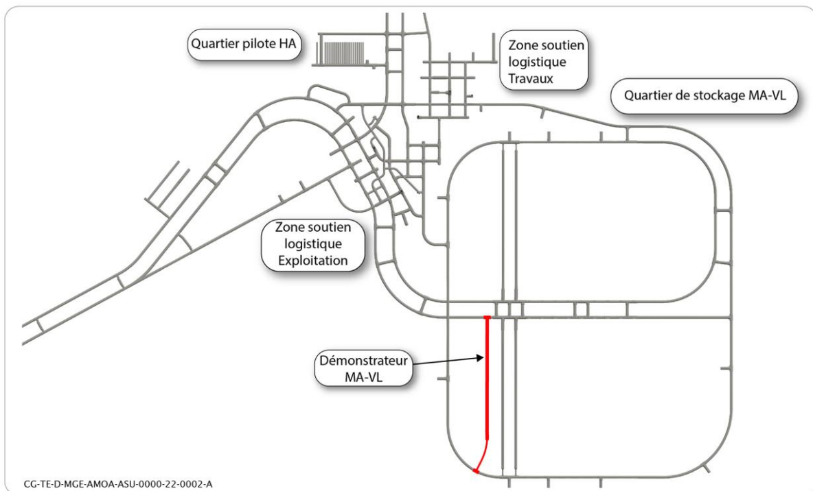
Figure 3-1 Illustration de la localisation du démonstrateur de constructibilité d'un alvéole MA-VL réalisé en tranche 1 dans le quartier de stockage MA-VL
