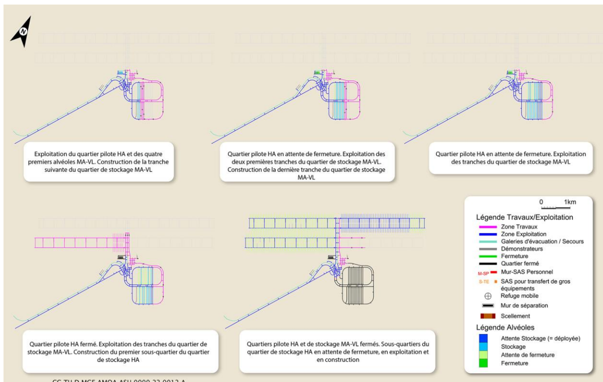
Figure 1-7 Illustration du développement progressif des ouvrages souterrains de l'installation souterraine
