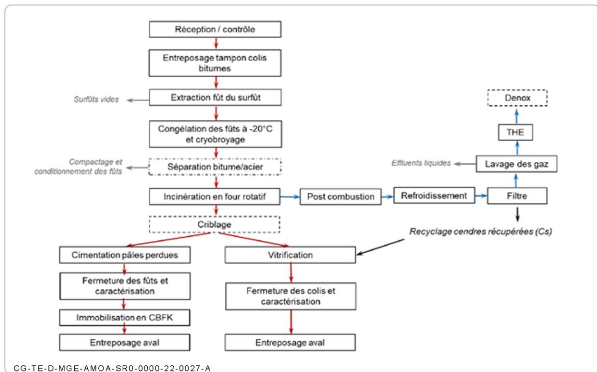
Figure Annexe 2-2 Diagramme fonctionnel du procédé de la filière 2 de traitement des déchets bitumés
