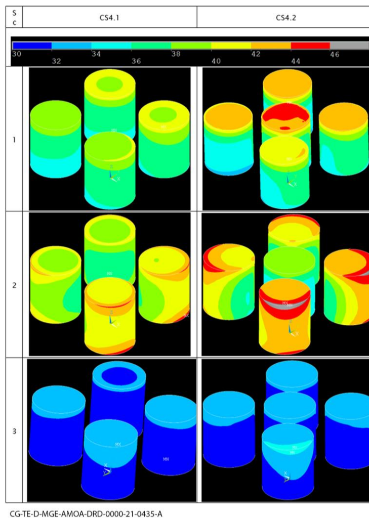
Figure 4-13 Illustration des champs de températures des colis de déchets bitumés soumis à différents scénarios d'incendie (scénario 1 = scénario court et scénario 2 = scénario long en cellule de manutention, scénario 3 en partie utile de l'alvéole)
