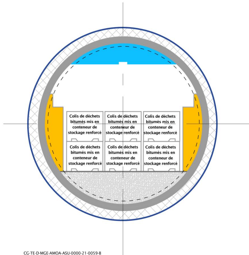
Figure 4-3 Illustration de la section de l'alvéole dédiée au stockage en l'état des colis de déchets bitumés et mis en conteneur renforcé vis-à-vis de l'incendie
