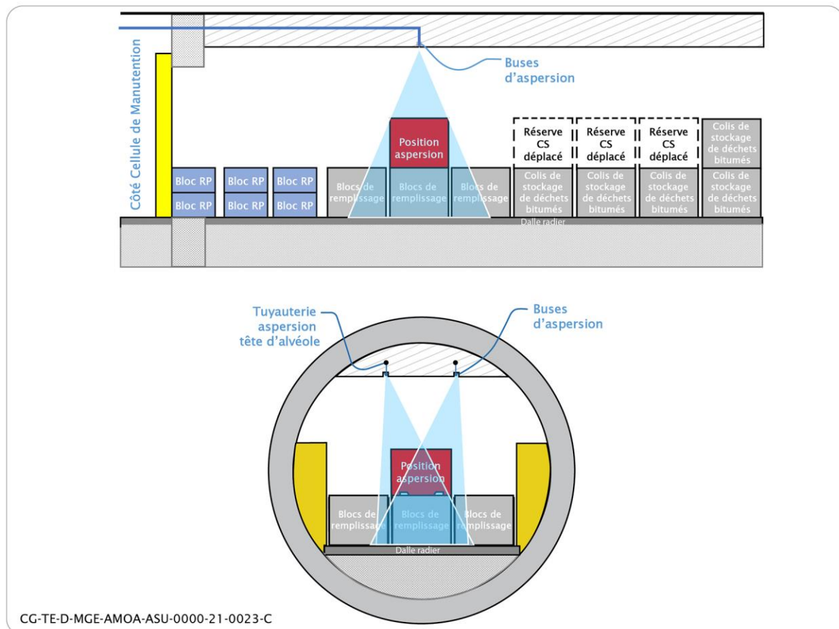
Figure 4-10 Schéma de principe d'implantation de la rampe d'aspersion d'eau dans la zone d'isolement, dans un alvéole dédié au stockage en l'état des colis de déchets bituminés et mis en conteneur renforcé vis-à-vis de l'incendie
