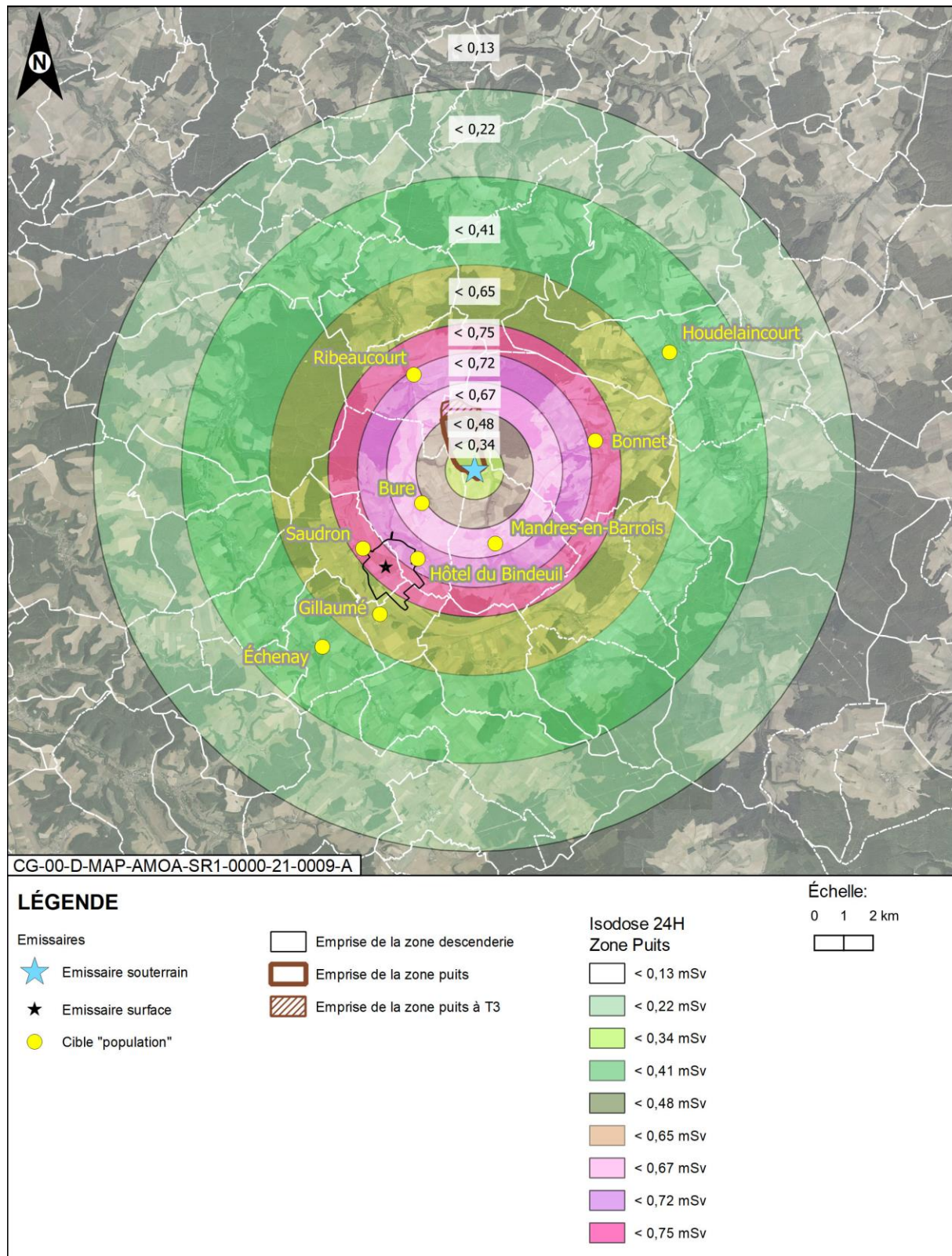
Figure Annexe 3-1 Doses maximales autour de la zone puits pour l'adulte pour une durée d'exposition de 24 heures, pour le scénario d'emballement postulé de déchets bitumés
