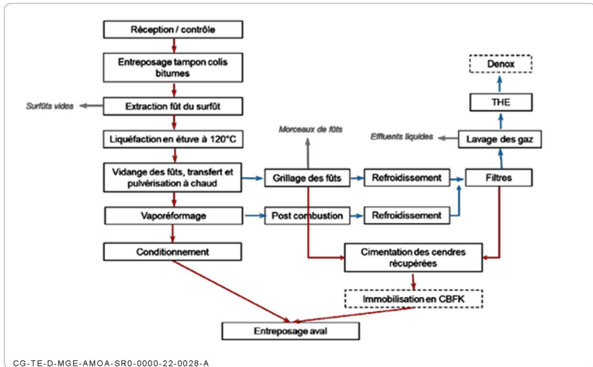
Figure Annexe 2-3 Diagramme fonctionnel du procédé de la filière 3 de traitement des déchets bitumés
