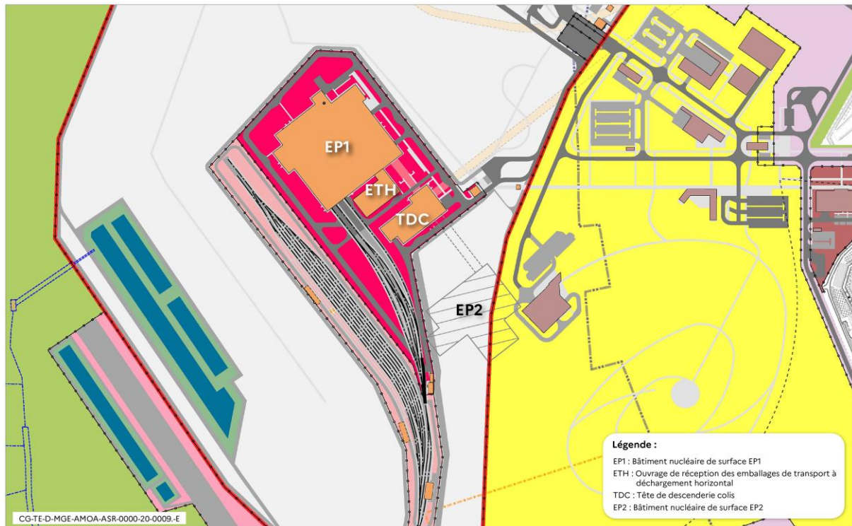
Figure 2-1 Illustration de l'implantation des ouvrages de surface et en particulier des futures constructions ET-H et EP1
