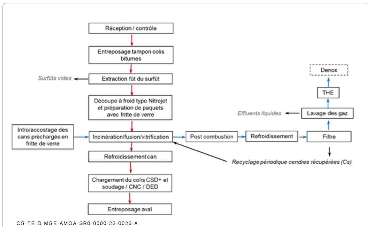
Figure Annexe 2-1 Diagramme fonctionnel du procédé de la filière 1 de traitement des déchets bitumés
