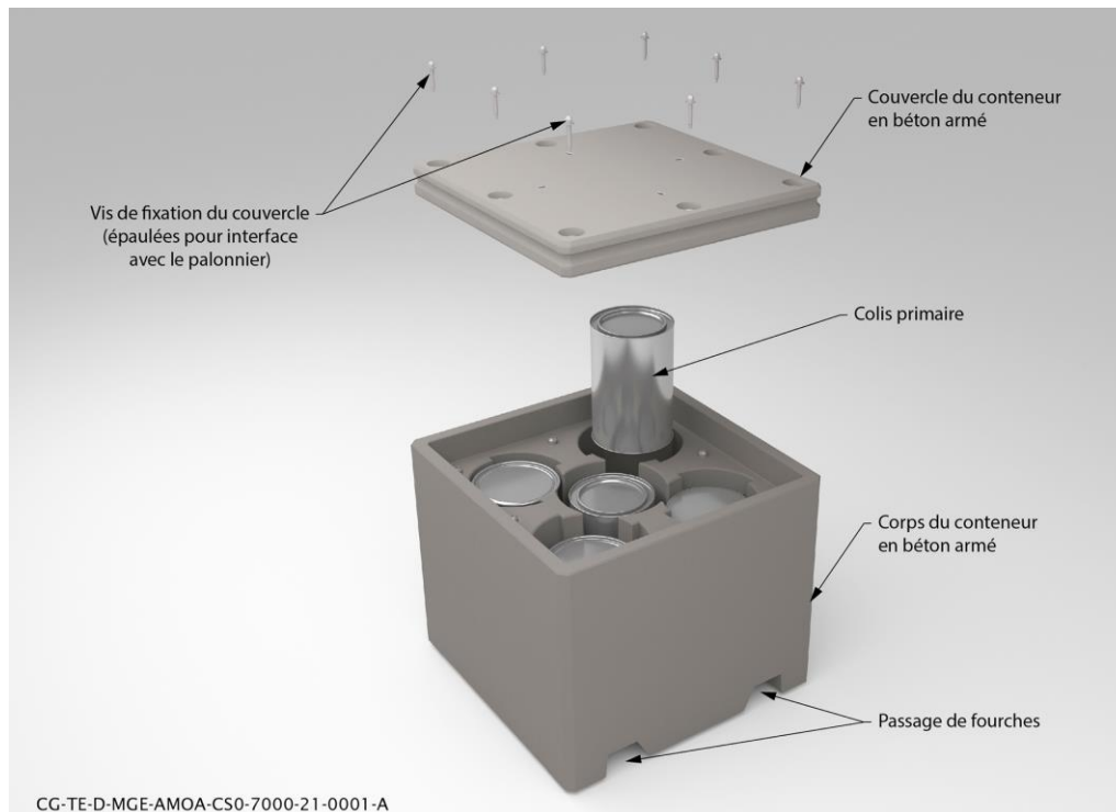
Figure 4-2 Schéma de principe d'un colis de stockage de déchets bitumés en l'état à cinq logements (CS4.2)
