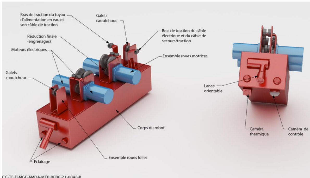
Figure 4-9 Schéma de principe du robot
