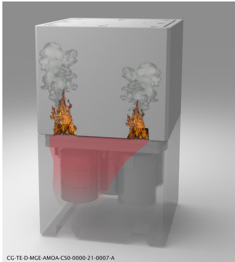
Figure 4-14 Illustration du scénario extrême d'emballement d'un colis de déchets bitumés dans un conteneur
