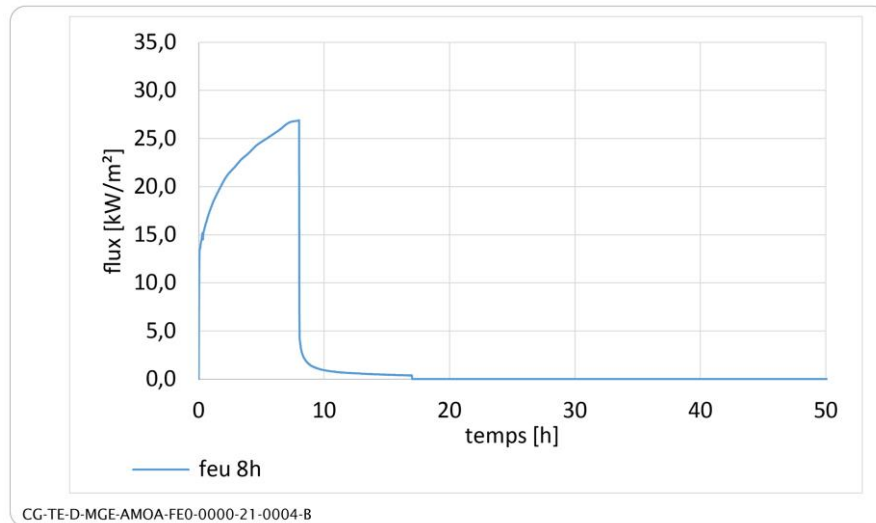
Figure 4-15 Courbe incendie maximale appliquée pendant huit heures sur le colis de déchets bitumés stockés en l'état, pour le scénario d'emballement postulé sur les colis adjacents
