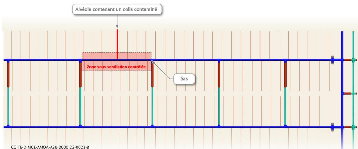
Figure 4-19 Schéma de principe du confinement d'un module pour le quartier de stockage HA
