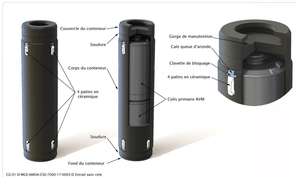
Figure 2-7 Schéma de principe d'un colis de stockage HA
