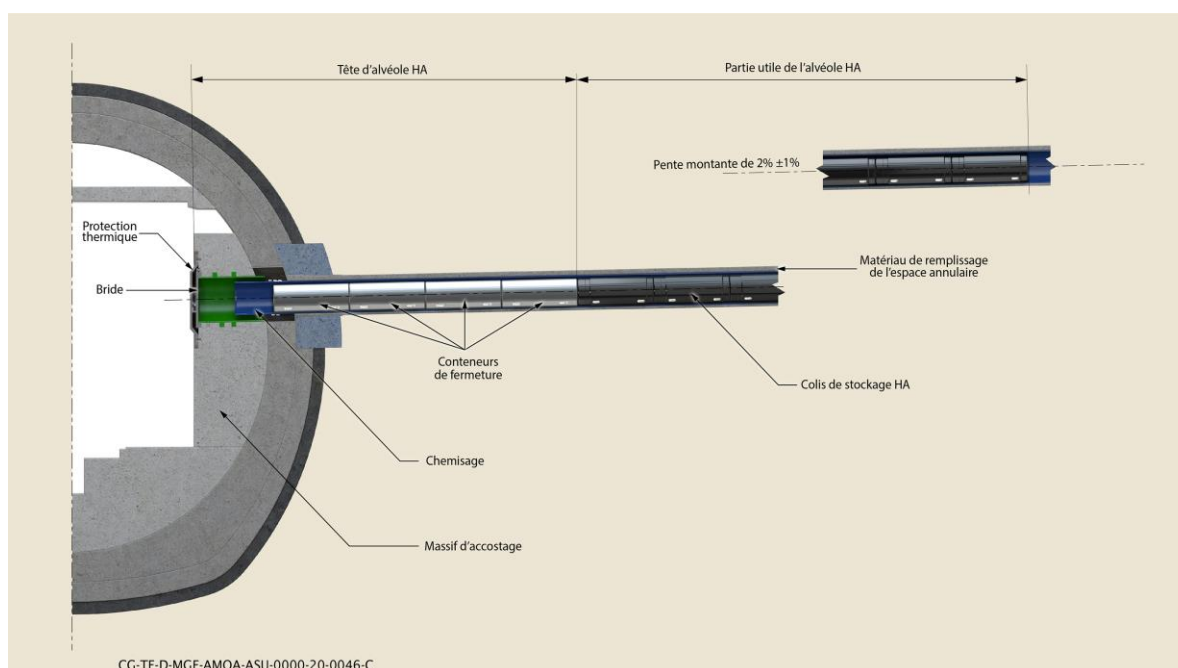
Figure 2-11 Schéma de principe d'un alvéole HA en attente de fermeture
