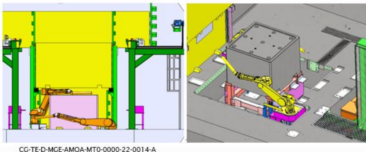
Figure 4-8 Schéma de principe du dispositif de contrôle de la contamination en cellule de manutention (colis MA-VL stocké en nappe Niveau 0 de la partie active)
