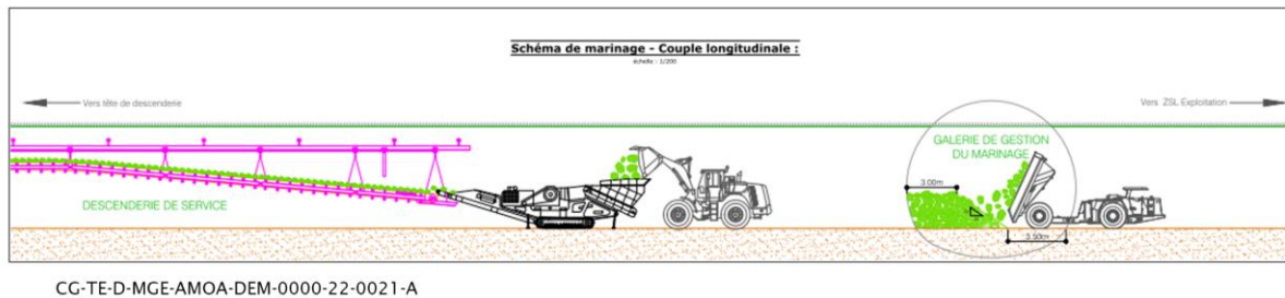
Figure 4-1 Schéma de principe du système de marinage combiné à une bande transporteuse pour évacuation des déblais
