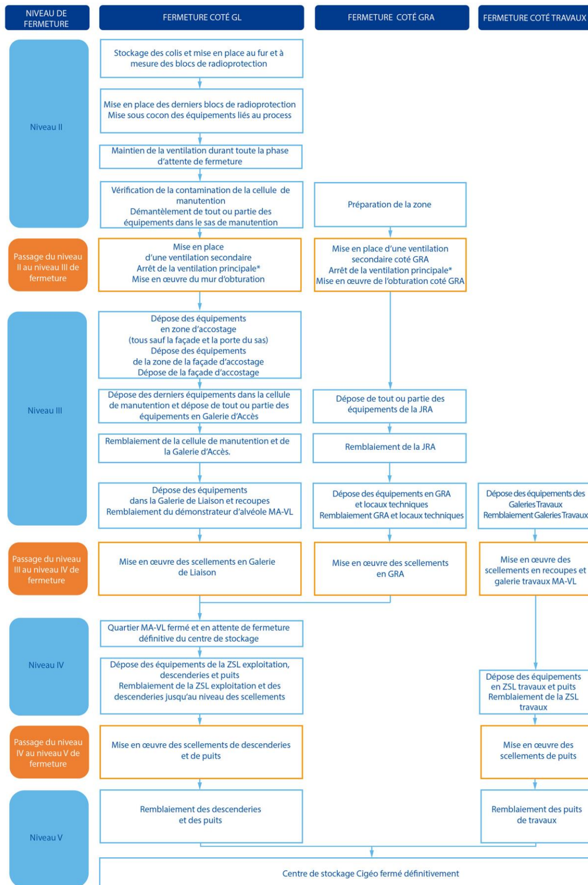
Figure 2-5 Niveaux de fermeture 2 à 5 de l'alvéole MA-VL
