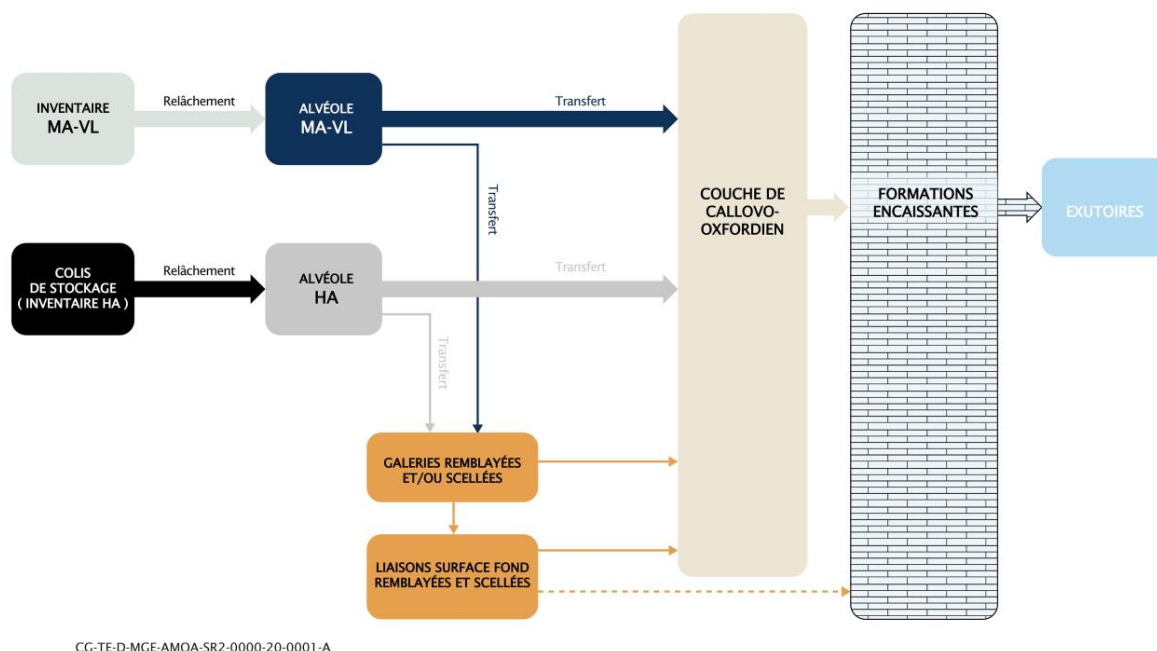
Figure 7-15 Schéma illustratif des composants et des voies de transfert pour le scénario d'évolution normale
