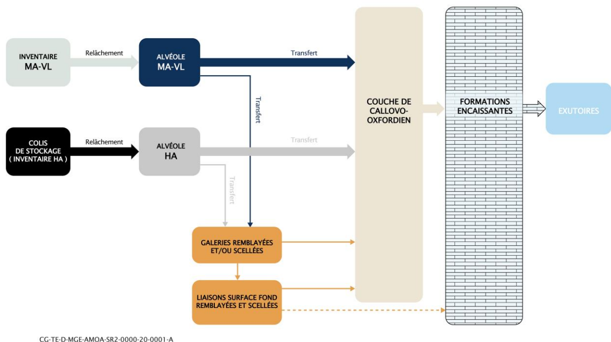
Figure 4-15 Schéma illustratif des composants et des voies de transfert potentielles pris en compte pour le scénario d'évolution normale
