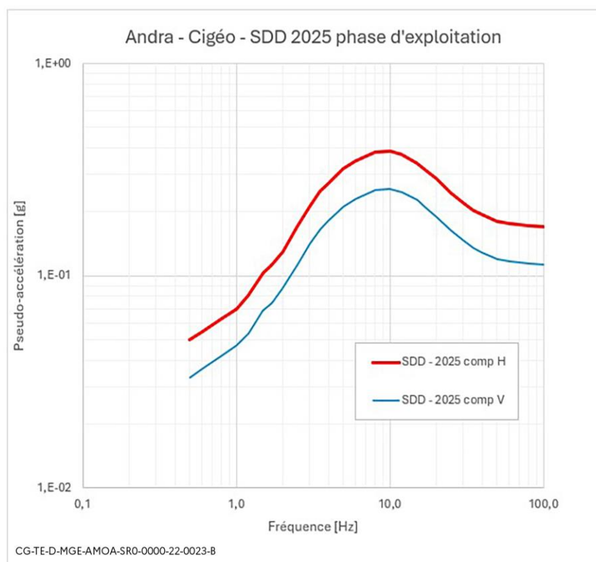
Figure 5-26 Spectre de sol du séisme de dimensionnement (SDD) - composantes horizontale et verticale
