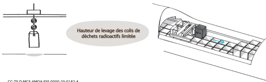
Figure 7-21 Illustration de la manutention des colis de stockage MA-VL à faible hauteur
