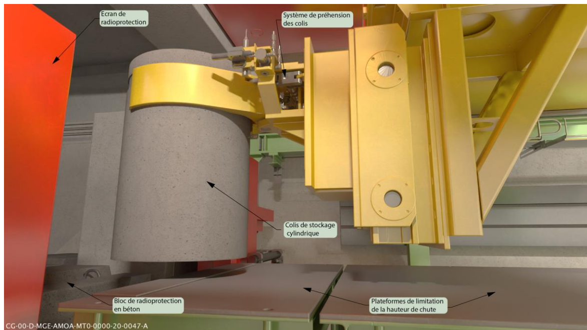
Figure 5-16 Illustration des équipements de manutention de colis de stockage MA-VL (cas de colis en stockage direct)
