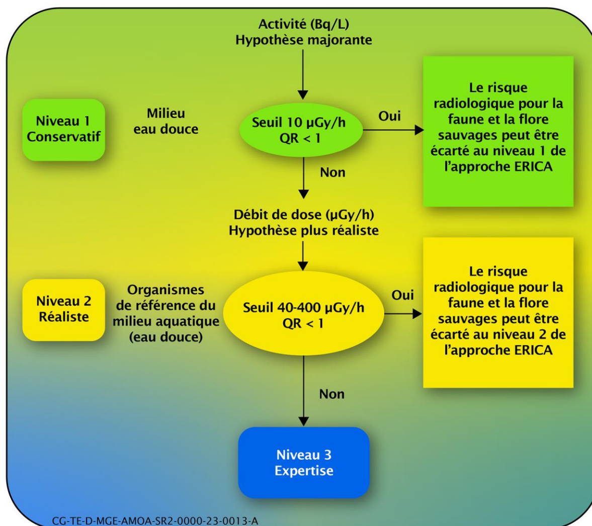
Figure 4-8 Synthèse de la démarche graduée pour définir le risque radiologique à l'environnement sur la période long terme après fermeture
