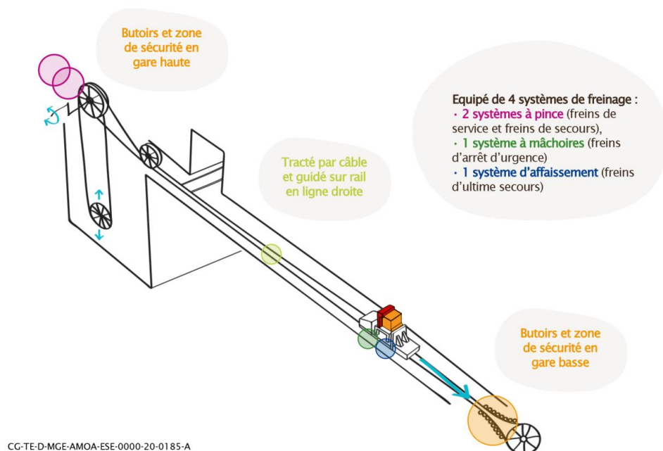
Figure 7-20 Illustration des dispositifs de sécurité du transfert incliné par funiculaire en descenderie
