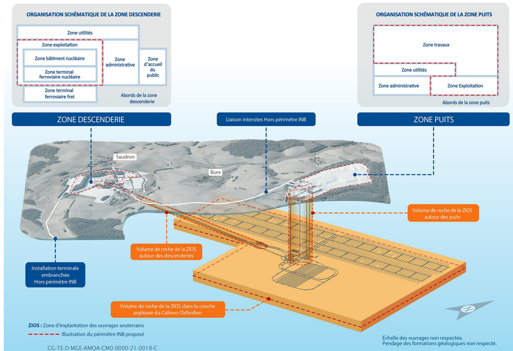
Figure 7-9 Représentation schématique du périmètre INB Cigéo
