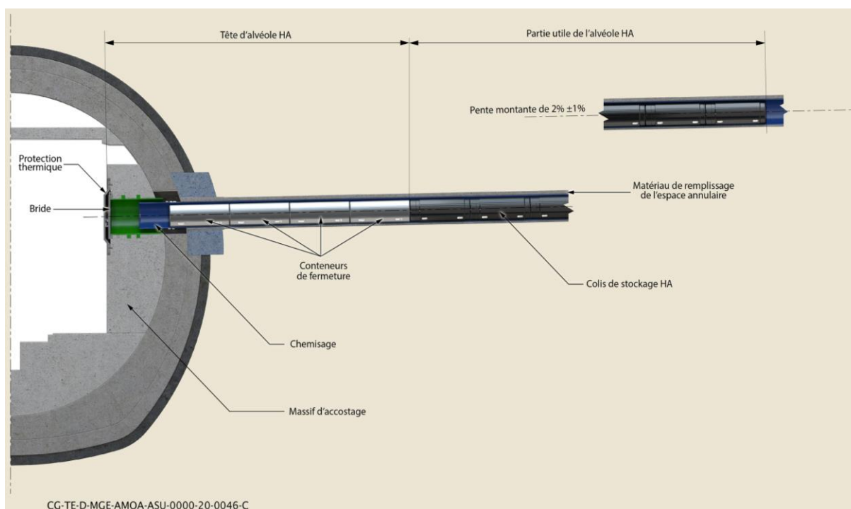
Figure 4-8 Schéma de principe d'un alvéole HA en attente de fermeture
