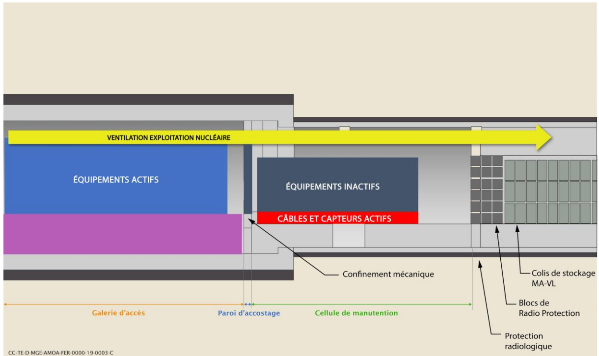
Figure 4-2 État de l'alvéole en attente de l'étape 1 de fermeture (obturation de l'alvéole) côté galerie d'accès
