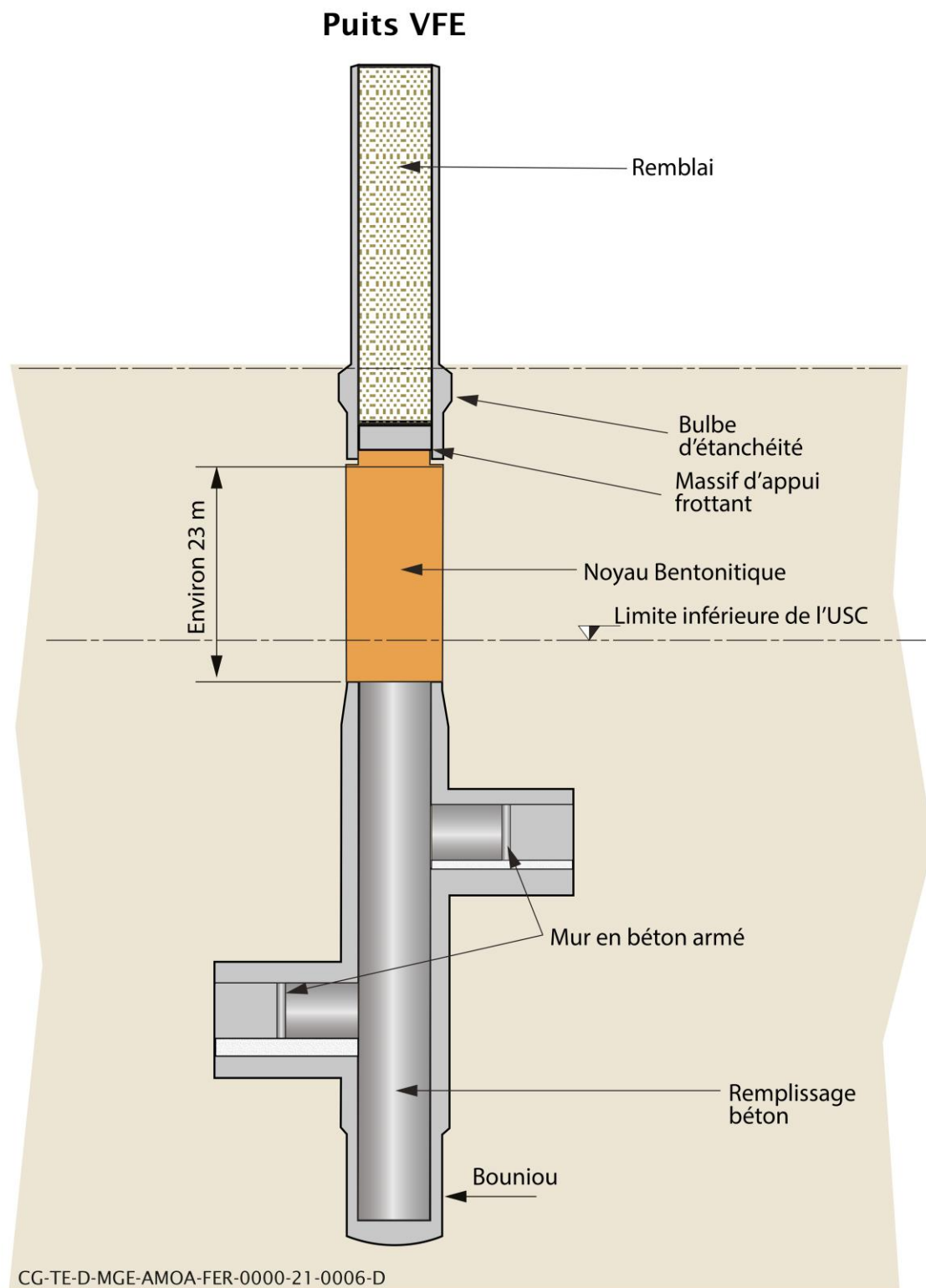
Figure 4-13 Schéma de principe d'un scellement d'un puits
