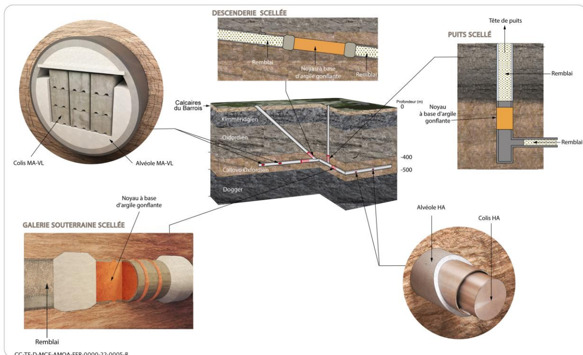
Figure 6-1 Schéma de principe de l'état final envisagé
