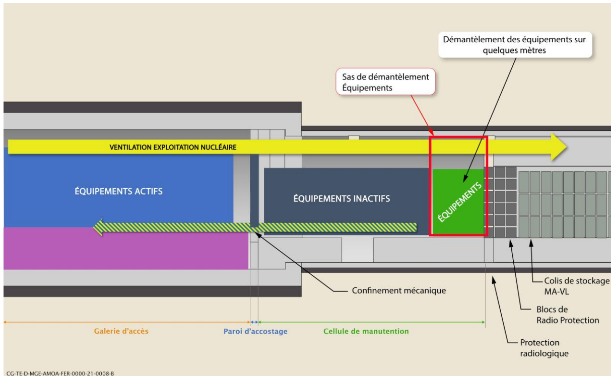
Figure 4-4 Démantèlement des équipements de la cellule de manutention sur quelques mètres devant le voile de radioprotection à l'entrée de la zone de stockage
