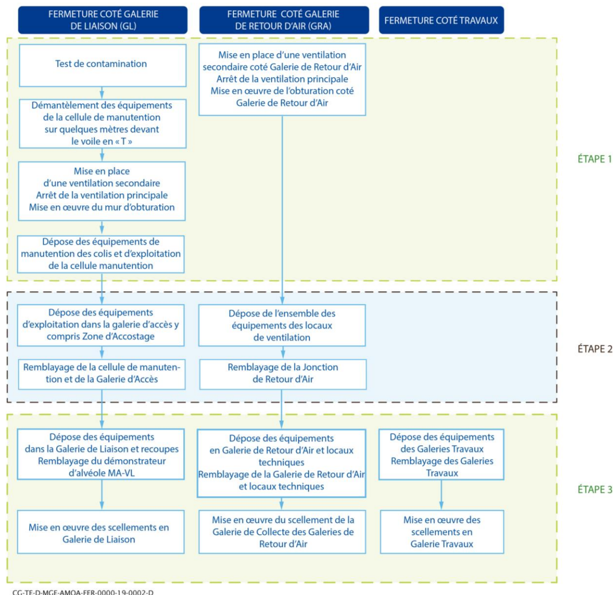
Figure 4-3 Schéma des étapes de fermeture pour le quartier de stockage MA-VL
