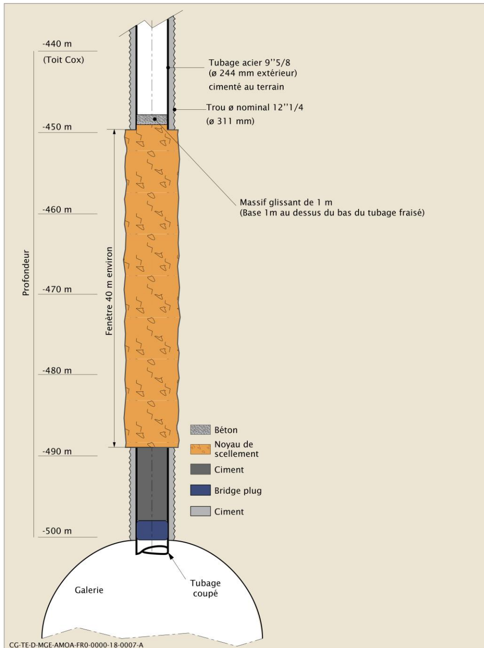
Figure 4-15 Schéma de principe de scellement de la colonne à carburant
