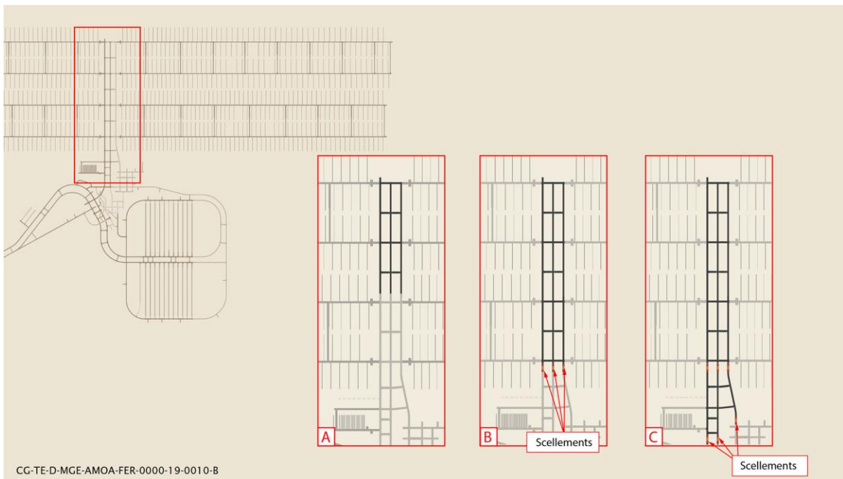
Figure 4-12 Fermeture Étape 4 - Séquençage de la fermeture de la zone de stockage HA
