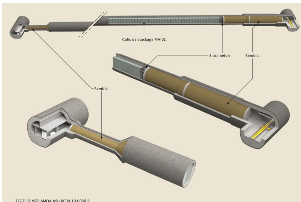
Figure 4-6 Alvéole MA-VL et galerie d'accès obturés et galeries de liaison et de retour d'air non obturées
