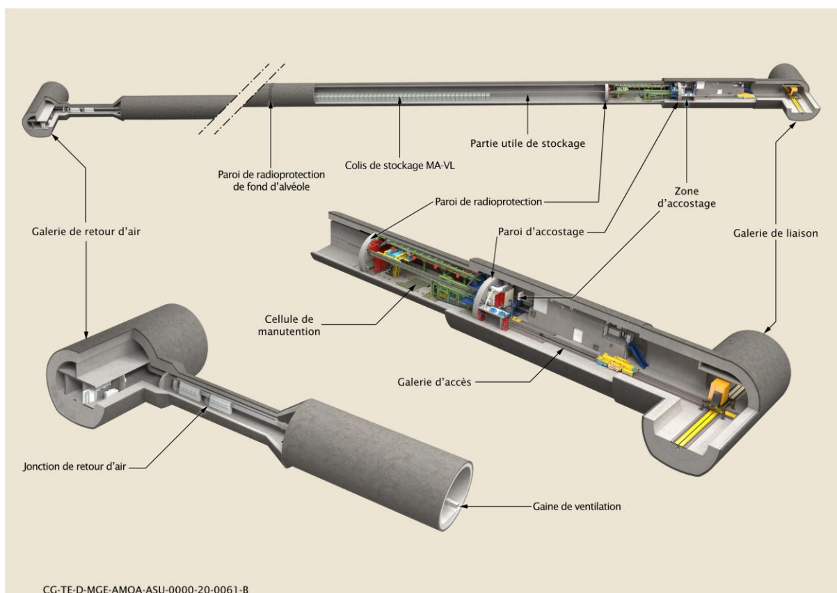
Figure 4-1 Vue globale de l'alvéole MA-VL en phase de fonctionnement
