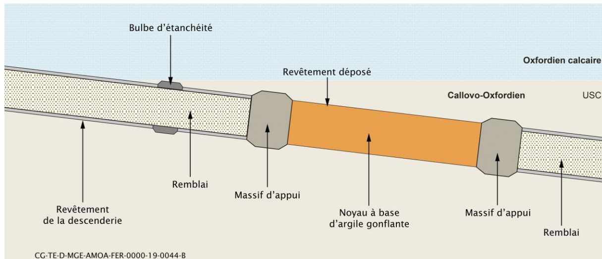
Figure 4-14 Schéma de principe de scellement en descenderie
